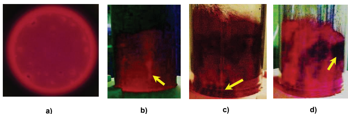
Figure 58. Photographies du lit fluidisé : a) Renardage en surface, b) Renardage en paroi, c) Couche ségrégée avec présence de renardage, d) Particules de lit collées en paroi du réacteur. Ces observations ont été réalisées pour une température opératoire de 850°C avec de l'air comme gaz de fluidisation ( H/D=0,6 , U_g \approx 2U_{mf} , m_{cendres}=0,3g ).
