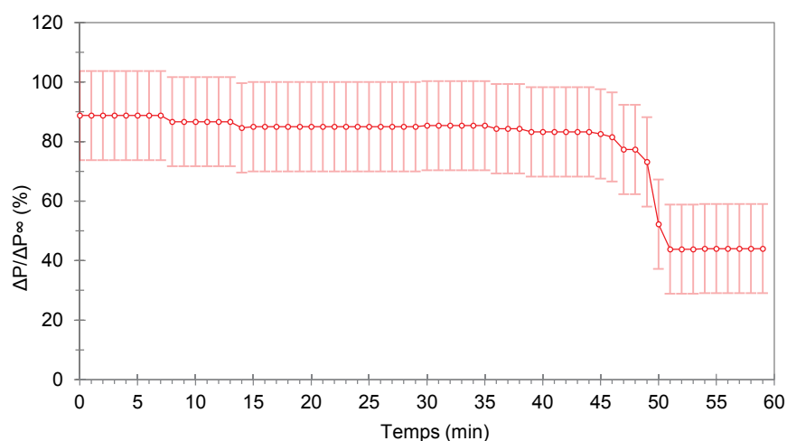
Figure 66. Evolution de la perte de charge du lit fluidisé sous atmosphère neutre à 850°C
