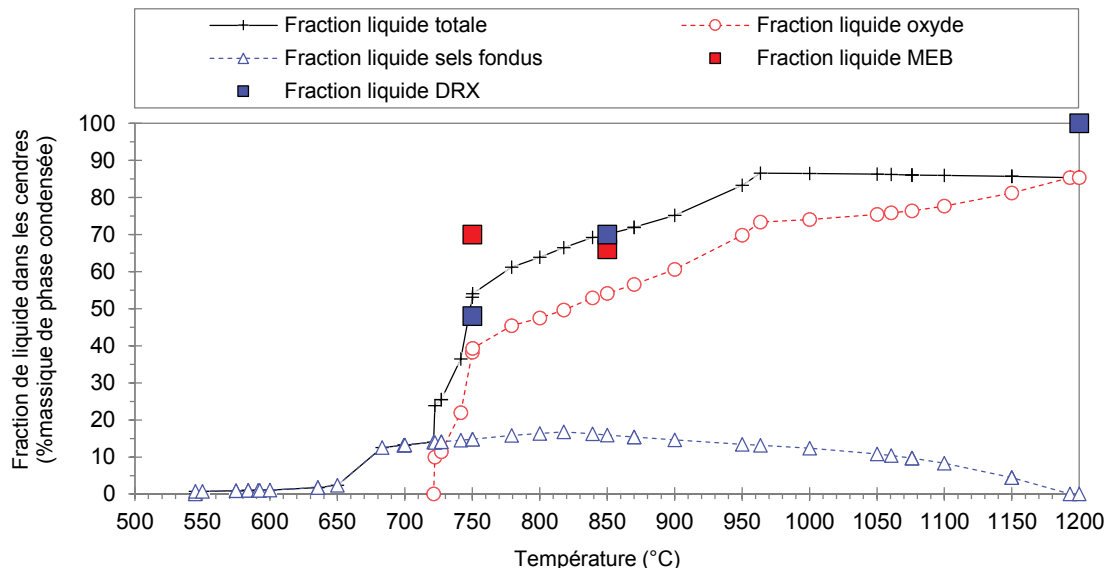
Figure 31. Evolution de la fraction de liquide calculée à l'équilibre thermodynamique (en % massique de cendres en phase condensée)
