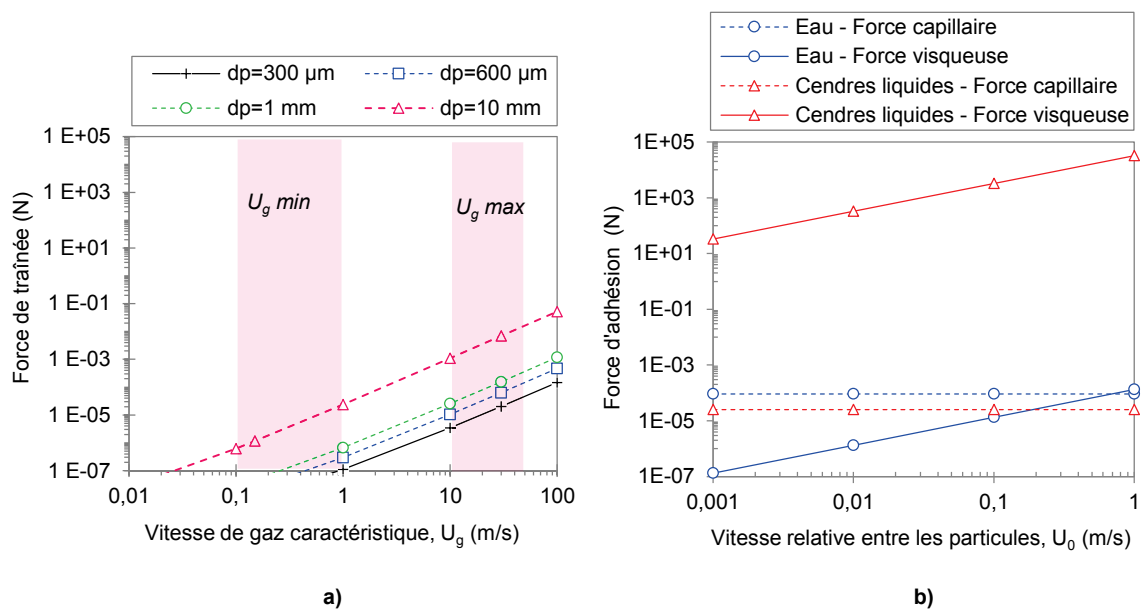
Figure 88. Comparaison des forces de rupture et d'adhésion des ponts liquides inter-particulaires : a) Evolution des forces de traînée en fonction de la vitesse caractéristique du gaz pour différents diamètres d'agglomérats, b) Evolution des forces d'adhésion des ponts liquides (capillaire, visqueuse) en fonction de la vitesse relative entre les particules de lit dans le cas d'un pont liquide constitué d'eau ou de cendres liquides.
