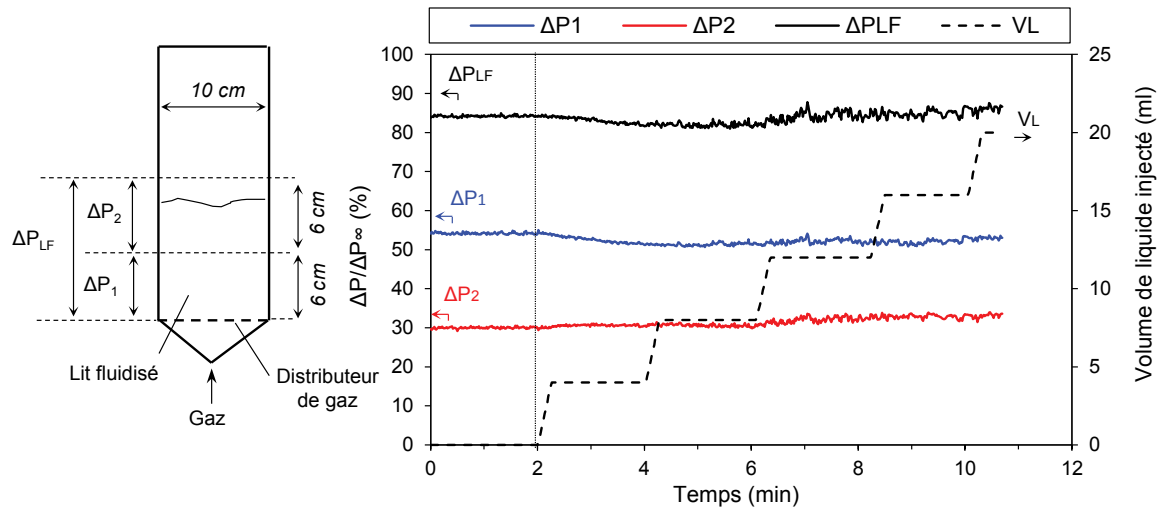
Figure 55. Evolution de la perte de charge du lit fluidisé, totale ( \Delta P_{LF} ) et par section ( \Delta P_1 , \Delta P_2 ), en fonction du volume d'eau injecté ( V_L ) dans la couche de solide au cours de l'essai (essai mauvais mouillage : H/D=1 , U_g=2U_{mf} , microbilles de verre). NB : les flèches indiquent l'axe de lecture des unités de chaque paramètre étudié.
