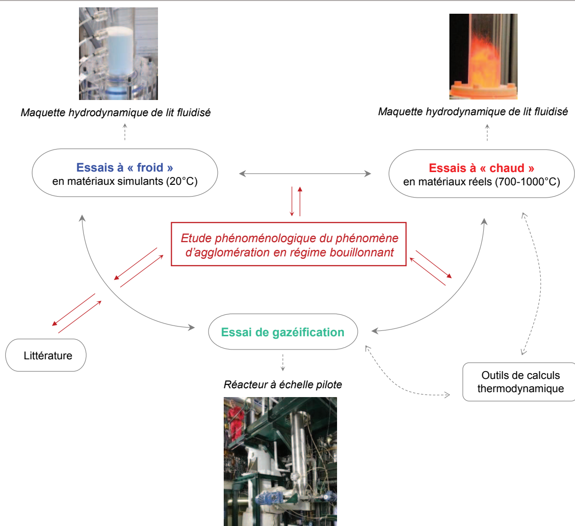
Figure 20. Schéma de l'approche expérimentale utilisée
