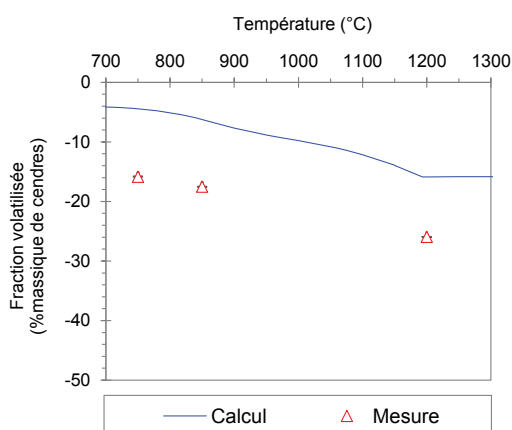
Figure 33. Evolution de la perte de masse des cendres en température : comparaison des valeurs mesurées et calculées à l'équilibre thermodynamique (en % massique de cendres)
