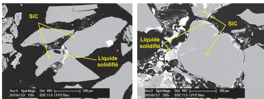
Figure 74. Coupes transversales d'agglomérats observés par MEB et provenant de l'essai de gazéification de paille de blé à échelle pilote dans un lit de SiC (observations réalisées en contraste de phase chimique).
