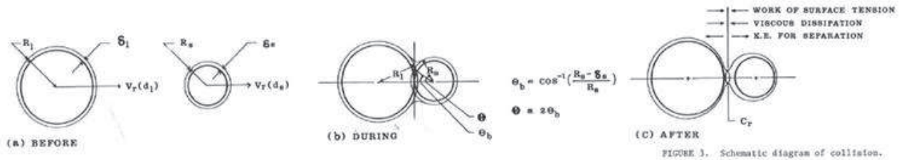
Figure 17. Représentation schématique de la collision inter-particulaire (Jen, 1980)
