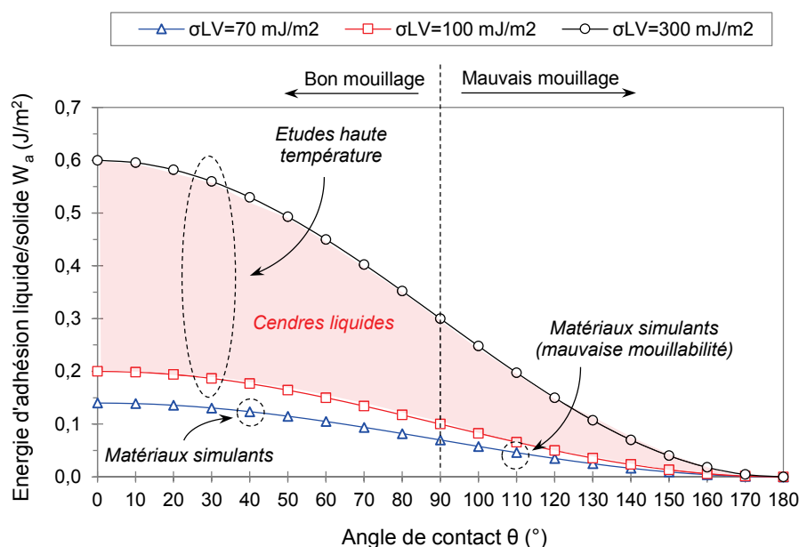
Figure 83. Evolution de l'énergie d'adhésion liquide/solide W_a en fonction de l'angle de contact \theta pour différentes valeurs de l'énergie de surface liquide/vapeur \sigma_{LV} (eau, cendres liquides). L'énergie d'adhésion est calculée à partir de la relation de Young-Dupré. Les différents systèmes étudiés expérimentalement sont également représentés.
