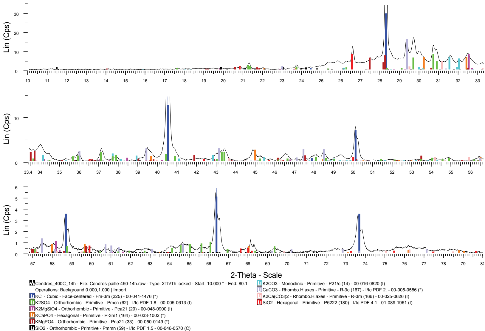
Figure 101. Diffractogramme des cendres obtenues après combustion de la paille de blé à 400°C sous air
