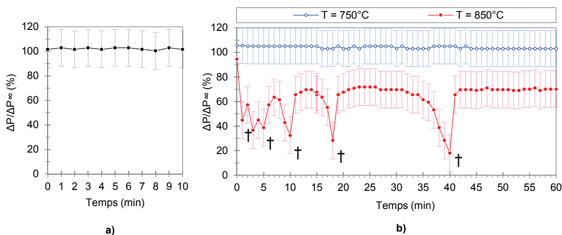
Figure 57. Evolution de la perte de charge du lit fluidisé au cours du temps : a) sans cendres à 850°C, b) avec cendres (0,4 % massique de lit) à 750°C et 850°C († : mélange manuel du lit à l'aide d'une tige métallique, cette opération est réalisée lorsque la défluidisation complète du lit est visuellement observée)
