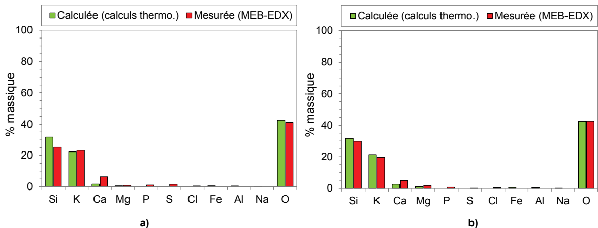
Figure 32. Comparaison des compositions du liquide oxyde calculées à l'équilibre thermodynamique et mesurées par sonde EDX (moyenne de plusieurs zones EDX) pour différentes températures de recuit : a) 750°C, b) 850°C
