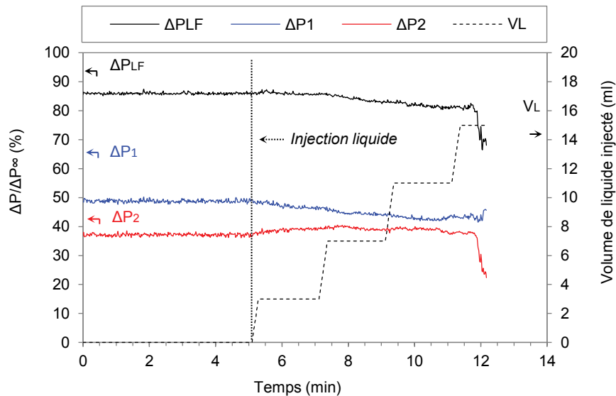
Figure 106. Essai E8 : Evolution de la perte de charge du lit fluidisé, totale ( \Delta P_{LF} ) et par section ( \Delta P_1 , \Delta P_2 ), en fonction du volume d'eau injecté ( V_L ) dans la couche de solide au cours de l'essai (essai de référence : H/D=1 , U_g=2U_{mf} , microbilles de verre). NB : les flèches indiquent l'axe de lecture des unités de chaque paramètre étudié.
