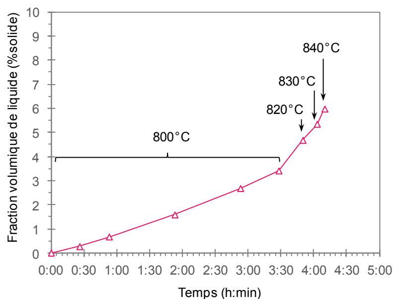
Figure 76. Estimation à l'équilibre thermodynamique de l'évolution de la fraction volumique de liquide dans le lit au cours du temps lors de l'essai de gazéification de paille de blé
