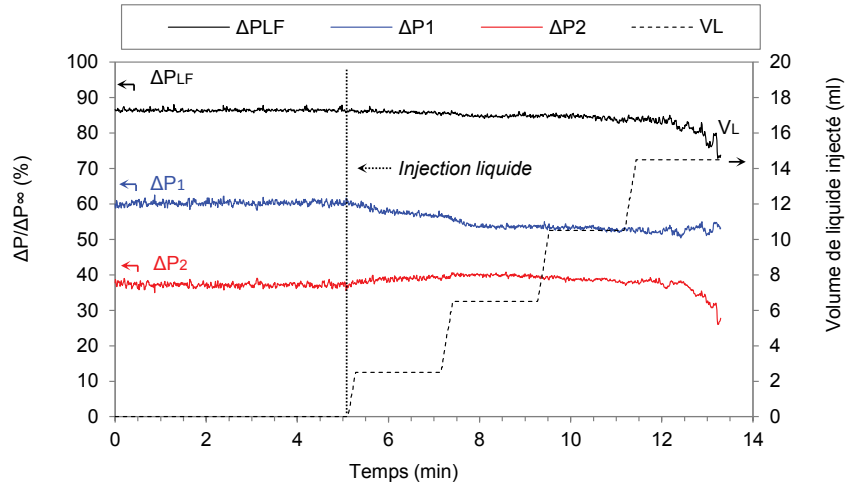
Figure 105. Essai E7 : Evolution de la perte de charge du lit fluidisé, totale ( \Delta P_{LF} ) et par section ( \Delta P_1 , \Delta P_2 ), en fonction du volume d'eau injecté ( V_L ) dans la couche de solide au cours de l'essai (essai de référence : H/D=1 , U_g=2U_{mf} , microbilles de verre). NB : les flèches indiquent l'axe de lecture des unités de chaque paramètre étudié.
