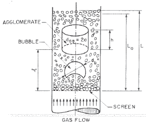
Figure 19. Illustration du cas modélisé par (Tardos, 1985)
