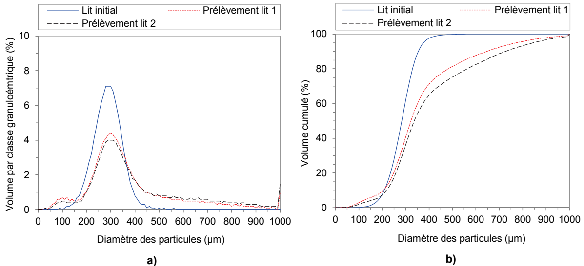
Figure 81. Comparaison de la distribution granulométrique des prélèvements de lit après l'essai de gazéification de paille de blé à échelle pilote par rapport à la granulométrie initiale du lit : a) Répartition en volume par classe granulométrique, b) Répartition en volume cumulé.
