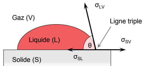
Figure 82. Mouillage d'une surface solide par une goutte de liquide
