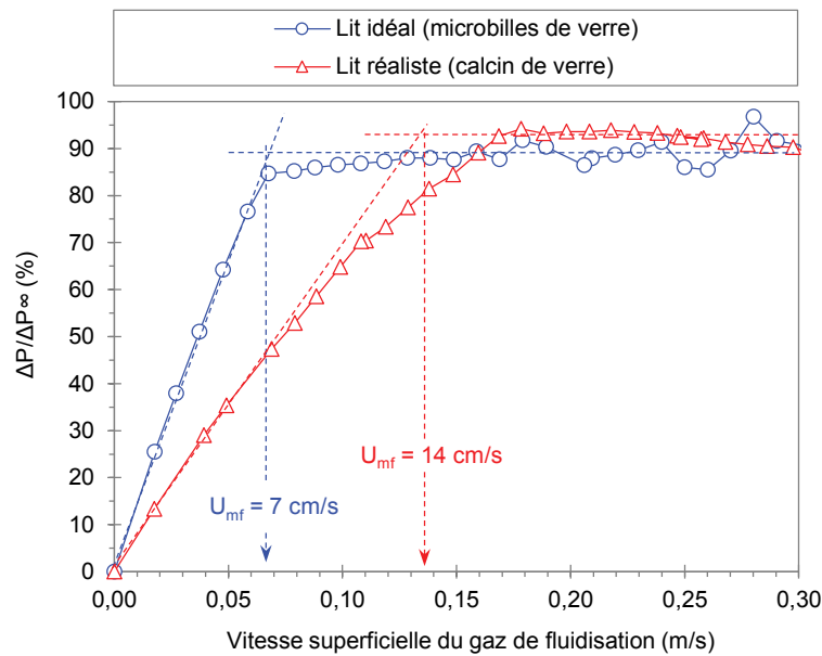
Figure 25. Détermination de la vitesse minimale de fluidisation des lits de verre (microbilles, calcin) à partir de la mesure de l'évolution de la perte de charge du lit en fonction de la vitesse superficielle du gaz de fluidisation (baisse progressive)
