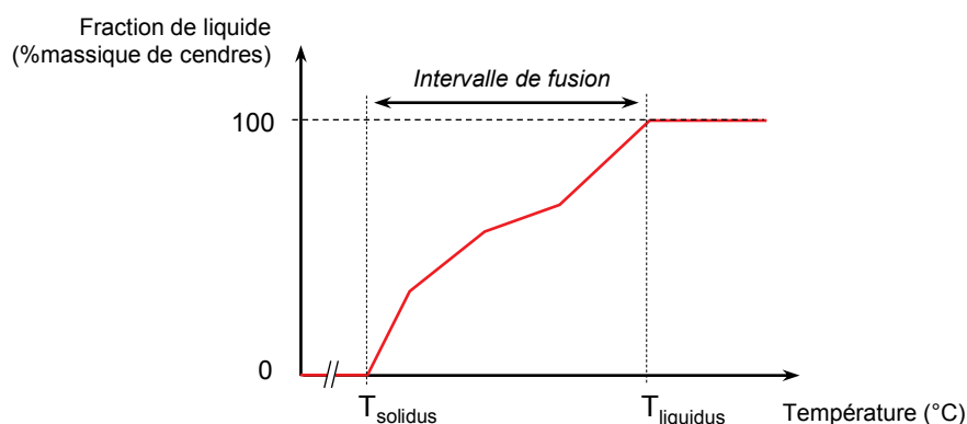
Figure 4. Exemple d'évolution de la quantité de liquide au cours de la fusion des cendres
