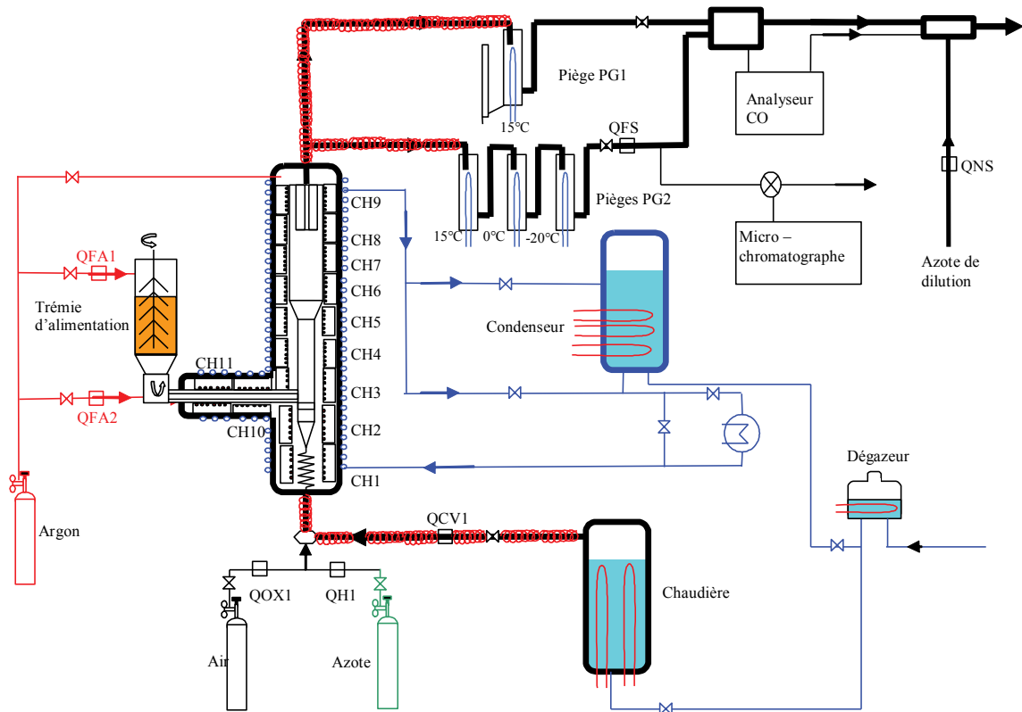
Figure 43. Schéma de l'installation LFHT
