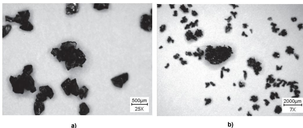
Figure 60. Photographies d'agglomérats observés à la loupe binoculaire : a) petits agglomérats de quelques particules, b) petits agglomérats de quelques particules et gros agglomérats millimétriques
