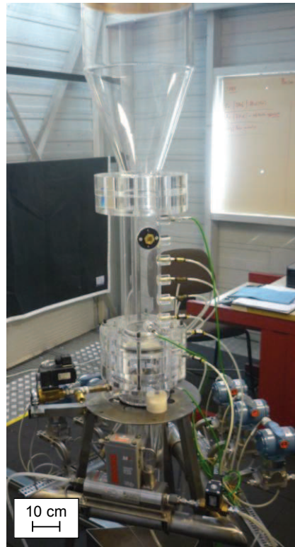
Figure 26. Photographie du dispositif LFBT
