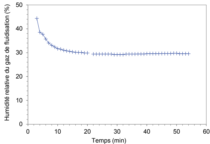
Figure 97. Evolution de l'humidité relative du gaz de fluidisation au cours du temps
