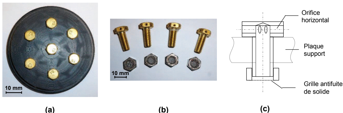
Figure 28. Distributeur de gaz à tuyères : a) photographie du distributeur (vue de dessus), b) photographie de quelques tuyères avec leur grille antifuite de solide, c) schéma des tuyères
