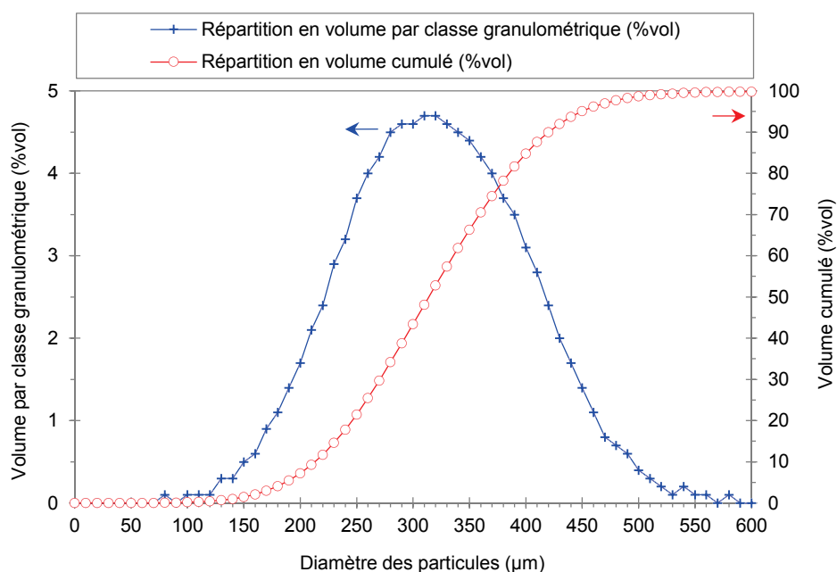
Figure 23. Distribution granulométrique du lit de calcin de verre (lit réel) utilisé lors des essais à « froid » (le diamètre des particules correspond ici au diamètre de corde)
