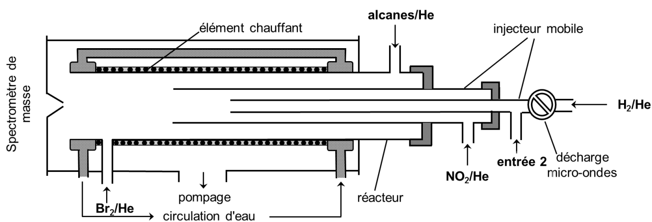
Figure III- 1 : Réacteur à écoulement haute température pour les réactions alcane + OH.
