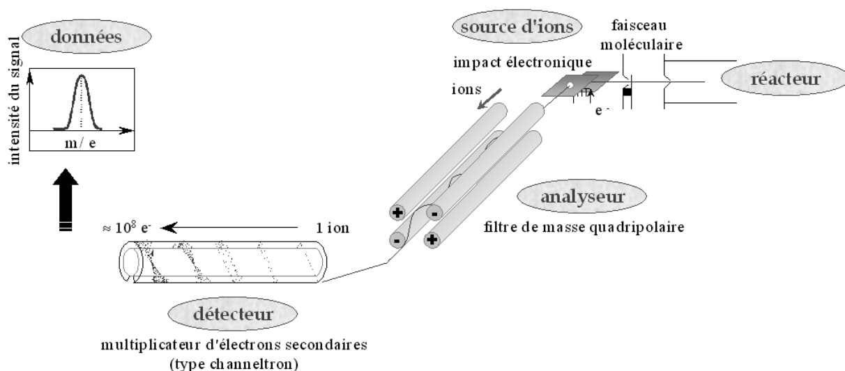
Figure II- 9 : Schéma de principe d'un spectromètre de masse avec quadripôle 36 .
