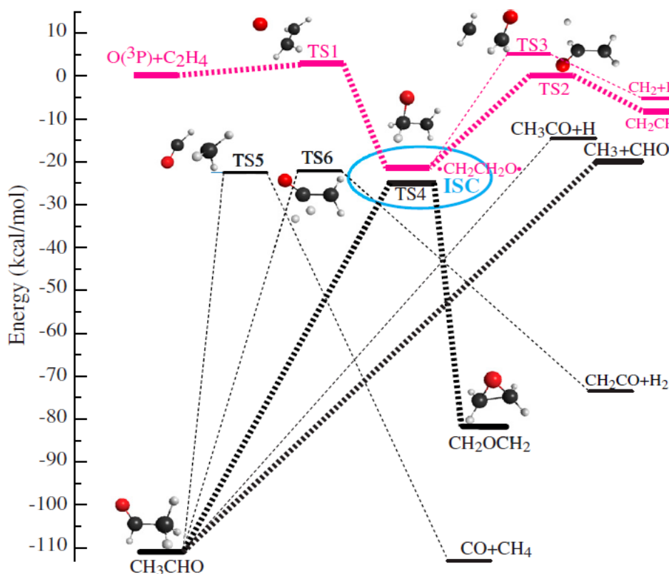
Figure V- 12 : Schéma simplifié utilisant les potentiels d'énergie de surface du triplet (rose) et du singulet (noir) pour la réaction O + C_2H_4 .
