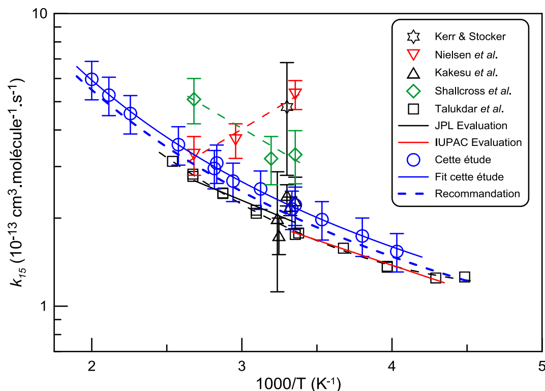
Figure IV- 9 : Ensemble des données existantes pour la réaction ETN + OH en fonction de la température. Les données proviennent de : ☆ Kerr & Stocker 64 , ▼ Nielsen et al. 65 , △ Kakesu et al. 66 , ◇ Shallcross et al. 67 , □ Talukdar et al. 68 , — JPL 69 , — IUPAC 60 .
