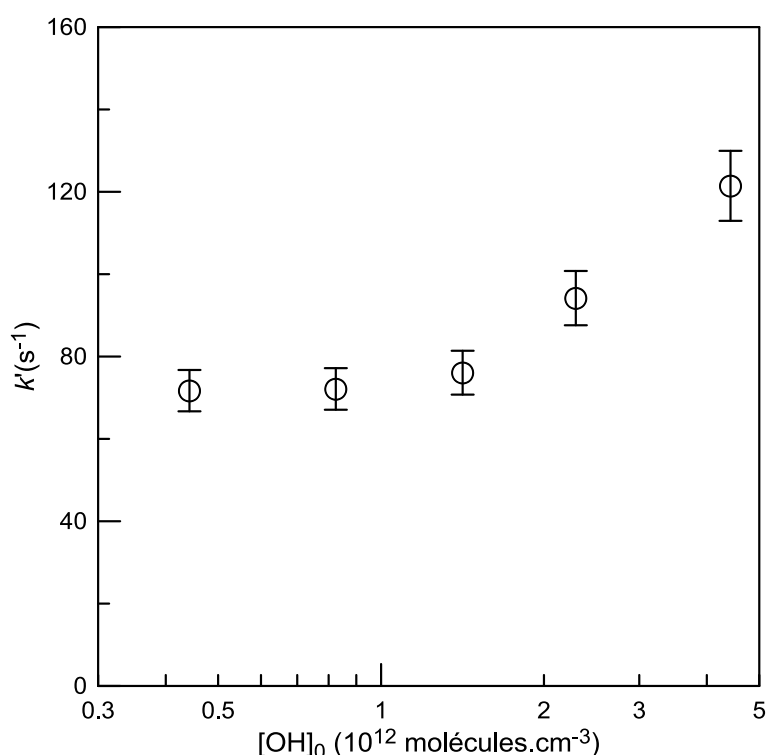
Figure IV- 11 : Constante de vitesse mesurée en fonction de [\text{OH}]_0 pour la réaction OH + PNT à 300 K.
