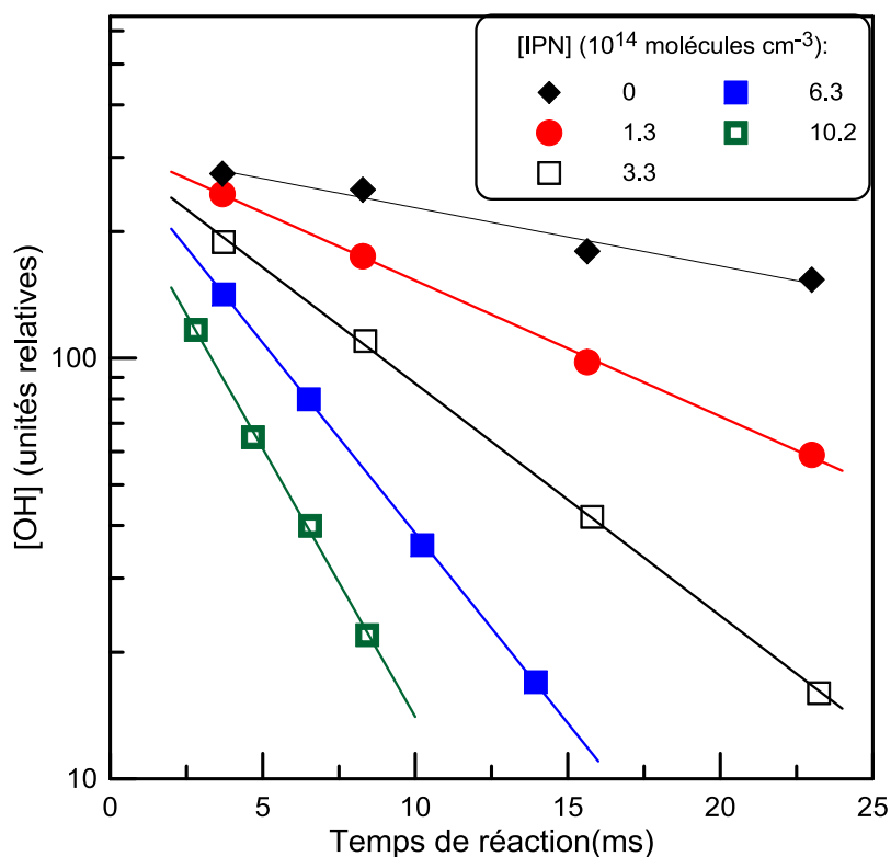
Figure IV- 3 : Exemple de cinétique de consommation de OH pour des concentrations d'IPN comprises entre 0 et 10,2 \times 10^{14} moléculas.cm -3 à 293 K et 1 Torr, source OH (H+NO 2 ).
