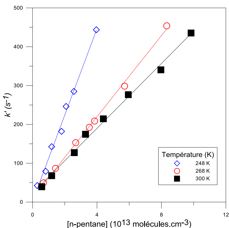
Figure III- 7 : Réaction \text{OH} + \text{C}_5\text{H}_{12} : Constante de vitesse apparente pour trois températures différentes 248, 268 et 300 K et une pression de 1 Torr.
