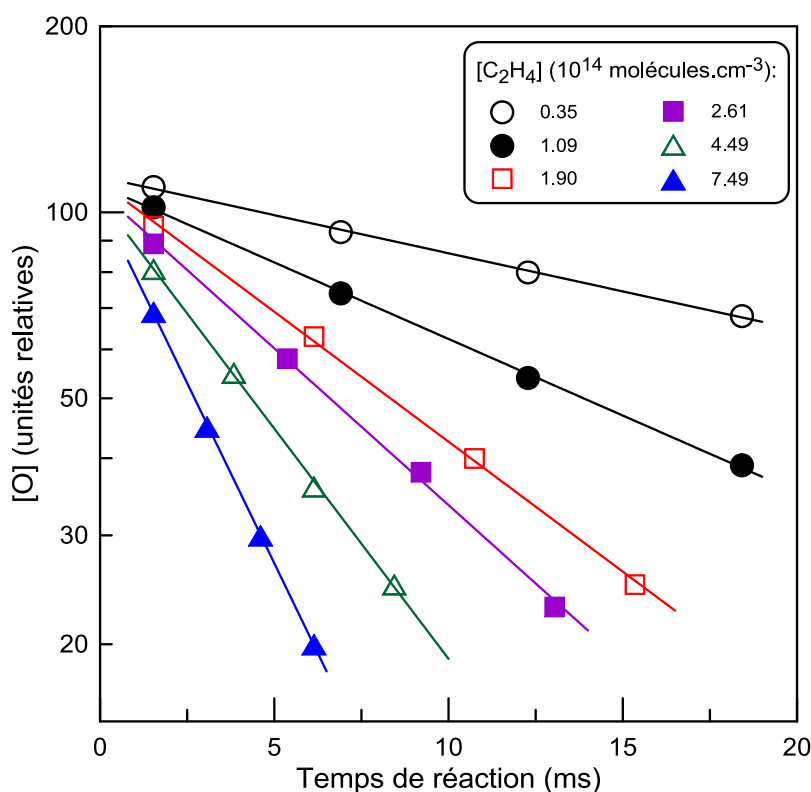
Figure V- 4 : Exemple de cinétique de consommation de O en excès d'éthylène à 230 K et 1 Torr.
