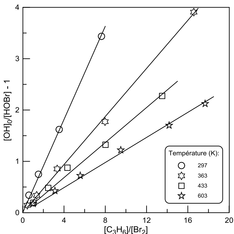
Figure V- 19 : Détermination du rapport k_{37}/k_5 pour différents ratios [\text{C}_3\text{H}_6]/[\text{Br}_2] à 297, 363, 433 et 603 K et une pression de 2 Torr.
