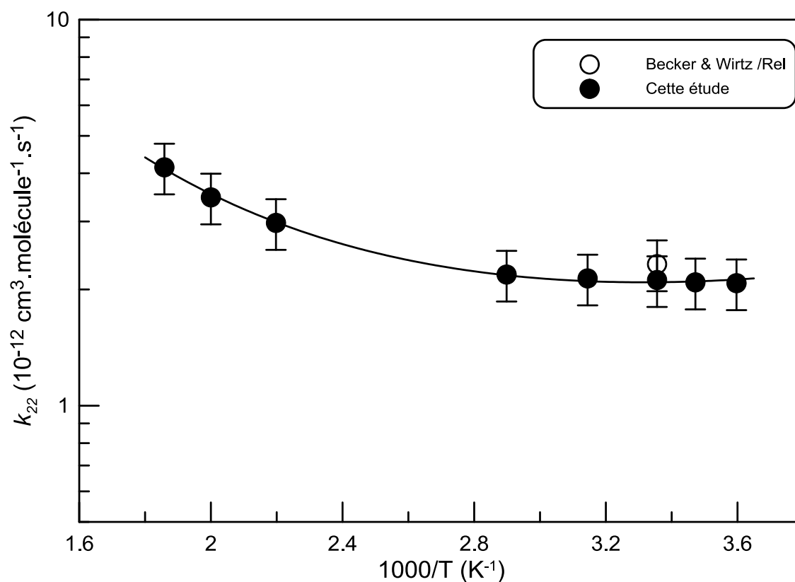
Figure IV- 22 : Ensemble des mesures pour la constante de vitesse du 2-MBNT + OH. Les données proviennent de : ○ Becker & Wirtz 58 .
