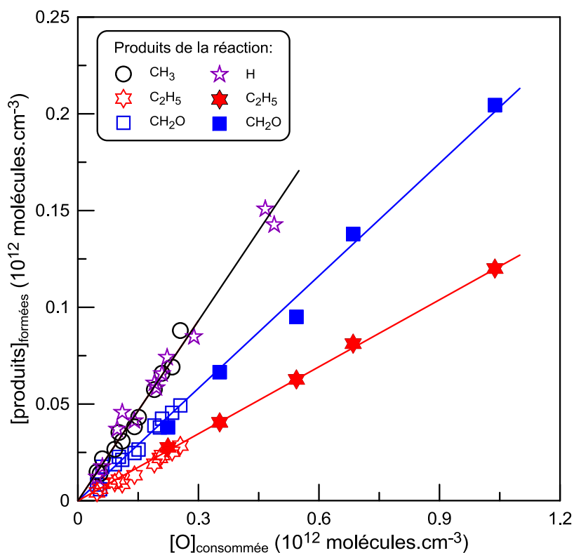
Figure V- 23 : Réaction \text{O} + \text{C}_3\text{H}_6 : concentration des produits formés \text{H} (violet), \text{CH}_2\text{O} (bleu), \text{C}_2\text{H}_5 (rouge) et \text{CH}_3 (noir) en fonction de \text{O} consommé à 905 K pour une pression de 2 Torr. Les symboles pleins correspondent aux résultats avec \text{Br}_2 à la fin du réacteur.
