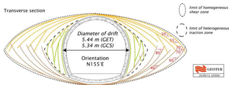
Fig. 1-2: EDZ in GCS (Galerie de conception souple), Bure URL, France (Armand et al., 2014)
