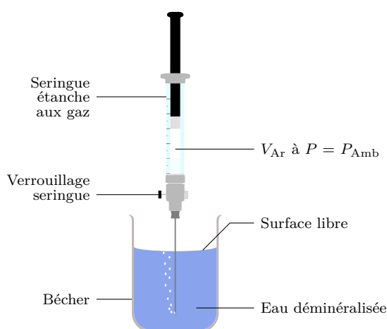
FIGURE E.2 – Détente dans un bécher d'un volume d'Ar contenu en surpression dans une seringue étanche aux gaz de sorte que la pression interne à celle-ci s'égale avec P_{\text{Amb}} . Le système de verrouillage permet l'étanchéité aux gaz de la seringue.
