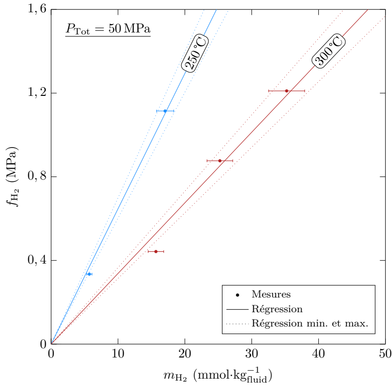
FIGURE 5.4 – Mesures expérimentales des couples f_{\text{H}_2} et m_{\text{H}_2} à P_{\text{Tot}} = 50 \text{ MPa} et à 250 et 300°C. Les paramètres des régressions linéaires sont donnée dans le Tableau 5.6.
