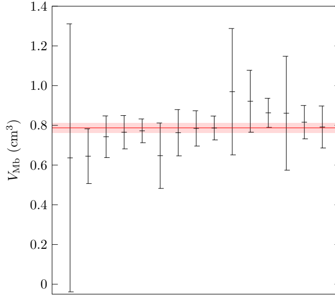
FIGURE F.7 – Les 15 mesures de V_{Mb} et erreurs associées obtenues à partir des 6 détenteurs réalisées. La ligne en rouge correspond au volume moyen pondéré, la zone en rouge clair à l'erreur associée.
