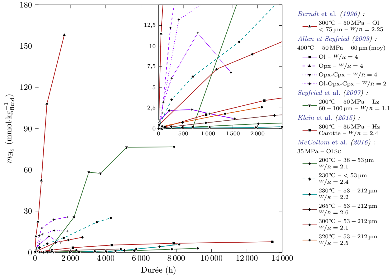
FIGURE 1.11 – Variation des m_{H_2, aq} au cours du temps dans les précédentes études expérimentales de serpentinisation du Tableau 1.1. Les expériences présentant des m_{H_2, aq} finales < 1 mmol.kg -1 ainsi que les expériences de McCollom et al. (2016), dont le seul paramètre distinctif est une durée plus courte, ne sont pas représentés. L'insert détaille l'évolution lors des 2500 premières heures.
