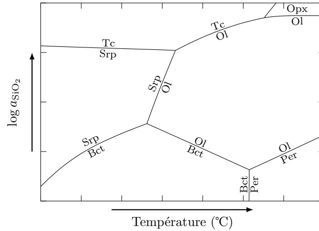
FIGURE 1.8 – Diagramme T - a_{\text{SiO}_2} montrant les domaines de stabilité des phases minérales impliquées dans la serpentinisation (modifié d'après Frost et Beard, 2007 ). Abréviations : Ol : olivine ; Opx : orthopyroxène ; Srp : serpentine ; Bct : brucite ; Tc : talc ; Per : périclase.
