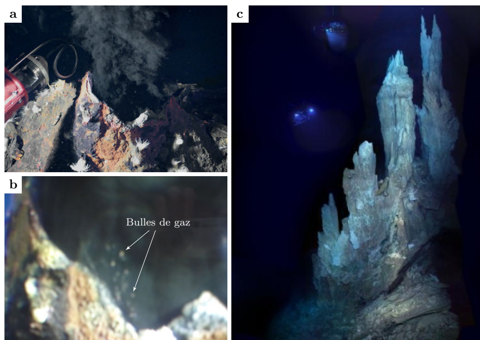
FIGURE 1.3 – Fumeurs observés sur substratum ultramafique. (a) et (b) Fumeurs noirs observés sur le site hydrothermal d'Ashadze ; les bulles de gaz (b) sont une particularité de ce site ( Charlou et al. , 2010 ). (c) Événements hydrothermaux observés sur le site hydrothermal de Lost City (photo de D. Kelley, U. of Washington).
