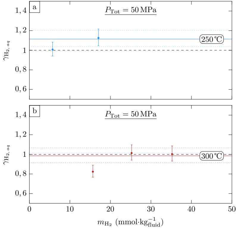
FIGURE 5.6 – \gamma_{\text{H}_2, aq} vs. m_{\text{H}_2} dans le système H 2 O-H 2 . a) à P_{\text{Tot}} = 50 MPa et à 250°C. b) à P_{\text{Tot}} = 50 MPa et à 300°C. Les valeurs discrètes sont calculées à partir de chacun des couples (f_{\text{H}_2}, m_{\text{H}_2}) . Les valeurs issues des régressions affines de f_{\text{H}_2} vs. m_{\text{H}_2} (Tableau 5.6) et indépendantes de m_{\text{H}_2} sont représentées par les droites pleines et leur domaine d'erreur borné par les droites en pointillés. Les lignes en tirets représentent les valeurs de \gamma_{\text{H}_2, aq} obtenues, pour les mêmes conditions, avec la méthode d'approximation du « CO 2 » (Paragraphe 5.5).
