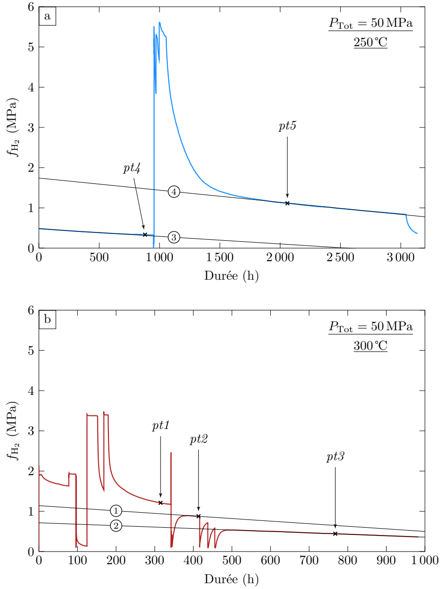
FIGURE B.1 – Régressions linéaires effectuées dans les domaines de diminution de la f_{H_2} imputable à la diffusion de l'H 2 dans les parois de l'autoclave. a) à P_{Tot} = 50 MPa et à 250°C. b) à P_{Tot} = 50 MPa et à 300°C. Les coefficients directeurs permettant de déterminer les taux de diminution de la f_{H_2} sont donnés dans le Tableau B.1.
