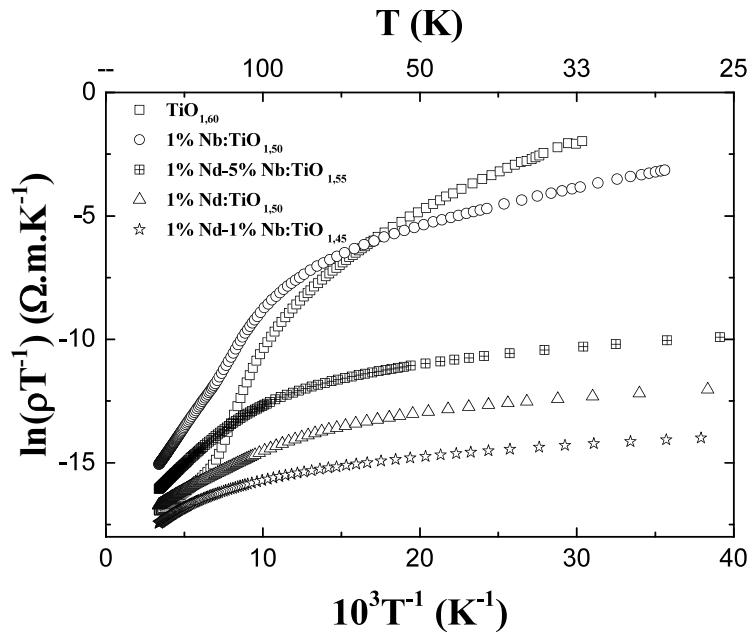
FIGURE 3.16 – Résistivité en fonction de la température des couches minces de TiO_x ( 1,45 \leq x \leq 1,60 ) dopées 1%Nd, 1%Nb, 1%Nd-1%Nb, 1%Nd-5%Nb et 3,5%Nd-1,5%Nb, obtenues à 700°C.
