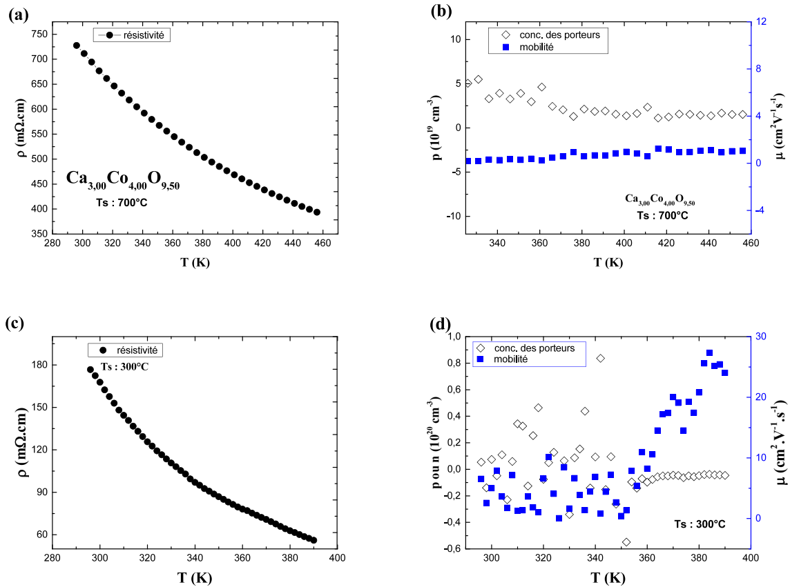
FIGURE 4.10 – Propriétés électriques des couches minces de CCO déposées à 10^{-2} mbar sur substrat \text{SiO}_2/\text{Si} à 700^\circ\text{C} (a),(b) et 300^\circ\text{C} (c),(d)
