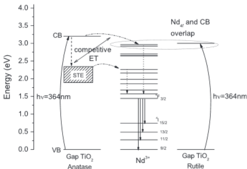
FIGURE 1.8 – Schéma représentatif des transitions électroniques entre les niveaux néodyme qui met en évidence la position des niveaux Nd par rapport à ceux des phases anatase, rutile et sur lequel est également représenté les transferts non radiatifs (flèche en tiret) et radiatifs ( flèche en trait plein) qui régissent la photoluminescence [59, 37].
