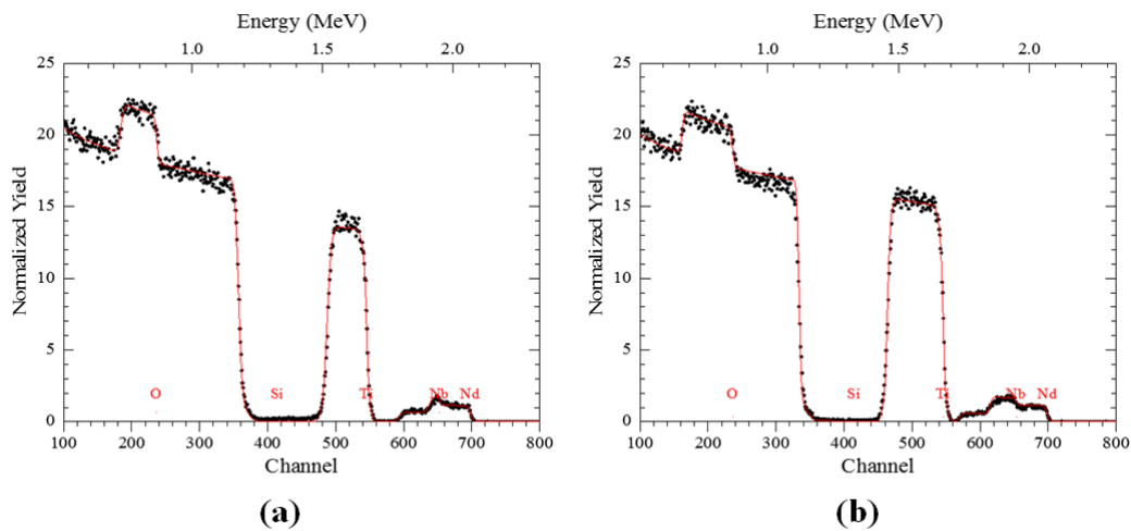
FIGURE 3.1 — Spectres RBS de la couche mince de TiO_x dopée 1%Nd et 1%Nb obtenues à 700°C de température de substrat pour (a) 10^{-1} mbar et (b) 10^{-6} mbar de pression partielle d'oxygène
