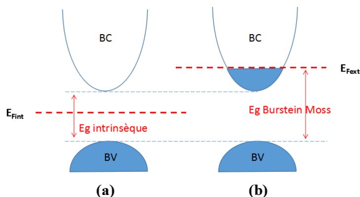
FIGURE 1.2 – Localisation du niveau de Fermi dans un semi-conducteur intrinsèque (a), un semi-conducteur extrinsèque (possédant une concentration élevée en dopants de type n) et corrélation avec l'effet Burstein Moss. E_g : Bande intrinsèque, E_{Fint} : niveau de Fermi intrinsèque, E_{Fext} : niveau de Fermi extrinsèque, BC : Bande de conduction, BV : Bande de valence.
