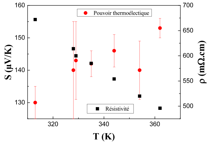
FIGURE 2.15 – Exemple de résultats obtenues grâce au ZT meter pour une couche d'oxyde de cobalt et de calcium déposée à 10^{-2} mbar et à 700^\circ\text{C}
