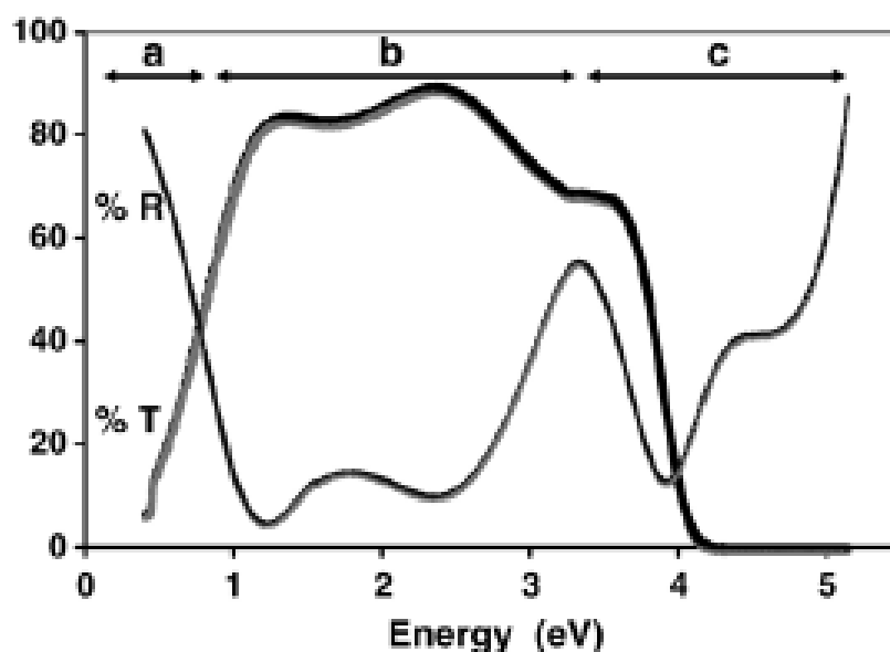
FIGURE 1.3 – Schéma représentatif de la transmission et de la réflexion d'une couche mince d'oxyde de fluor dopée par l'étain sur lequel sont définis 3 principaux domaines : celui de d'absorption quasitotale des porteurs de charge libre (a), le domaine de transmission élevée (b) et la région de forte absorption due à la transition inter-bande (c) [24].
