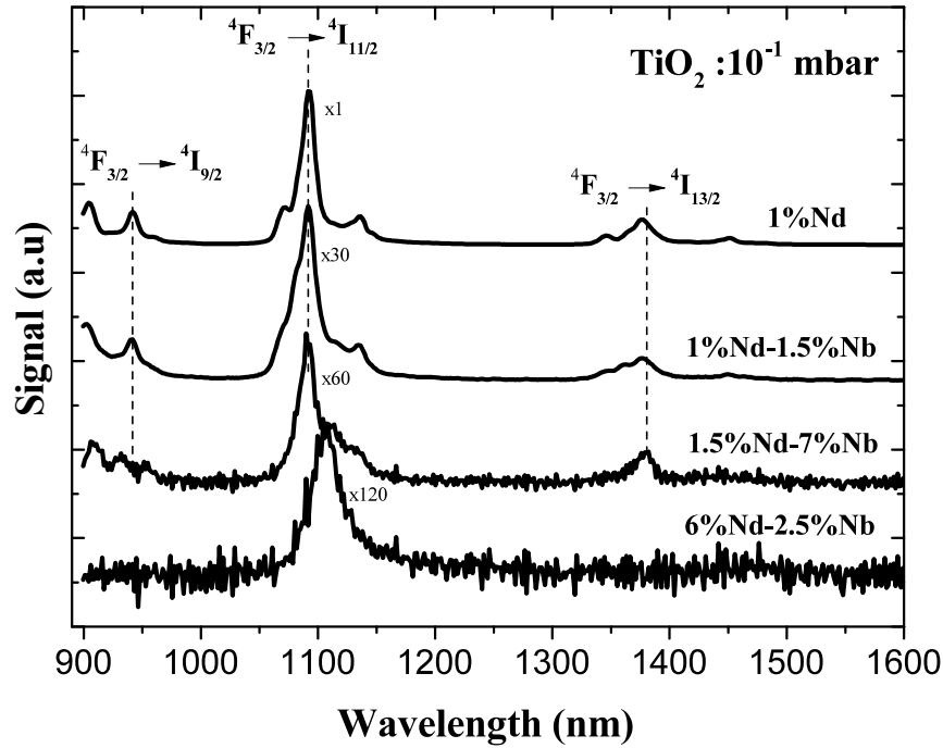
FIGURE 3.11 – Spectres de photoluminescence des couches minces de \text{TiO}_x ( 1,95 \leq x \leq 2,00 ) dopées 1%Nd, 1%Nb, 1%Nd-1,5%Nb, 1,5%Nd-7%Nb et 6%Nd-2,5%Nb, obtenues à 700°C.
