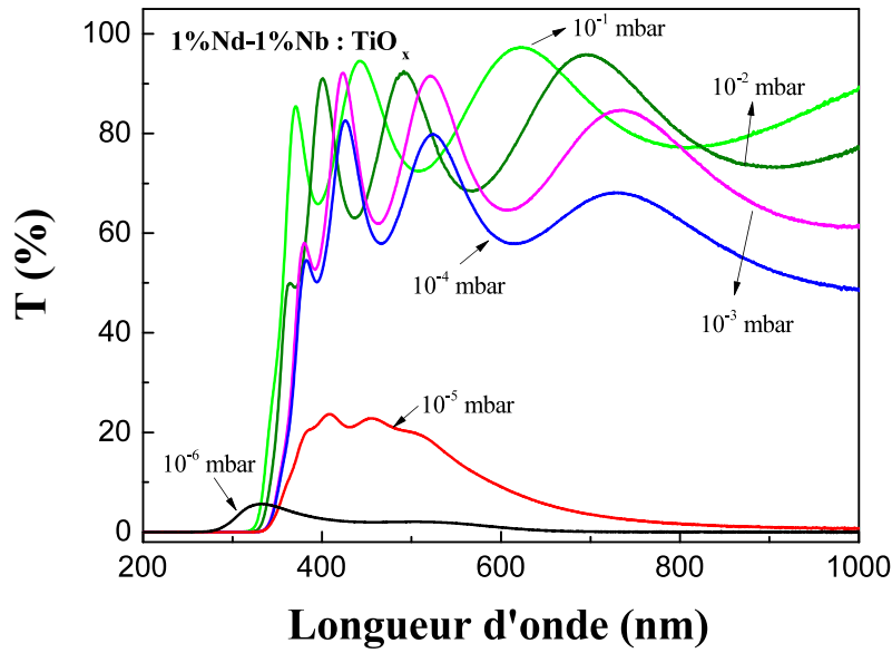
FIGURE 3.9 – Évolution en fonction de la pression partielle d'oxygène des spectres de transmission des couches minces de \text{TiO}_x ( 1,75 \leq x \leq 2,00 ) dopées 1%Nd - 1%Nb obtenues à 700°C de température de substrat.
