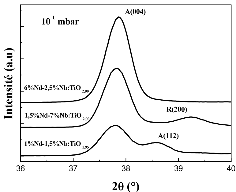
FIGURE 3.2 – Diagramme de DRX des couches minces de TiO_x dopées 1%Nd-1,5%Nb ; 1,5%Nd-7%Nb et 6%Nd-2,5%Nb ; obtenues à 700°C pour 10^{-1} mbar de pression partielle d'oxygène
