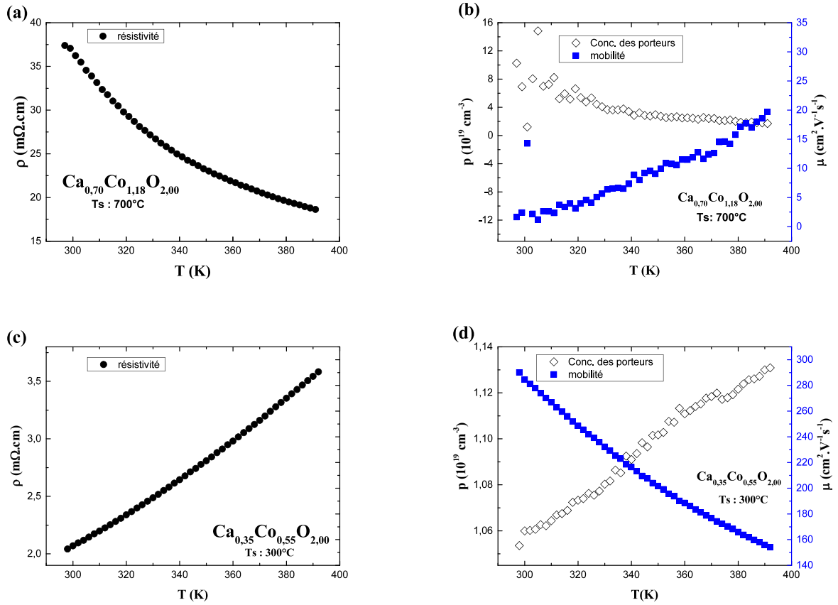
FIGURE 4.9 – Propriétés électriques des couches minces CCO déposées à 10^{-1} mbar sur SiO_2/Si à 700^\circ C (a),(b) et 300^\circ C (c),(d)
