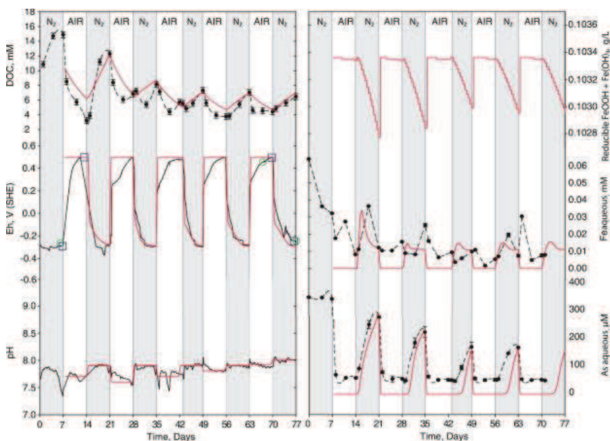
Figure 1.6 : Impact de l'alternance de cycles redox sur différents paramètres chimiques (en noir : mesuré ; en rouge : modélisé). (d'après Parsons et al. , 2013)
