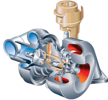
Fig. 4.3.: Turbocharger
