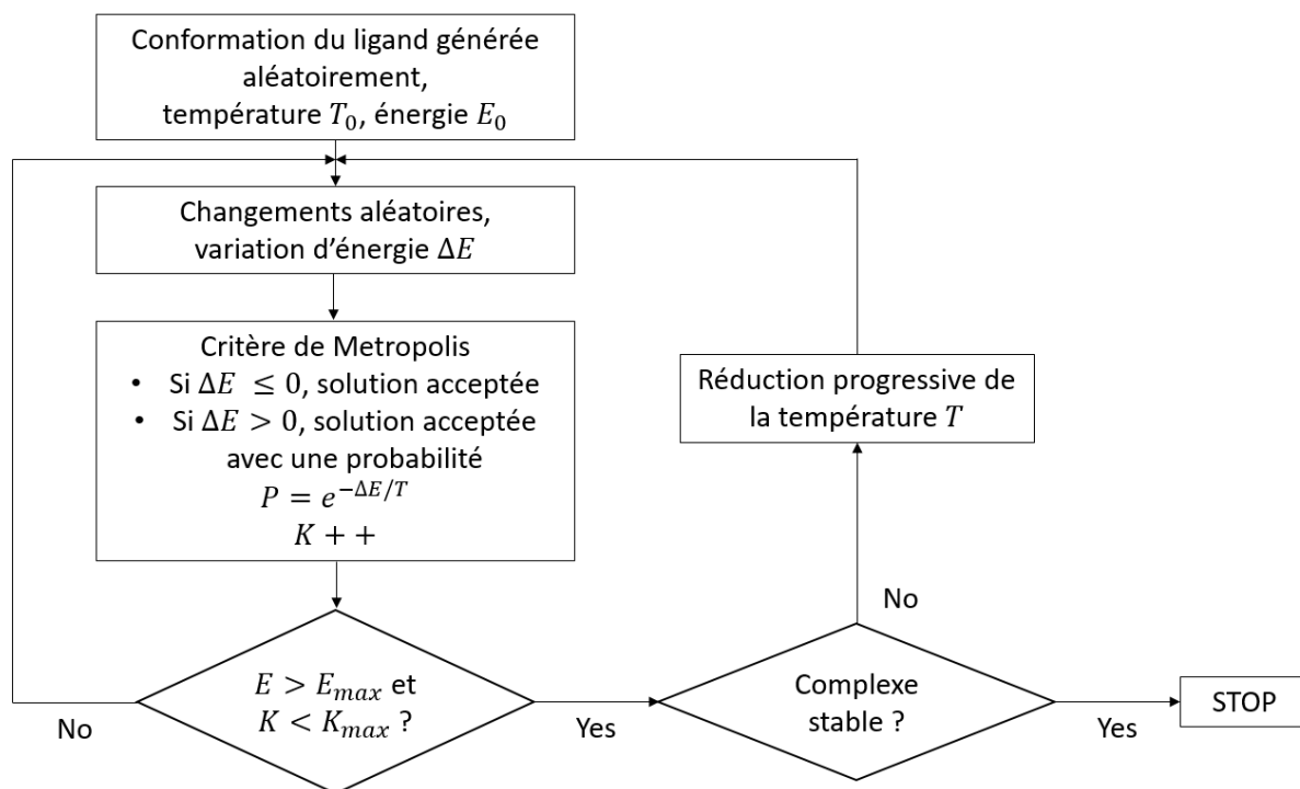
Figure 57 : Algorithme de recuit simulé
