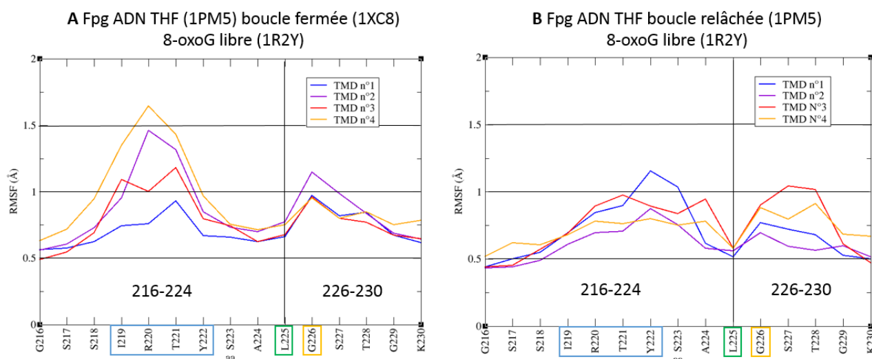
Figure 87 : RMSF des Cα de la boucle LCL des TMD -1 s
