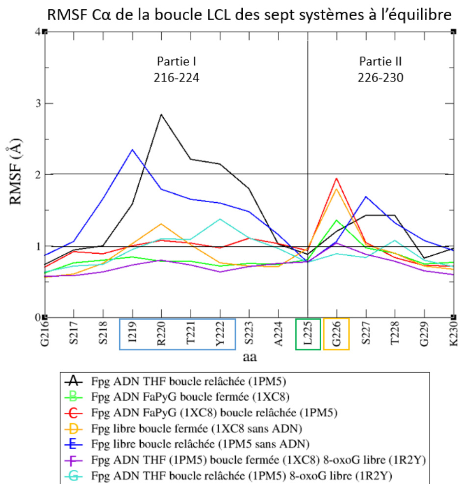
Figure 67 : RMSF de la boucle LCL
