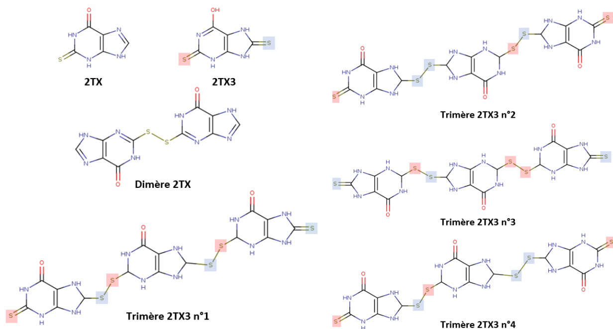
Figure 113 : Structures des monomères et des polymères de 2TX et 2TX3 utilisées pour le docking sans a priori sur les 30 structures de L/Fpg et hNEIL1
