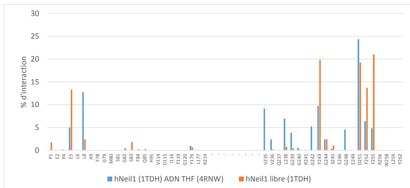
Figure 110 : Aa composant le site actif des modèles étudiés
