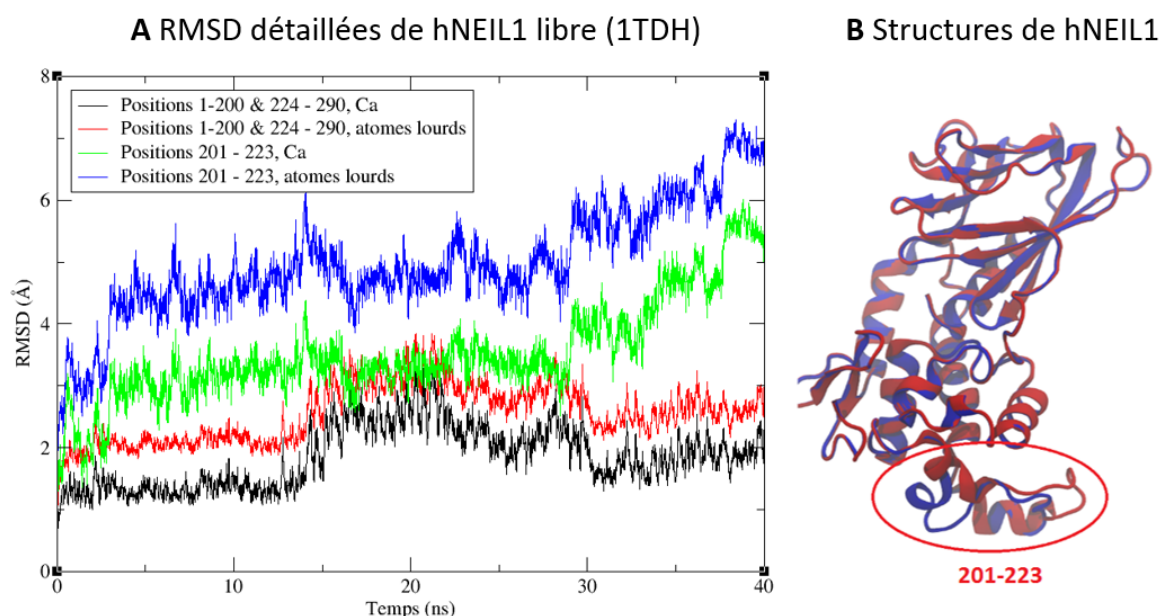
Figure 91 : Détails de la RMSD du système hNEIL1 libre (1TDH)
