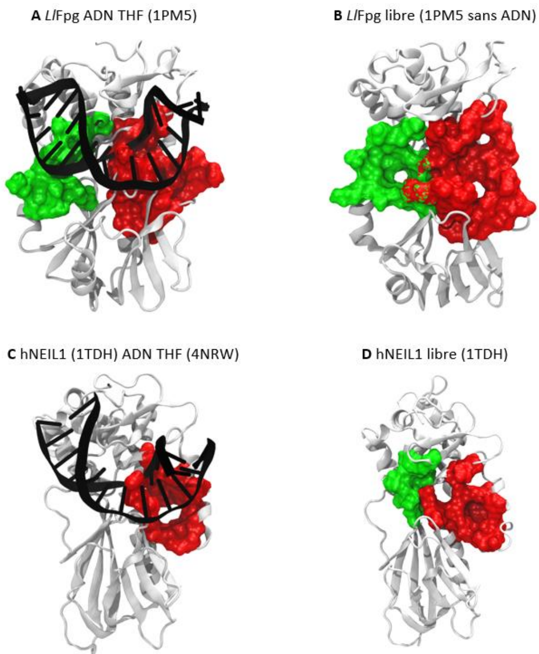
Figure 103 : Sites de fixation prédits par le test n°3 du docking sans a priori
