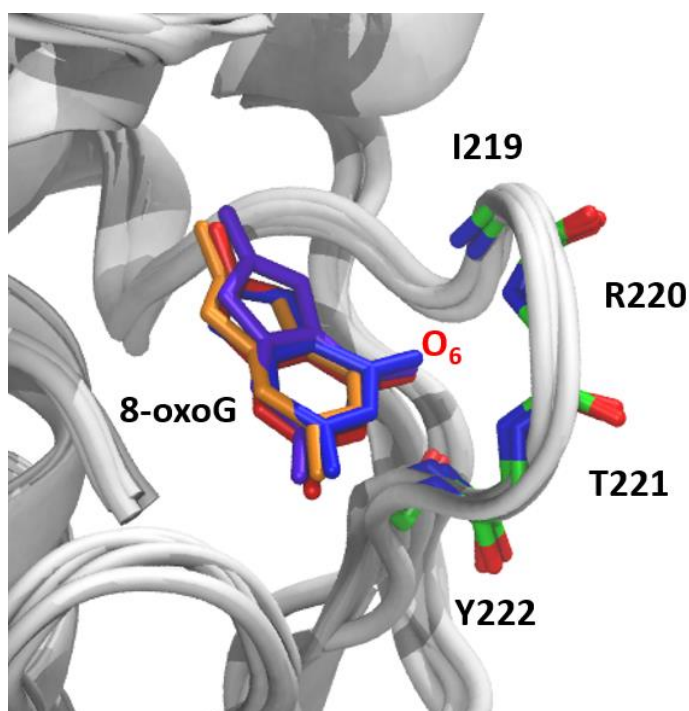
Figure 83 : Conservation de la couronne d'interactions de la boucle LCL dans les structures initiales du système boucle fermée
