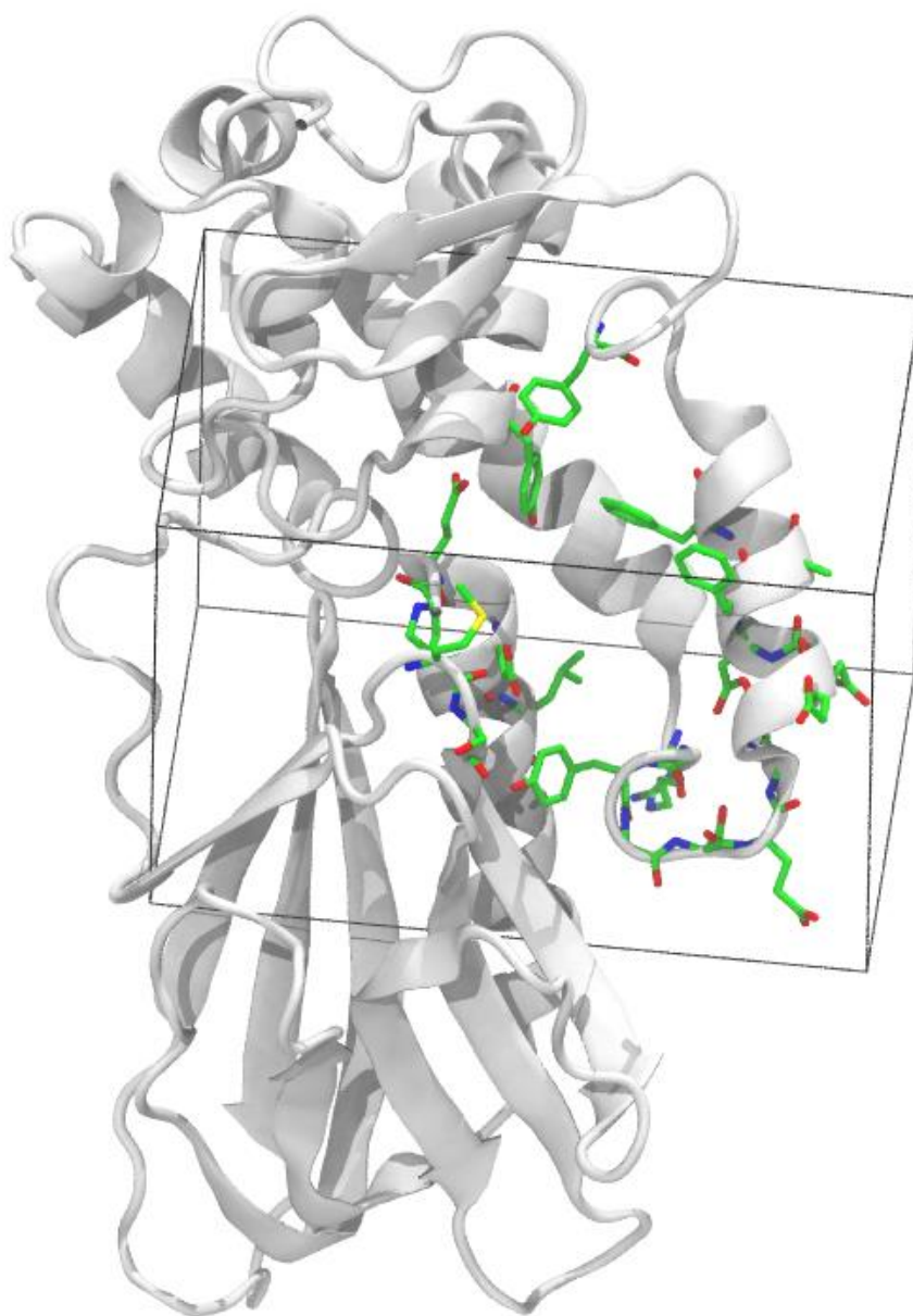
Figure 115 : Site actif de hNEIL1 criblé
