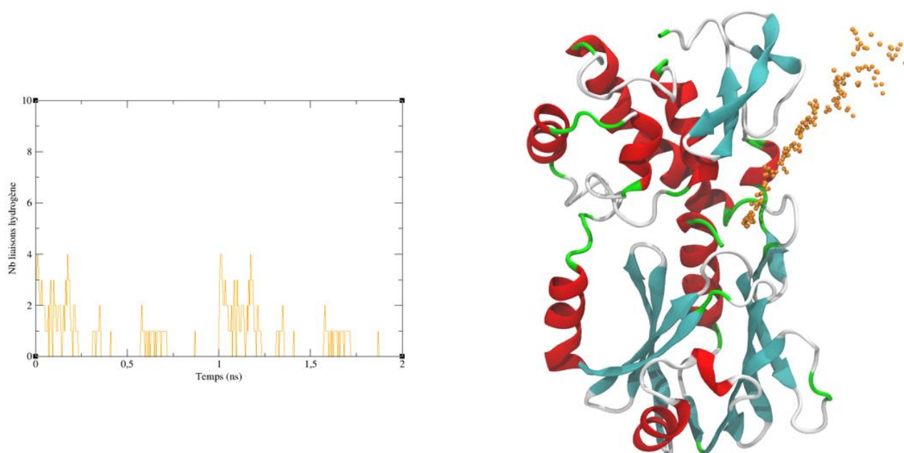
Figure 84 : Description des chemins de sortie empruntés par la base libre dans le système Fpg ADN THF (1PM5) boucle fermée (1XC8) 8-oxoG libre (1R2Y)
