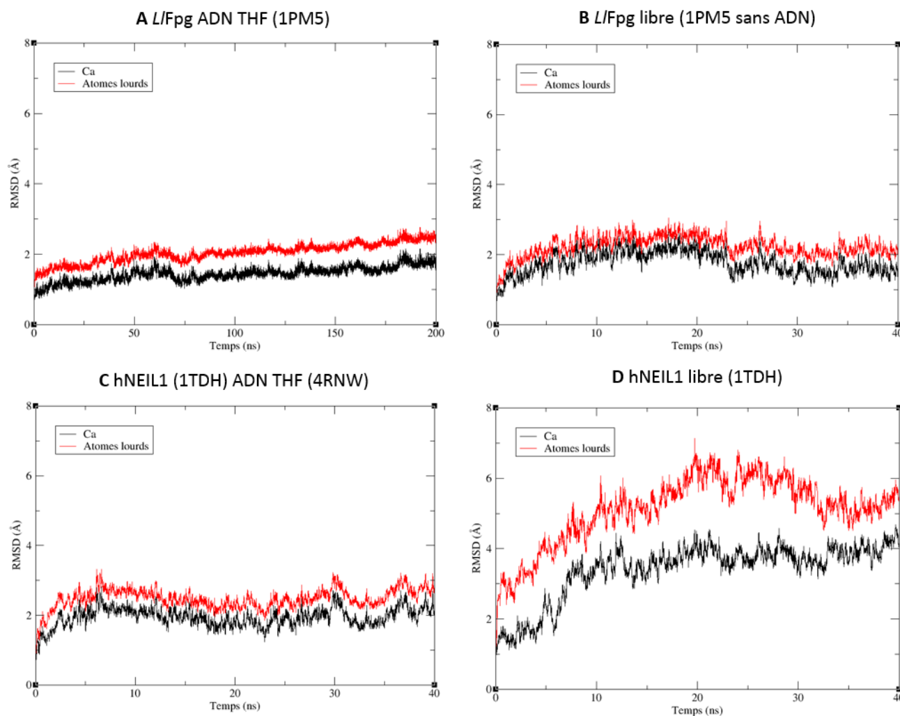
Figure 90 : Courbes de RMSD des quatre systèmes de L/Fpg et hNEIL1
