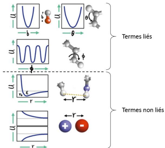
Figure 45 : Potentiels de liaison, d'angle de valence, d'angle dièdre et d'interaction à distance implémentés dans le champ de force d'Amber
