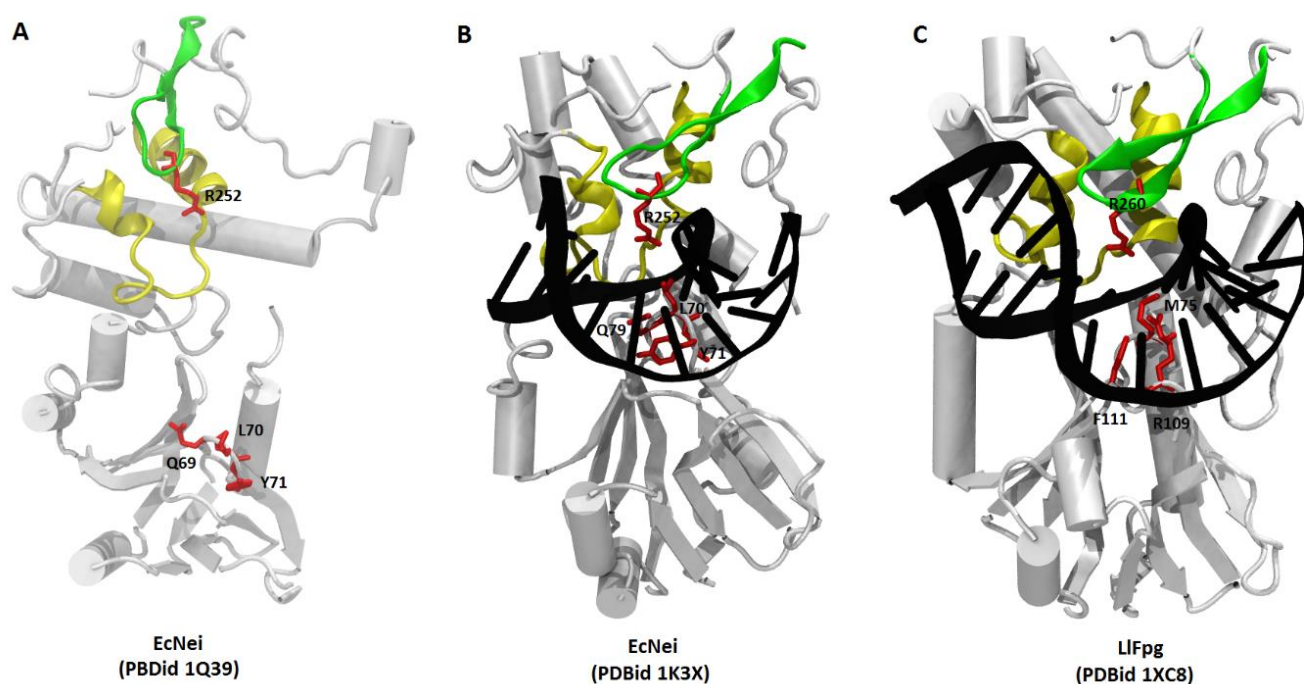
Figure 35 : Représentation de la triade d'intercalation de plusieurs Fpg/Nei libre ou complexées
