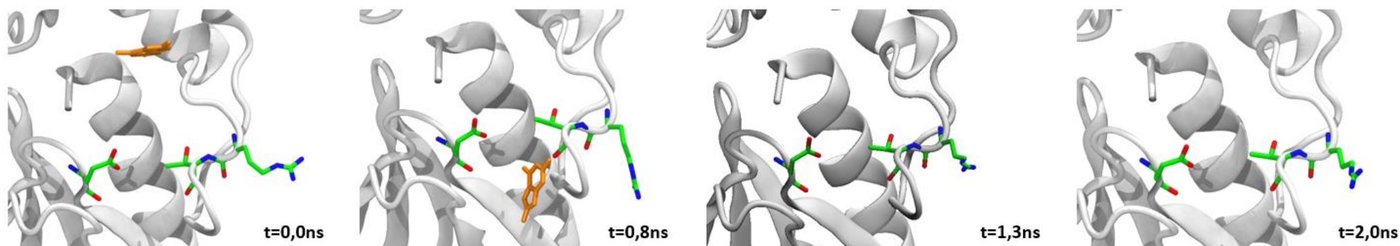
Figure 89 : Évolution de la position de la 8-oxoG dans les quatre TMD -1 s du système Fpg ADN THF boucle relâchée (1PM5) 8-oxoG libre (1R2Y)
