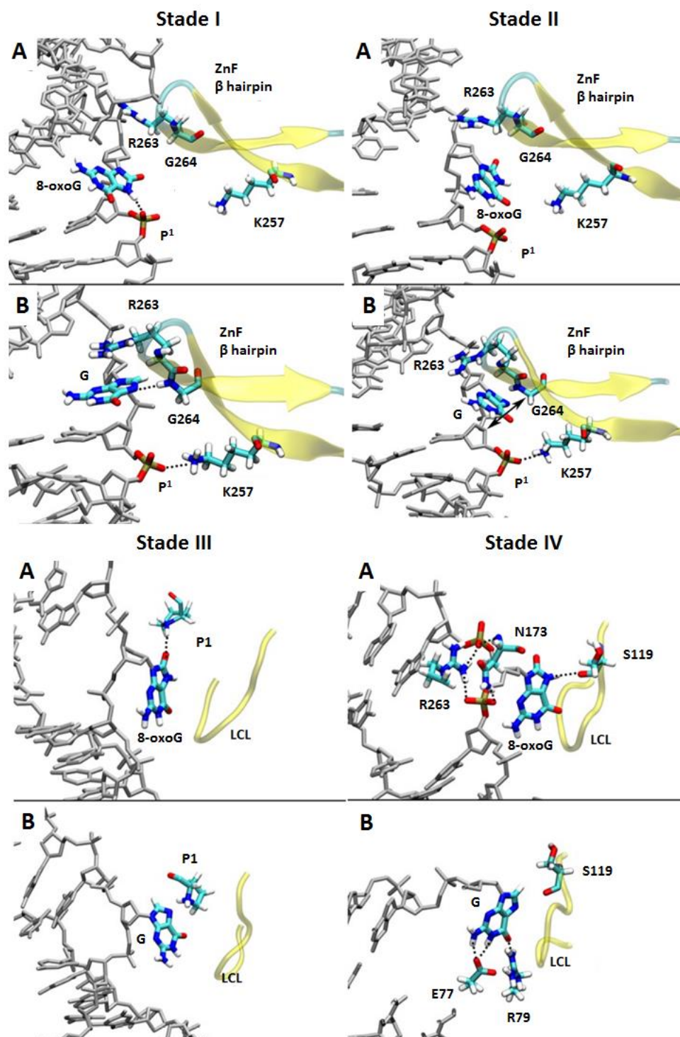
Figure 38 : Étude de la différenciation d'une 8-oxoG d'une G classique par Bst Fpg
