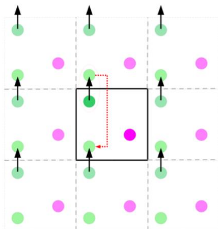
Figure 47 : Les conditions périodiques permettent de modéliser des systèmes « infinis »
