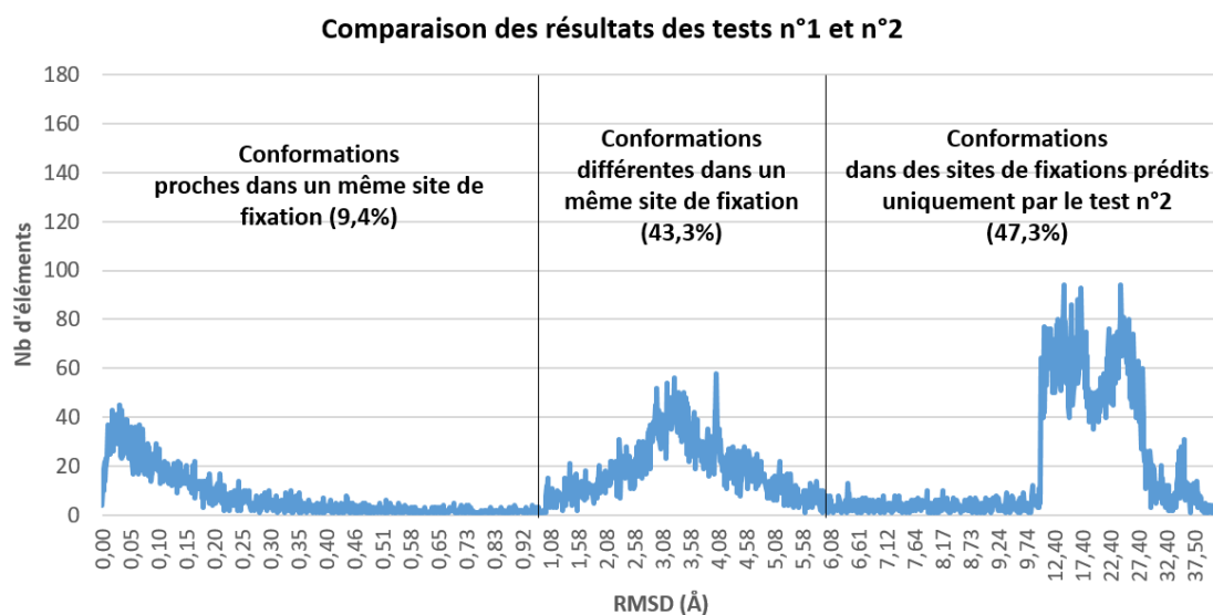
Figure 100 : Comparaison conformationnelle des poses générées par les tests n°1 et n°2 du docking sans a priori
