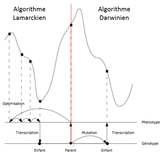
Figure 60 : Comparaison entre un algorithme génétique Lamarckien à gauche et Darwinien à droite
