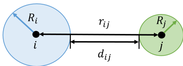
Figure 54 : Description de la distance d_{ij}
