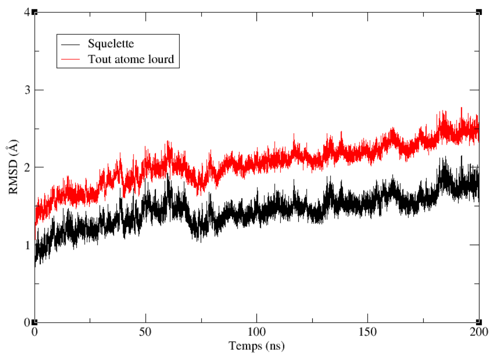
Fpg ADN FaPyG (1XC8) boucle LCL relâchée (1PM5)
