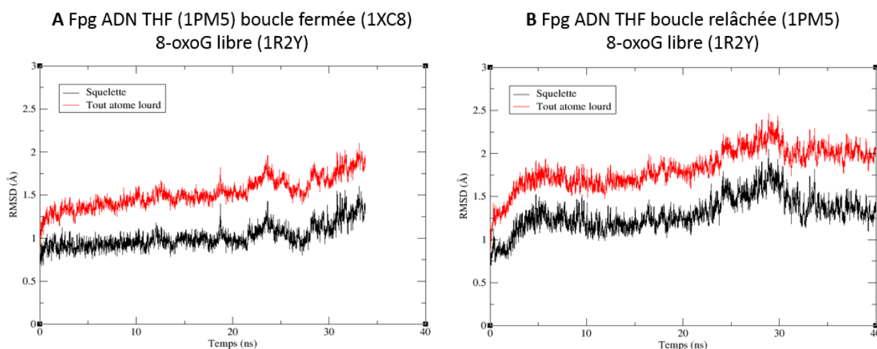
Figure 79 : Courbes de RMSD des deux systèmes produits en dynamique moléculaire classique A) Système Fpg ADN THF (1PM5) boucle fermée (1XC8) 8-oxoG libre (1R2Y) et B) Fpg ADN THF boucle relâchée (1PM5) 8-oxoG libre (1R2Y). En noir la RMSD sur le squelette (C, C \alpha , N et O) de la protéine et en rouge sur tous les atomes lourds (tous les atomes sauf les hydrogènes).
