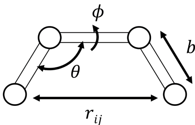
Figure 46 : Modélisation des molécules dans AMBER
