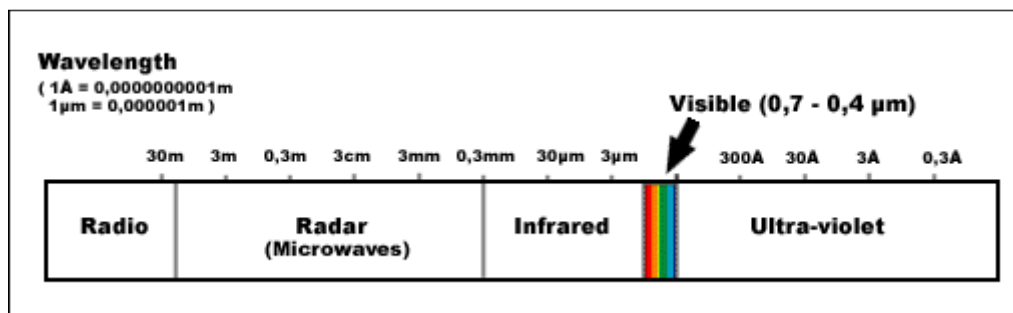
Figure 17 : Spectre électromagnétique
