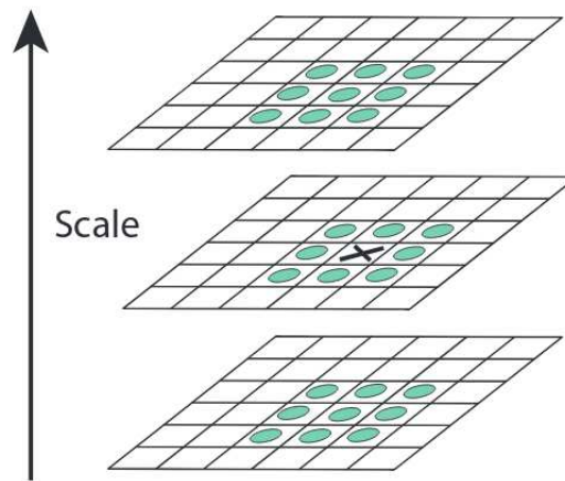
FIGURE 4.5 – Les maxima et les minima sont détectés en comparant un pixel (marqué avec X) à ses 26 voisins dans un voisinage 3x3x3 (marqué par des cercles) (source [2]).
