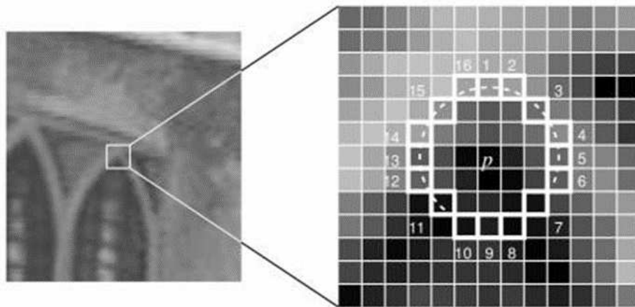
FIGURE 3.5 – Voisinage utilisé pour déterminer si un pixel est un point caractéristique ou non avec le détecteur FAST (source [1])
