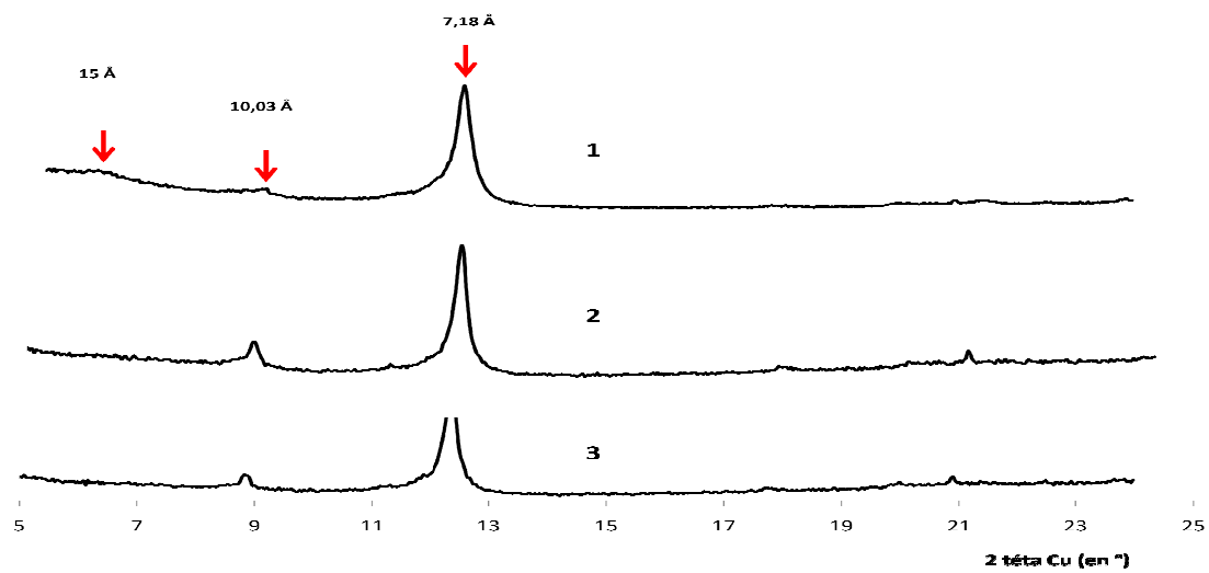
Figure 25: Diffactogrammes des différents traitements 1: Z+CP+C; 2 : Témoin ; 3 : CP+C (couche 0-10 cm)
