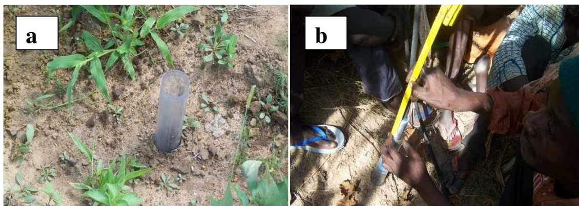
Figure 12 : Implantation du tube (a) et mesure d'humidité au champ (b) ( Sampieri 2014, Auteur Coulibaly Aboubacar)
