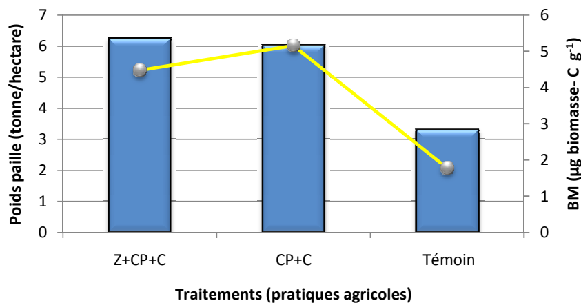
Figure 62 : Biomasse microbienne (µg biomasse-C g -1 ) et poids paille du sorgho (T/ha) cultivé au champ
