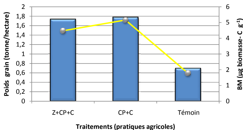
Figure 61 : Evolution de la biomasse microbienne (µg biomasse-g -1 ) et du poids des grains du sorgho (T/ha) cultivé au champ
