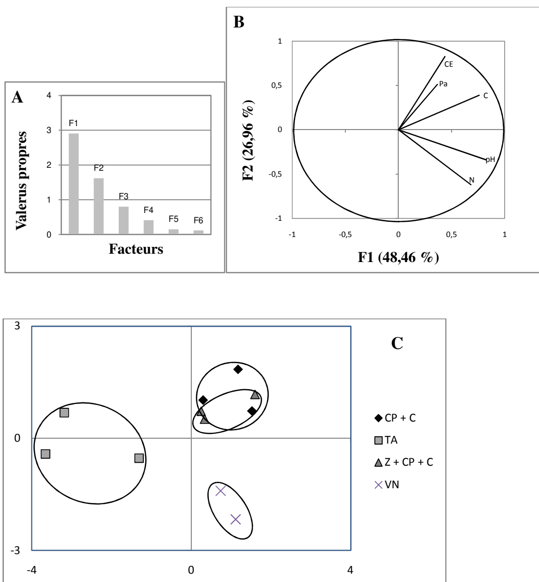
Figure 56 : Résultats de l'ACP pour la base de données des analyses physiques et chimiques (12 observations). A : Valeurs propres en fonction des facteurs. B: Projection des variables dans le plan F1-F2. C : Projection dans le plan F1-F2 des observations.
