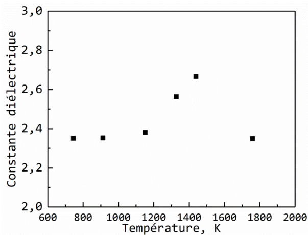
Figure 5-26, constante diélectrique de l'échantillon Syn-10Fe en fonction de la température.
