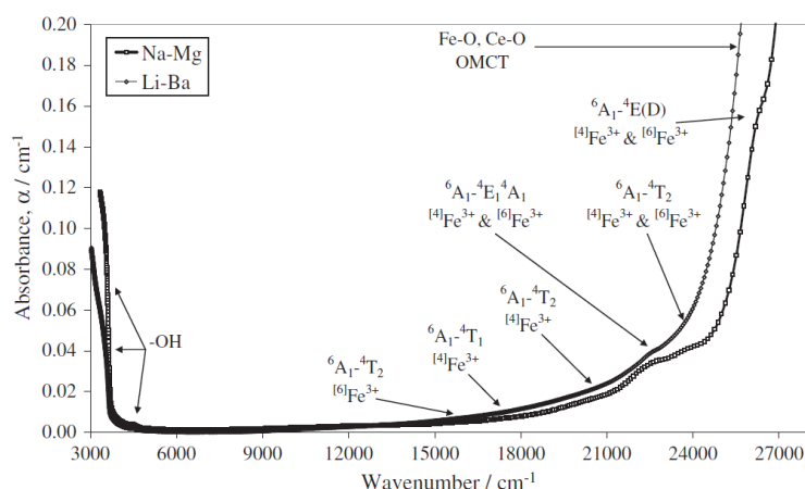
Figure 3-7, absorbances des verres 60\text{SiO}_2\cdot 20\text{Na}_2\text{O}\cdot 20\text{MgO}\cdot [+0,25\text{ mol\% Fe}_2\text{O}_3] et 60\text{SiO}_2\cdot 20\text{Li}_2\text{O}\cdot 20\text{BaO}\cdot [+0,25\text{ mol\% Fe}_2\text{O}_3] (Bingham et al., 2014).
