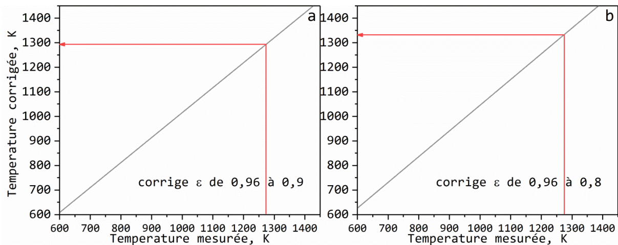
Figure 5-38, représentation de la relation entre température mesurée et corrigée, a) une modification d'émittance de 0,96 à 0,9; b) une modification d'émittance de 0,96 à 0,8.
