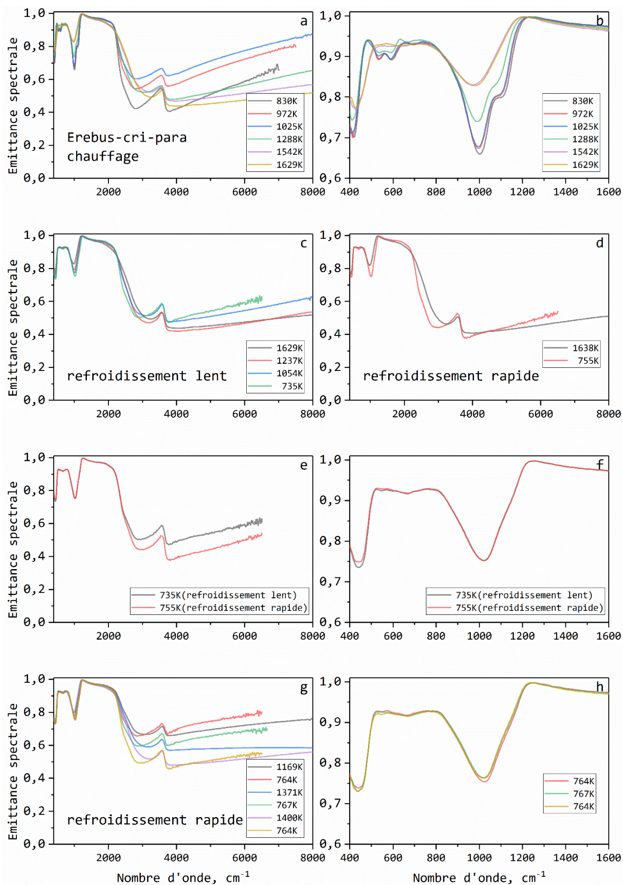
Figure 4-12, évolution de l'émittance de l'échantillon Erebus-cri-para au cours du traitement thermique, a) émittance entre 830K et 1629K; b) zone phonon entre 400 et
