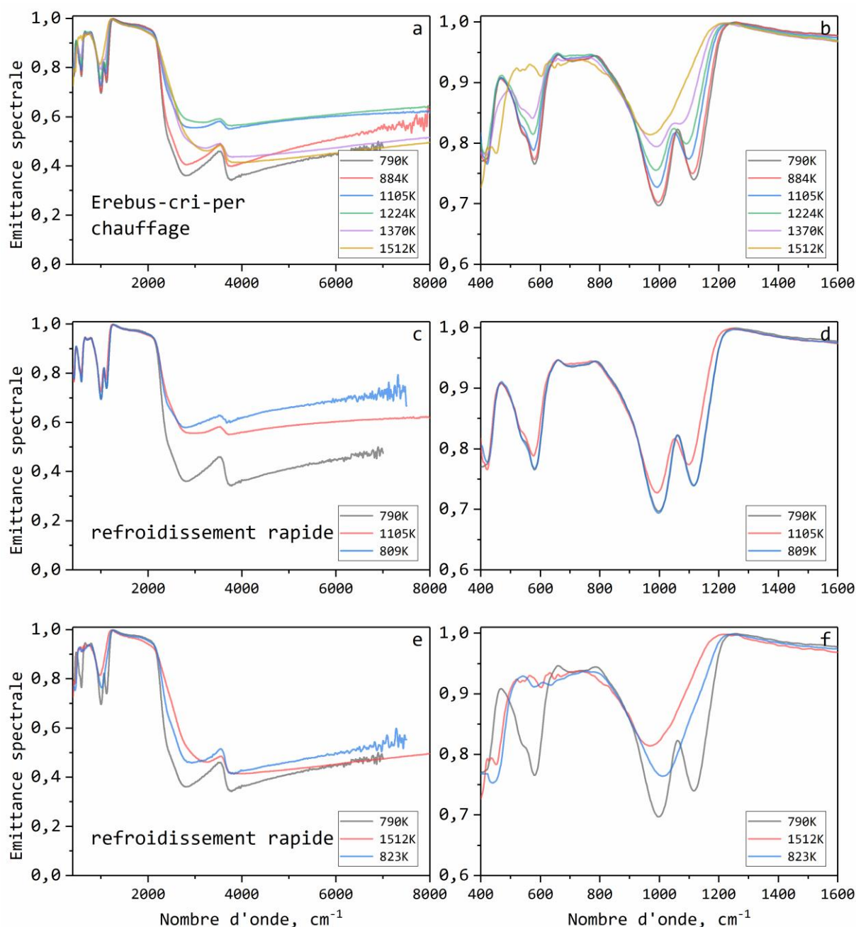
Figure 4-10, émittance d'Erebus-cri-per, a) l'émittance pendant le chauffage de 790K à 1512K entre 400 et 8000 cm -1 ; b) l'émittance pendant le chauffage entre 400 et 1600 cm -1 ; c) l'émittance après refroidissement rapide de 1105K à 809K entre 400 et 8000 cm -1 ; d) l'émittance après refroidissement rapide entre 400 et 1600 cm -1 ; e) l'émittance après refroidissement rapide de 1512K à 809K; f) l'émittance après refroidissement rapide entre 400 et 1600 cm -1 .
