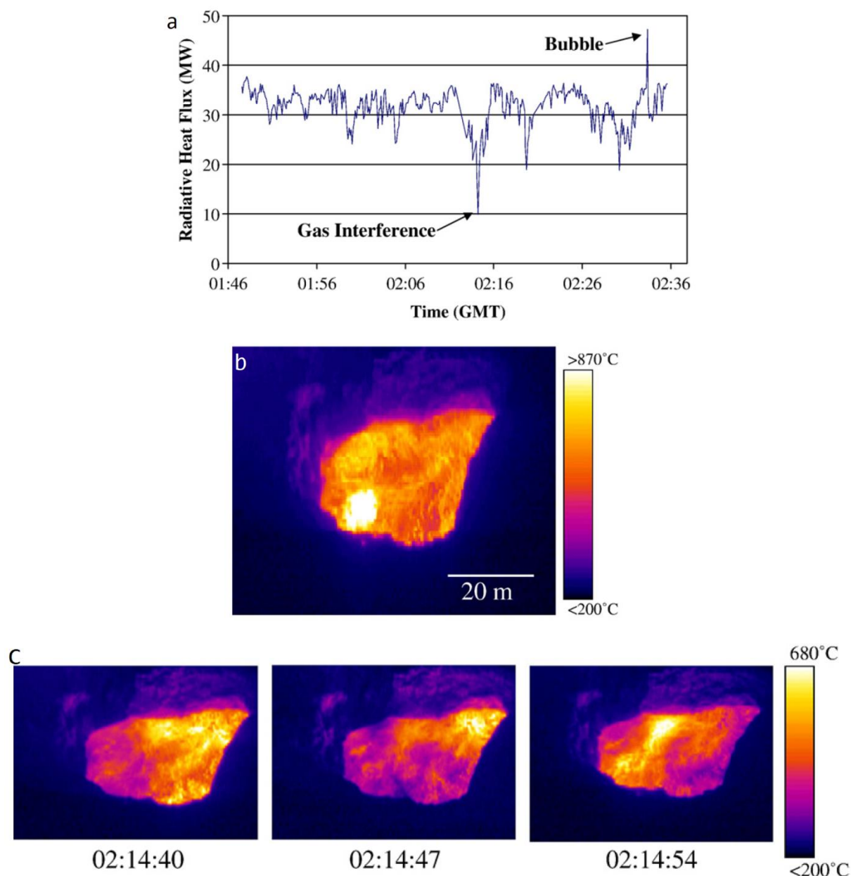
Figure 1-9, a) variation du flux radiatif de la surface pendant l'éruption de bulles de gaz. b) image thermique de l'explosion d'une bulle de gaz à la surface du lac Ray. c) séquence d'images montrant le refroidissement effectif du lac de lave par l'extrusion d'un nuage de gaz à mesure qu'il bouge de droite à gauche ( Calkins, Oppenheimer et Kyle, 2008 ).
