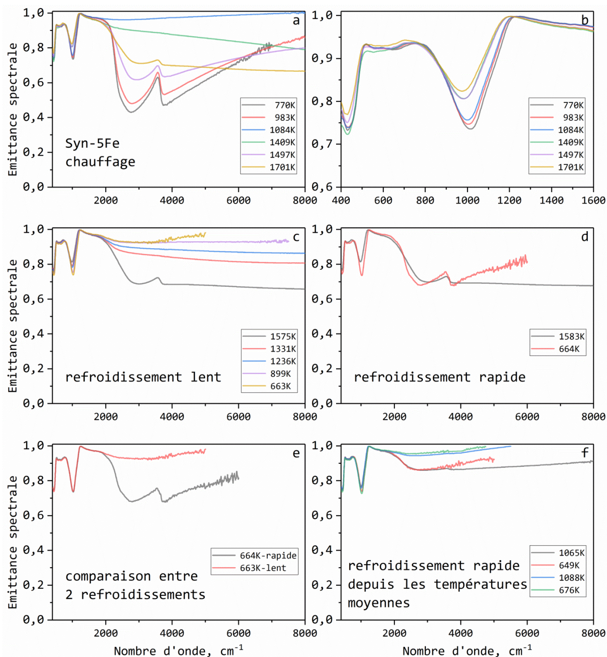
Figure 4-19, évolution en température de l'émittance de l'échantillon Syn-5Fe, a) au cours du chauffage de 770K à 1701K; b) de 770K à 1701K-zoom sur les basses fréquences; c) refroidissement lent de 1575K à 663K; d) refroidissement rapide de 1583K à 664K; e) comparaison des deux types de refroidissement à basse température; f) refroidissement rapide à partir de 1065K et de 1088K.
