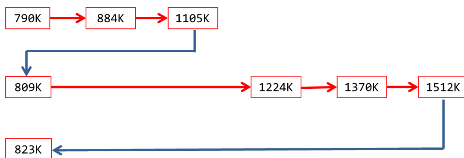
Figure 4-9, traitement thermique et températures mesurées pour l'échantillon Erebus-cri-per.
