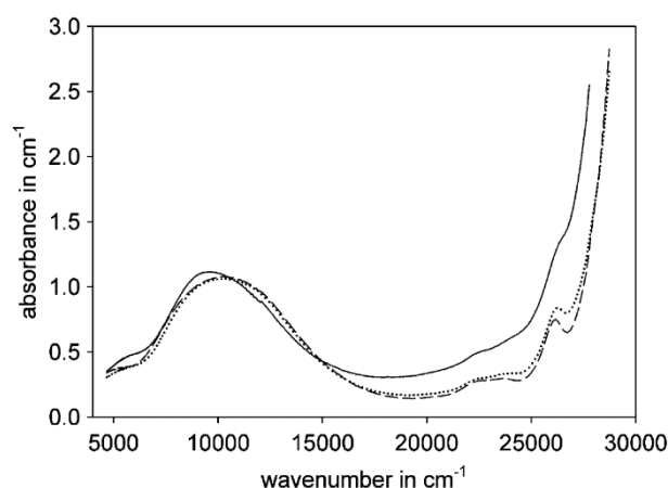
Figure 3-4, spectres optiques de verres de compositions x\text{Na}_2\text{O} \cdot 10\text{MgO} \cdot 10\text{Al}_2\text{O}_3 \cdot (80-x)\text{SiO}_2 [+0,25 \text{ mol\% Fe}_2\text{O}_3] , (—) x=10 , (···) x=15 , (- -) x=20 (Carl, Gerlach et Rüssel, 2007).
