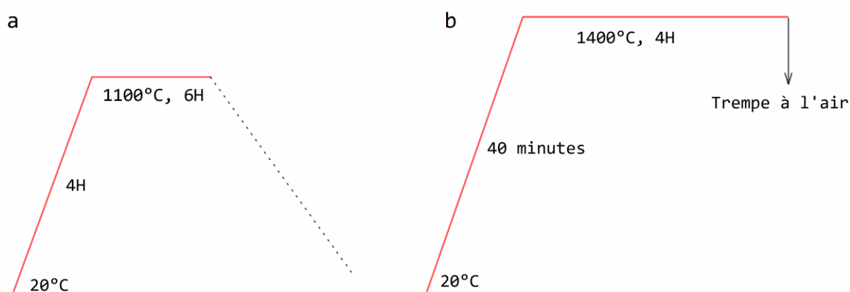
Figure 2-10, a) programme de la décarbonation, b) programme de la fusion d'échantillons de synthèse.
