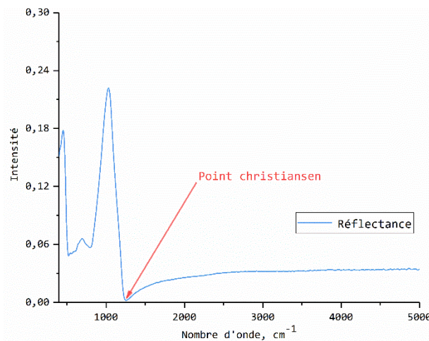
Figure 3-19, le point Christiansen sur la réflectance d'un échantillon Erebus poudre.
