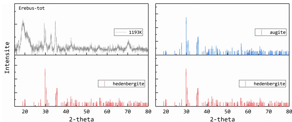
Figure 5-16, diffractogramme de l'échantillon Erebus-tot à 1193K et tentative d'identification de la phase cristallisée: augite ou hedenbergite.
