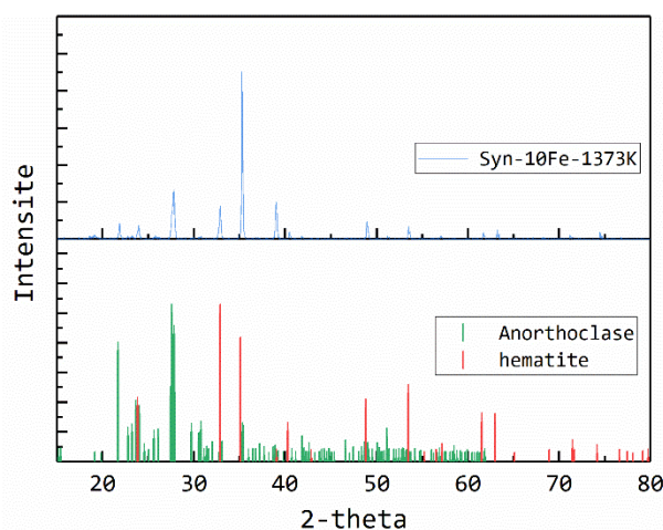
Figure 5-32, diffractogramme de l'échantillon Syn-10Fe à 1373K et ceux de l'hématite et de l'anorthoclase ( \text{Na}_{0,63}\text{K}_{0,27}\text{Ca}_{0,1}\text{Al}_{1,1}\text{Si}_{2,9}\text{O}_8 ).
