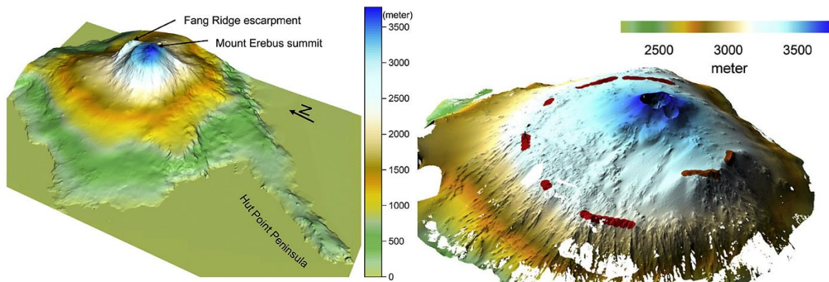
Figure 1-6, modèle numérique du mont Erebus (Csatho et al., 2008), a) visualisation 3D du Mont Erebus, crée à partir de Ross Island DEM (Digital Elevation Model); b) représentation 3D du DEM ALS (airbone laser scanning) montrant les affleurements de coulée pré-caldeira autour de la caldeira.
