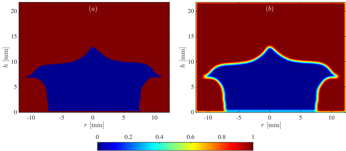
FIGURE C.1 – (a) Image binarisée d'une flamme de méthane à la stœchiométrie à t = 10 \text{ ms} acquise en utilisant le diagnostic de tomographie laser. (b) Application du filtre Gaussien de taille 30 \times 30 \text{ px}^2 à l'image binarisée (a).
