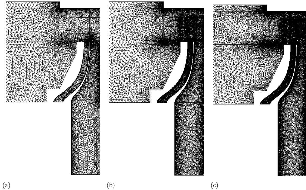
FIGURE B.2 – Différents maillages étudiés. (a) : grossier M_g , (b) : intermédiaire M_i et (c) : fin M_f .
