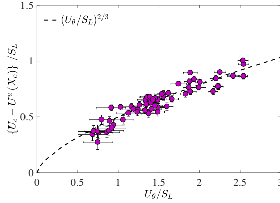
FIGURE 3.13 – La vitesse de convection U_c - U^u(X_c) , où U^u(X_c) est la vitesse de l'écoulement non perturbée au niveau du centre de vortex X_c , en fonction de U_\theta . La ligne en pointillée est donnée par 0.5(U_\theta/S_L)^{2/3} .
