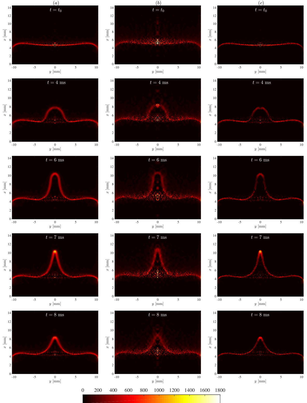
FIGURE 3.7 – Séquence temporelle de l'interaction d'une flamme propane/air à \phi = 0.9 avec un vortex toroïdal ayant une intensité U_\theta/S_L = 2.6 : colonne (a) \text{CH}^* , colonne (b) \text{CO}_2^* et colonne (c) la différence entre \text{CH}^* et \text{CO}_2^* . Une déconvolution d'Abel a été appliquée aux images pour récupérer l'information en 2D.
