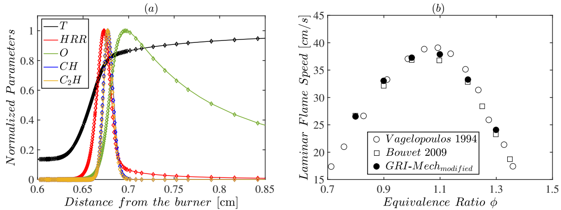
FIGURE 2.16 – (a) Effet de l'addition des réactions OH^* et CH^* sur la température, le taux de dégagement de chaleur ( HRR ) et les fractions molaires normalisées O , CH et C_2H pour une flamme méthane/air prémélangée à \phi = 1.0 , en utilisant le GRI-Mech original 3.0 (symboles) et le GRI-Mech 3.0 incluant les espèces excitées (lignes). (b) Comparaison des vitesses de flamme laminaire calculées en utilisant le GRI-Mech 3.0 modifié avec les données expérimentales de VAGELOPOULOS et al. 1994 et BOUVET 2009.
