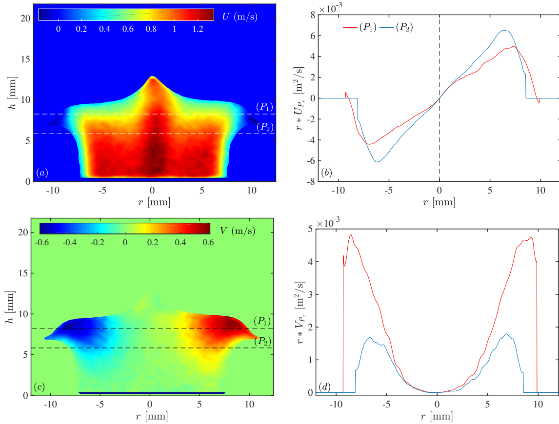
FIGURE C.4 – Champs de vitesse axiale (a) et radiale (c) de la flamme méthane/air à t = 10 ms. (P_1) et (P_2) représentent les deux positions où les vitesses ont été tracées (b) et (d).
