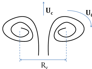
FIGURE 2.32 – Caract  ristiques d'un vortex toro  dal : U_c sa vitesse de convection, U_\theta sa vitesse de rotation et R_v l'inter-distance entre les deux noyaux du vortex.
