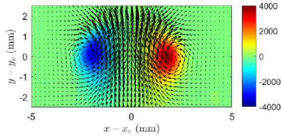
FIGURE 5.14 – Champ de vitesse mesuré à l'aide de la PIV superposé sur le champ de vorticit . Le rep re est centr  sur le centre du vortex instantan  ( x_v, y_v ).
