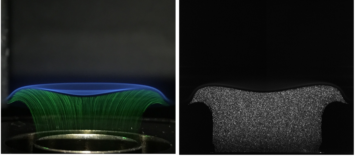
FIGURE 2.6 – (Gauche) Photographie et (droite) exemple d'image de tomographie laser par diffusion de Mie d'une flamme de propane à \phi = 1.2 .
