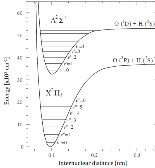
FIGURE 1.10 – Schéma simplifié des niveaux d'énergie du radical OH pris du travail de LUQUE et CROSLLEY 1998. Les deux courbes représentent l'état électronique fondamental ( X^2\Pi_i ) et l'état électroniquement excité ( A^2\Sigma^+ ) et qui sont décomposées en multiples états vibrationnels \nu'' à l'état fondamental et \nu' à l'état excité.
