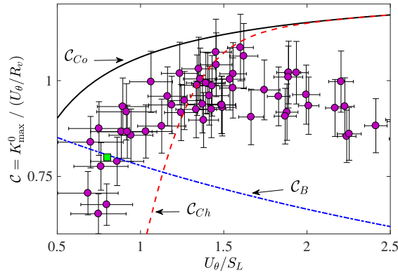
FIGURE 3.12 – Fonction d'efficacité \mathcal{C} = K_{max}^0 / (U_\theta/R_v) en fonction de U_\theta/S_L . Les lignes labelisées \mathcal{C}_{Co} , \mathcal{C}_{Ch} , et \mathcal{C}_B correspondent respectivement aux expressions paramétriques fournies par COLIN et al. 2000, CHARLETTE et al. 2002 et BOUGRINE et al. 2014 corrigées par l'Eq. (3.10) afin d'obtenir K_{max}^0 . Les symboles en cercles correspondent aux mesures expérimentales tandis que le symbole en carré vert est extrait du travail de BOUGRINE et al. 2014.
