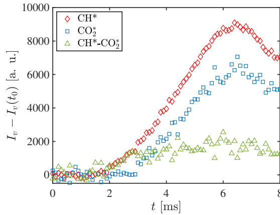
FIGURE 3.8 – Évolution de l'intensité durant l'interaction de la flamme propane/air à \phi = 0.9 avec un vortex toroïdal ayant une intensité U_\theta/S_L = 2.6 .
