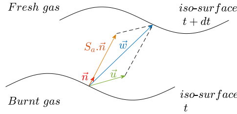
FIGURE 1.2 – Vitesses d'une flamme laminaire prémélangée.
