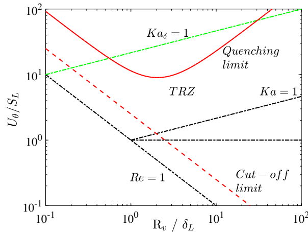
FIGURE 1.7 – Diagramme de combustion proposé par BORCHI 1985 et modifié par POINSOT et al. 1991b et PETERS 1999. Les traits en rouge correspondent aux limites proposées par POINSOT et al. 1991b et le trait en vert à celle proposée par PETERS 1999 .
