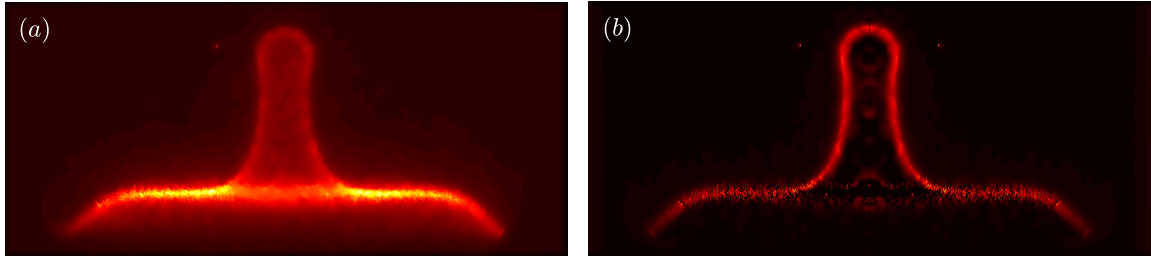
FIGURE 2.30 – Chimiluminescence du radical \text{CH}^* : (a) avant et (b) après déconvolution d'Abel.
