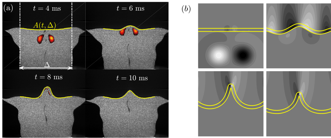
FIGURE 4.5 – S quence d'interaction d'une flamme m thane   la stoechiom trie : (a) Contours de vorticit  et isotherme c t  gaz frais superpos s sur les images issues de la tomographie laser. (b) Champs de vorticit  issus de la DNS avec superposition des iso-contours   Y_f^* = 0.01 et Y_f^* = 0.99 . Notons que le champ DNS a  t  doubl  par sym trie.
