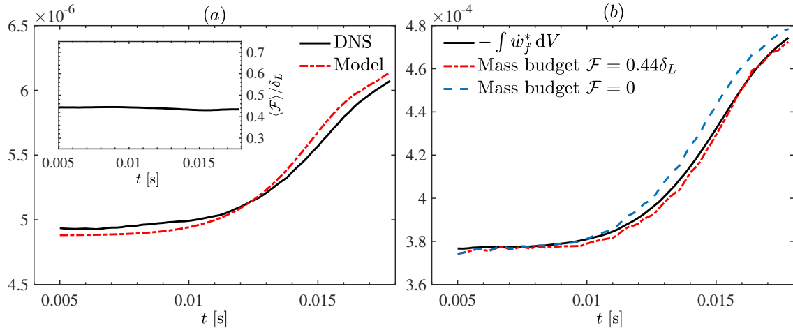
FIGURE 4.6 – (a) Évolution temporelle de la masse contenue dans la flamme déterminée depuis la DNS effectuée (terme de gauche de l'Eq. (4.42)) et du modèle avec \mathcal{F} = \text{cst} = 0.44\delta_L (terme de droite de l'Eq. (4.42)). La sous-figure se trouvant en haut à gauche représente l'évolution temporelle du rapport \mathcal{F}/\delta_L . (b) Le taux de réaction du carburant intégré sur le volume a été calculé à partir de la DNS et comparé au bilan de masse en utilisant \mathcal{F} = 0 et \mathcal{F} = \text{cst} = 0.44\delta_L . \mathcal{F} = \text{cst} = 0.5\delta_L a été également testé et la courbe obtenue a été superposée sur \mathcal{F} = \text{cst} = 0.44\delta_L (aucune différence entre les deux cas n'a été relevée).
