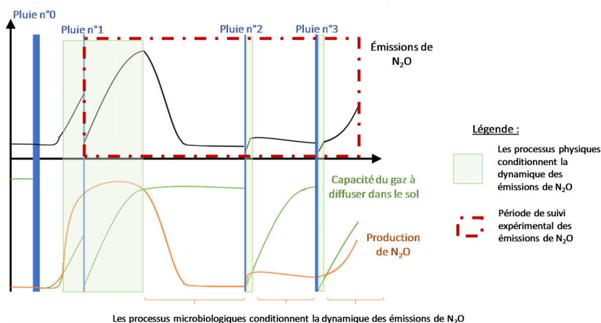
Figure 2-13 : Rôle des processus microbiologiques et physiques dans la dynamique des émissions de N_2O : schéma explicatif de l'hypothèse proposée pour expliquer les observations lors du suivi expérimental.
