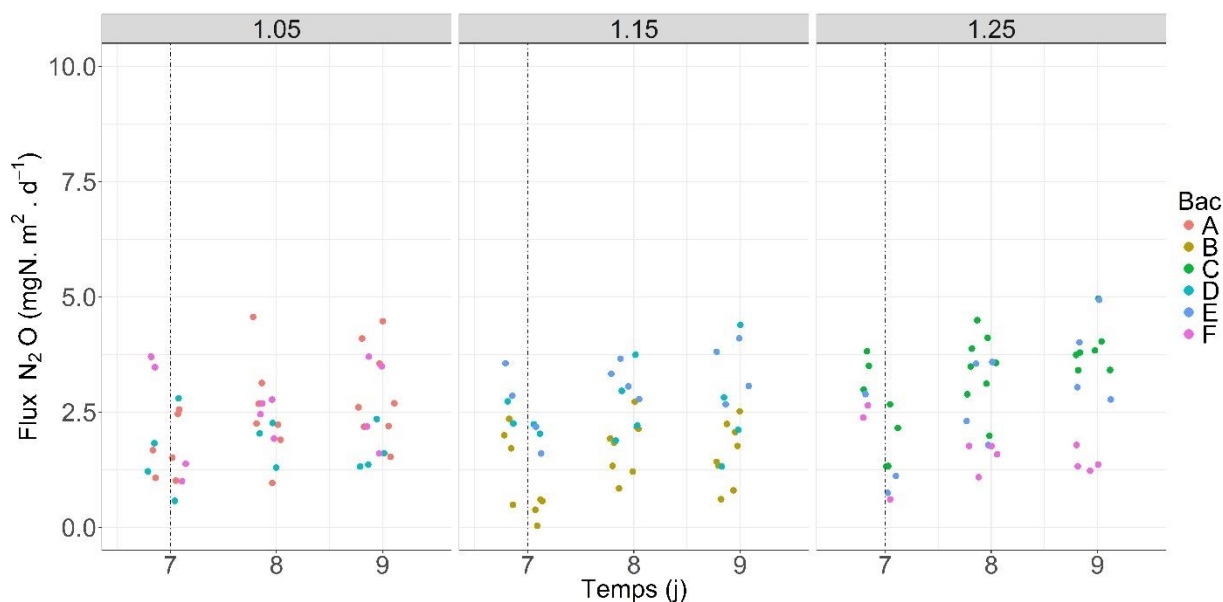
Figure 2-9 : Flux de N_2O mesurés les 7, 8 et 9 e jours du suivi expérimental pour les trois masses volumiques initiales visées. La ligne en pointillé correspond à la pluie n°2 simulée (5 mm.h -1 , 30 mn).
