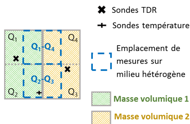
Figure 2-4 : Localisation des emplacements de mesure Q1-Q4 et Q2-Q3
