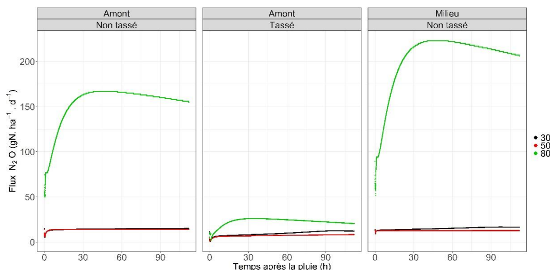
Figure 4-14 : Emissions de N_2O simulées pour une pluie de 30 mn à 16 \text{ mm.h}^{-1} et une pente à 5 % pour trois valeurs d'humidité initiale : 30 %, 50 % et 80 % de la teneur en eau volumique à saturation.
