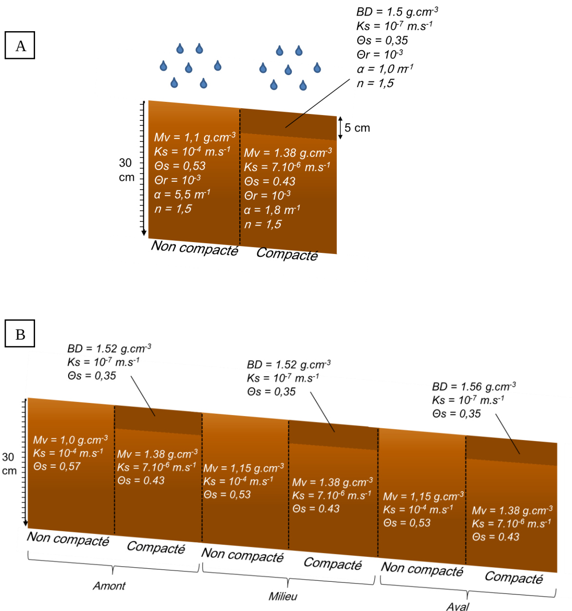
Figure 4-4 : A) Paramètres hydrodynamiques moyens utilisés lors des simulations dans les conditions expérimentales. B) Variation des paramètres hydrodynamiques entre les emplacements de simulation.
