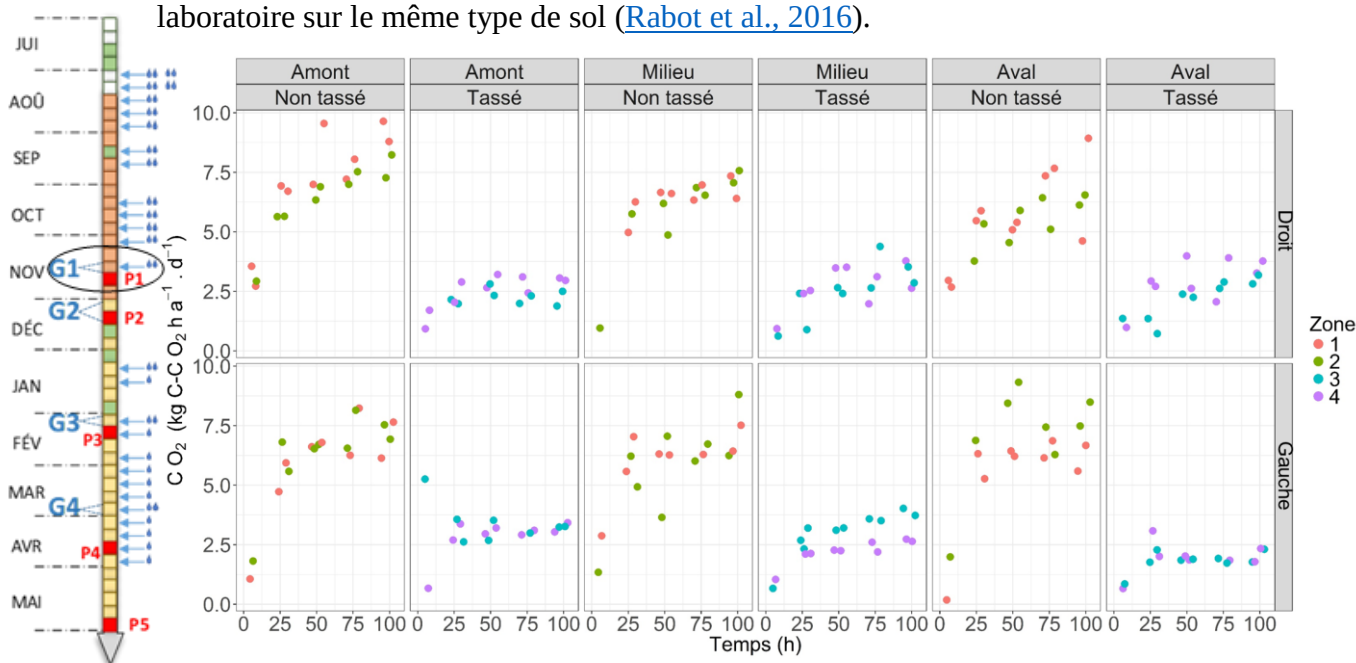
Figure 3-21 : Evolution des émissions de CO 2 sur les 100 premières heures suivant la simulation d'une pluie en kgC-CO 2 .ha -1 .d -1 (suivi G1). La pluie est réalisée au temps 0 h.
