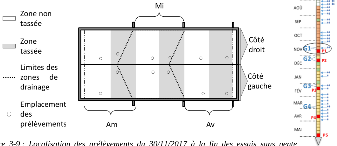
Figure 3-9 : Localisation des prélèvements du 30/11/2017 à la fin des essais sans pente (prélèvements P1).
