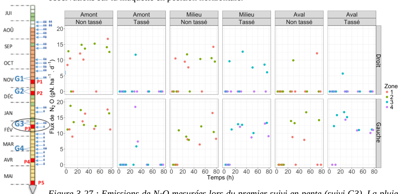
Figure 3-27 : Emissions de N 2 O mesurées lors du premier suivi en pente (suivi G3). La pluie est réalisée au temps 0 h.
