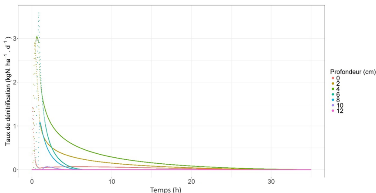
Figure 4-11 : Taux de dénitrification simulé dans les 12 premiers centimètres pour la zone aval tassée.
