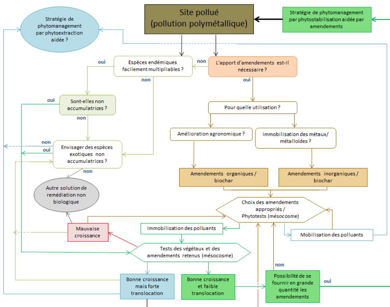
Figure 5.1 : Outil d'aide à la décision en vue de la mise en place d'une stratégie de phyomanagement par phytostabilisation de sites pollués par des métaux et métalloïdes assisté par des amendements.
