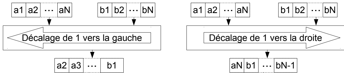
FIGURE 2.12 – Le décalage des données en registre vectoriel.
