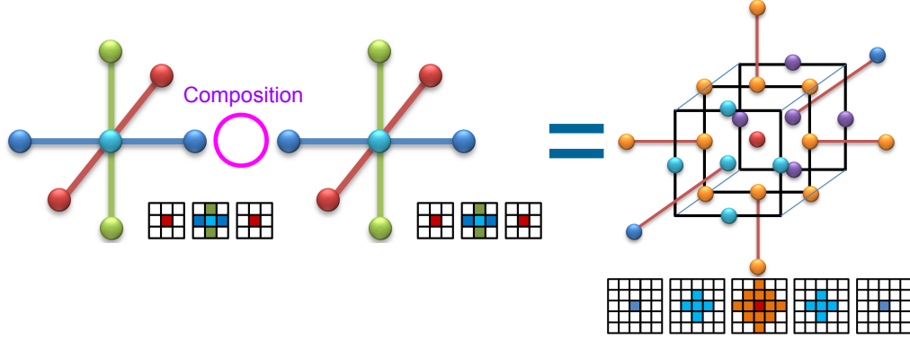
FIGURE 3.20 – Le stencil 25-point (à gauche) correspondant à la composition de deux noyaux 7-point (à droite).
