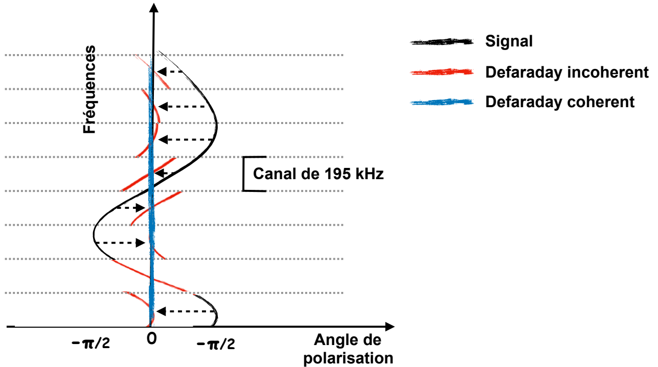
FIGURE 7.9 – Schéma comparant les deux méthodes de defaraday. En rouge, le defaraday incohérent, en bleu le defaraday cohérent. Il y est représenté en noir l'impulsion d'un pulsar fortement affecté par la rotation Faraday. Les canaux sont séparés par des pointillés gris (195 kHz pour LOFAR et NenuFAR) tandis que les courbes rouge et bleu représentent le signal après les correction incohérente et cohérente respectivement.
