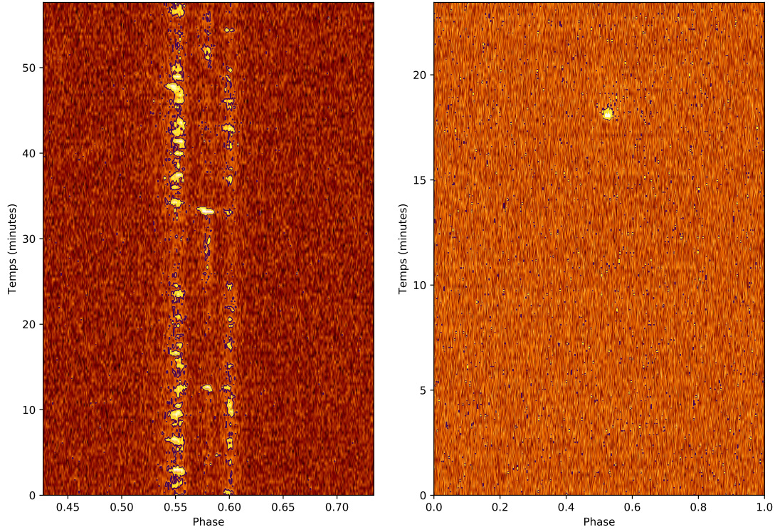
FIGURE 4.3 – Observation de deux pulsars à changement de modes avec NenuFAR. À gauche, B1237+25 où l'on aperçoit une composante centrale apparaître dans un mode puis disparaître dans l'autre (voir dans Backer (1970)). À droite, se trouve B0823+26 pour lequel un des modes est 1000 fois plus intense (visible à 17 minute) que l'autre (pulsar étudié dans Sobey et al. (2015)).
