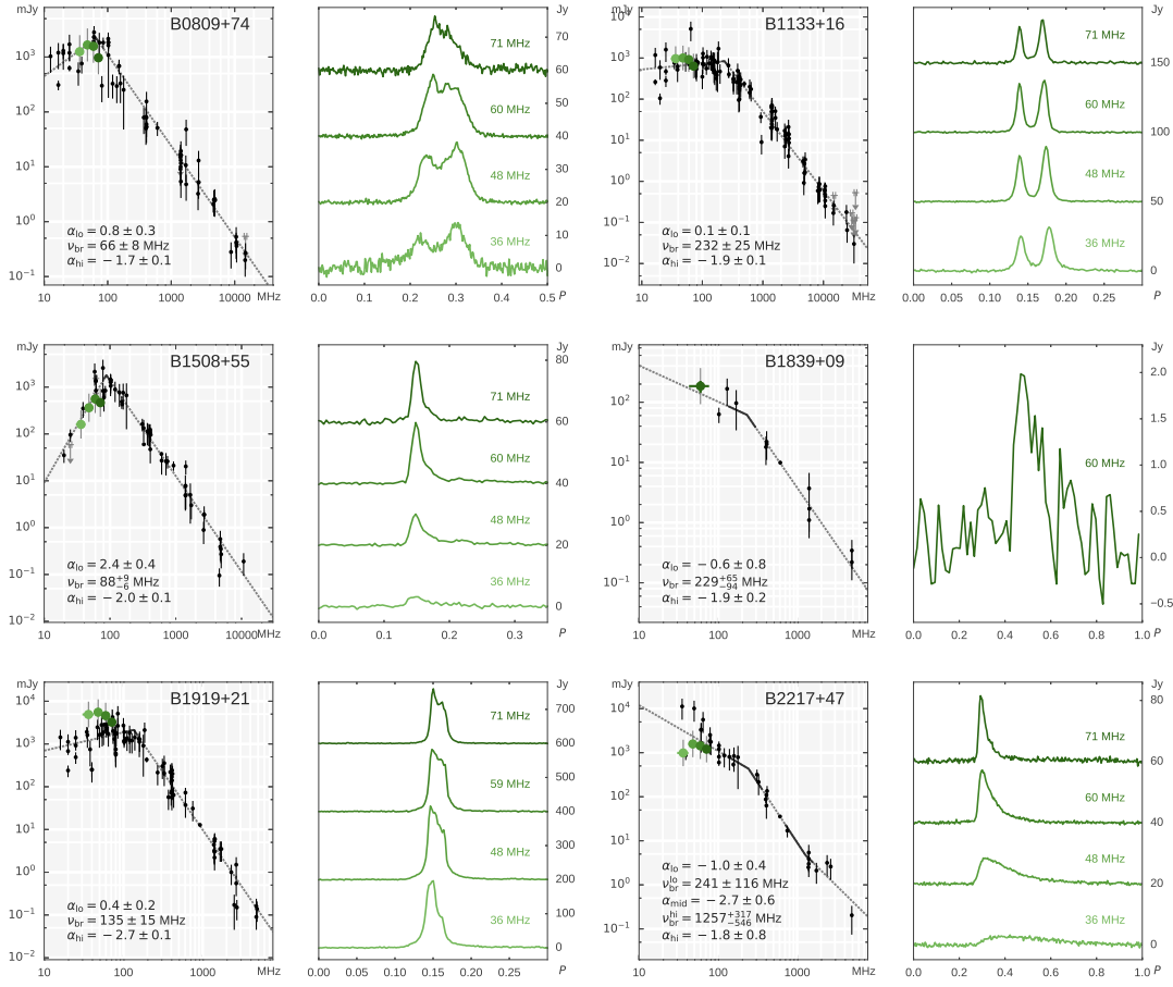
FIGURE 10.4 – Spectres et profils pour six observations du relevé de LOFAR cœur. Dans les spectres sont représentées en noir les valeurs extraites de la littérature et en vert les densité de flux moyennes calculées à partir des profils calibrés adjacents (un profil par valeur de flux). Les pulsars avec un ratio signal-sur-bruit important sont découpés en quatre canaux donnant une dimension fréquentielle aux profils et aux flux.
