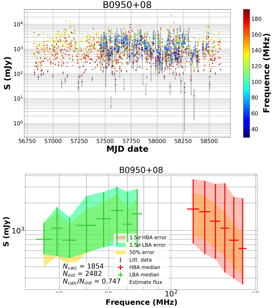
FIGURE D.8 – Suivi de B0950+08 par la station LOFAR FR606 en HBA et LBA. Dans le panneau supérieur : graphique du flux moyen en fonction du MJD (Modified Julian Date) et de la fréquence (échelle de couleurs sur la droite). Les points représentés avec des flèches grises sont des limites supérieures. Dans le panneau inférieur : spectre médian du même pulsar avec une erreur de 1.5\sigma (surface verte pour les LBA et rouge pour les HBA). L'erreur habituelle de 50 % est représentée par la surface jaune. Les crois bleus sont les observations utilisées pour la construction du spectre médian. Les crois grises sont les flux provenant de la littérature utilisées pour construire le spectre théorique (en gris) en loi de puissance provenant de Bilous et al. (2016).
