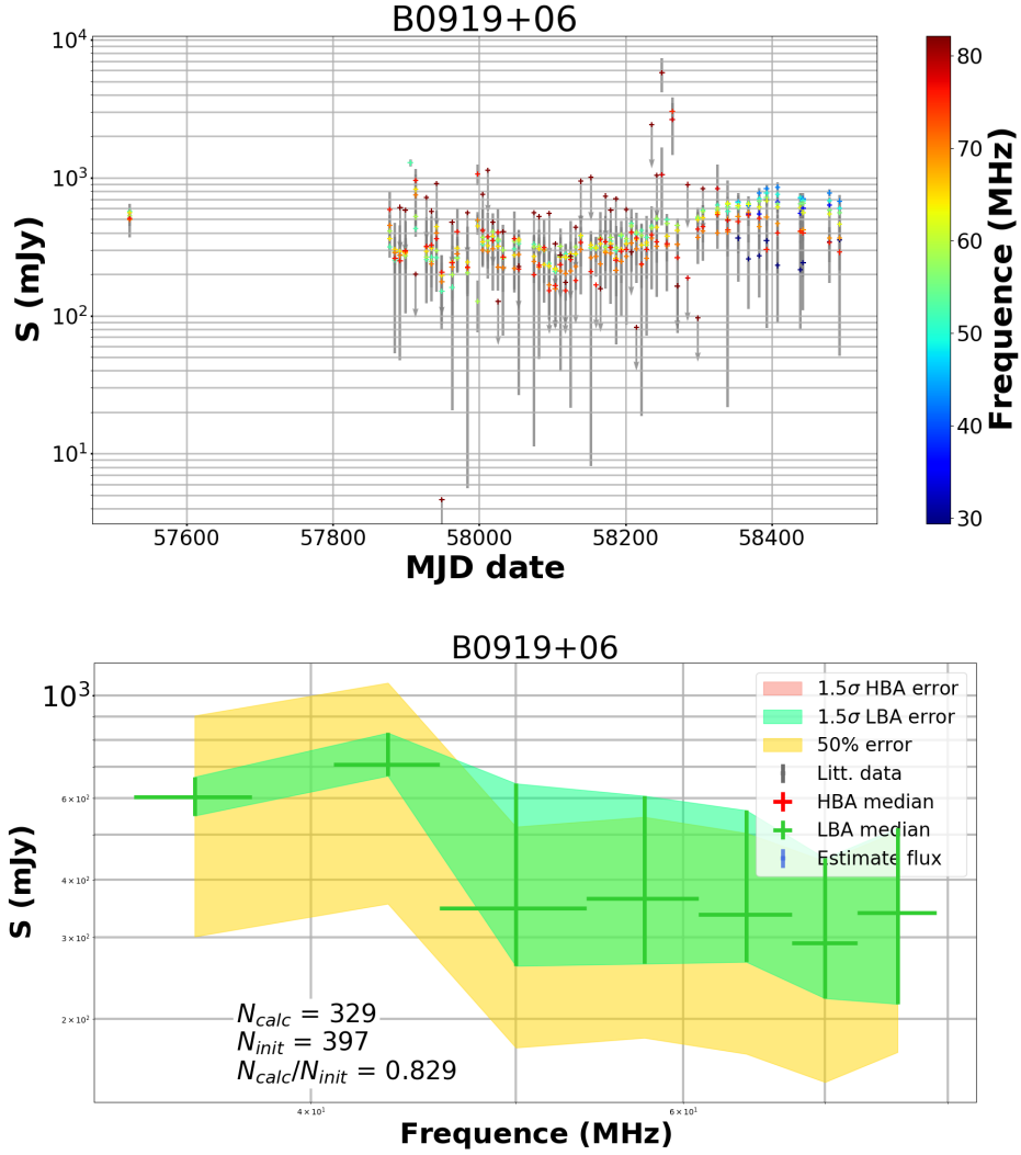
FIGURE D.6 – Suivi de B0919+06 par la station LOFAR FR606 en HBA et LBA. Dans le panneau supérieur : graphique du flux moyen en fonction du MJD (Modified Julian Date) et de la fréquence (échelle de couleurs sur la droite). Les points représentés avec des flèches grises sont des limites supérieures. Dans le panneau inférieur : spectre médian du même pulsar avec une erreur de 1.5\sigma (surface verte pour les LBA et rouge pour les HBA). L'erreur habituelle de 50 % est représentée par la surface jaune. Les crois bleus sont les observations utilisées pour la construction du spectre médian. Les crois grises sont les flux provenant de la littérature utilisées pour construire le spectre théorique (en gris) en loi de puissance provenant de Bilous et al. (2016).
