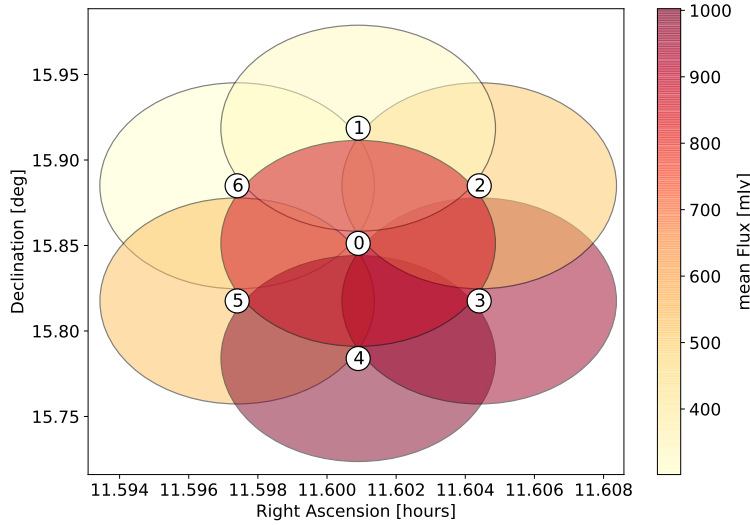
FIGURE 10.1 – Observation multi-faisceaux de B1133+16 avec le cœur de LOFAR en LBA. Les faisceaux sont fixes en ascension droite ainsi qu’en déclinaison, le recouvrement est de 0.06 degré correspondant au rayon à mi-hauteur des faisceaux à 60 MHz. Dans ce graphique les couleurs des faisceaux correspondent aux densités de flux moyen observées.
