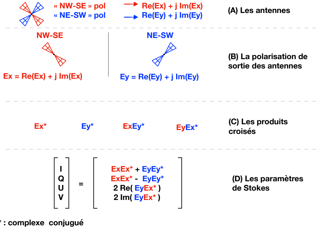
FIGURE 7.3 – Schéma de la polarisation de NenuFAR. Les signaux provenant des antennes NW-SE et NE-SW (A) sont numérisés dans les complexes \text{Re}(Ex) + \text{Im}(Ex) et \text{Re}(Ey) + \text{Im}(Ey) (B). Ensuite vient l'étape du calcul des produits croisés (C) afin de préparer le calcul des quatre paramètres de Stokes I, Q, U et V (D).
