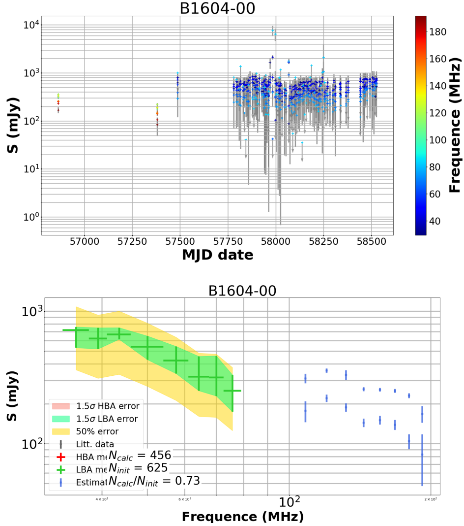
FIGURE D.10 – Suivi de B1604-00 par la station LOFAR FR606 en HBA et LBA. Dans le panneau supérieur : graphique du flux moyen en fonction du MJD (Modified Julian Date) et de la fréquence (échelle de couleurs sur la droite). Les points représentés avec des flèches grises sont des limites supérieures. Dans le panneau inférieur : spectre médian du même pulsar avec une erreur de 1.5\sigma (surface verte pour les LBA et rouge pour les HBA). L'erreur habituelle de 50 % est représentée par la surface jaune. Les crois bleus sont les observations utilisées pour la construction du spectre médian. Les crois grises sont les flux provenant de la littérature utilisées pour construire le spectre théorique (en gris) en loi de puissance provenant de Bilous et al. (2016).
