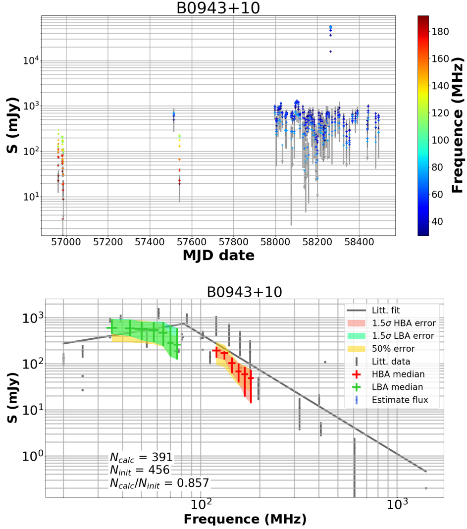
FIGURE D.7 – Suivi de B0943+10 par la station LOFAR FR606 en HBA et LBA. Dans le panneau supérieur : graphique du flux moyen en fonction du MJD (Modified Julian Date) et de la fréquence (échelle de couleurs sur la droite). Les points représentés avec des flèches grises sont des limites supérieures. Dans le panneau inférieur : spectre médian du même pulsar avec une erreur de 1.5\sigma (surface verte pour les LBA et rouge pour les HBA). L'erreur habituelle de 50 % est représentée par la surface jaune. Les crois bleus sont les observations utilisées pour la construction du spectre médian. Les crois grises sont les flux provenant de la littérature utilisées pour construire le spectre théorique (en gris) en loi de puissance provenant de Bilous et al. (2016).
