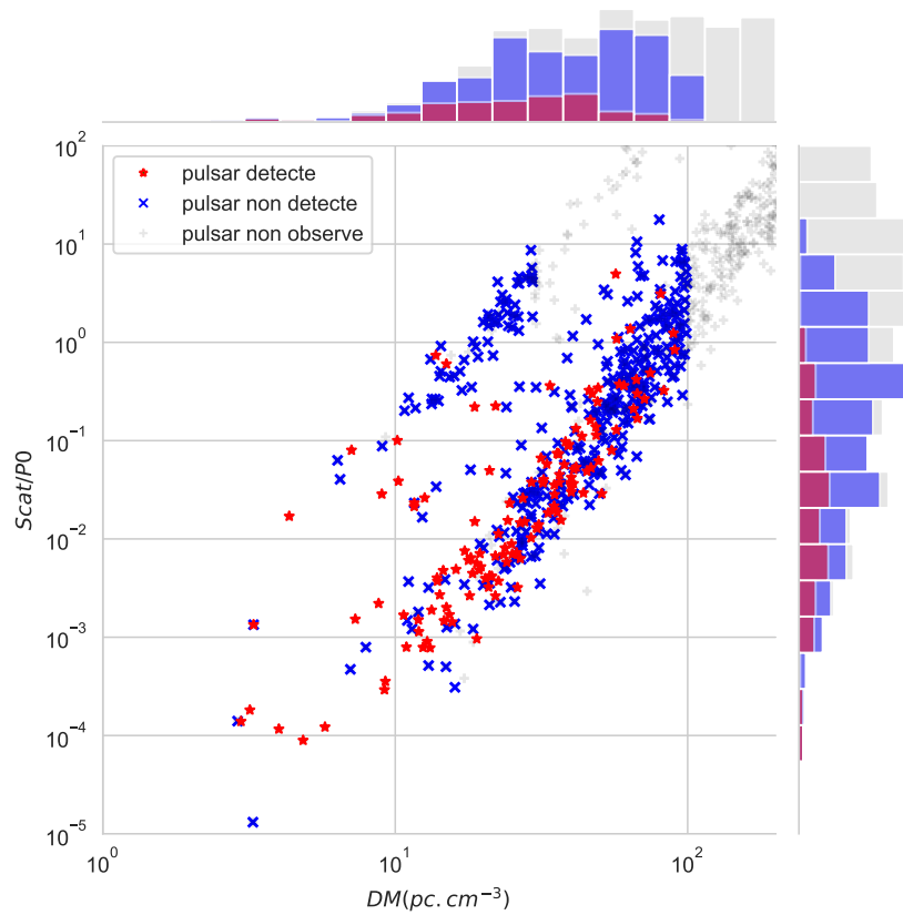
FIGURE 12.11 – Représentation de temps de multi-propagation divisé par la période ( \tau_{scat}/P0 ) en fonction du DM pour les pulsars du relevé de NenuFAR. Les étoiles rouges représentent les détections alors que les croix bleues sont les pulsars non détectés. Les croix grises représentent toute la population de pulsars du ciel observable de Nançay par NenuFAR sans les coupures en DM. La population des pulsars millisecondes est ici séparée des pulsars normaux par le facteur \frac{1}{P0} . Pour les deux axes de ce diagramme, il est affiché un histogramme des populations citées précédemment.
