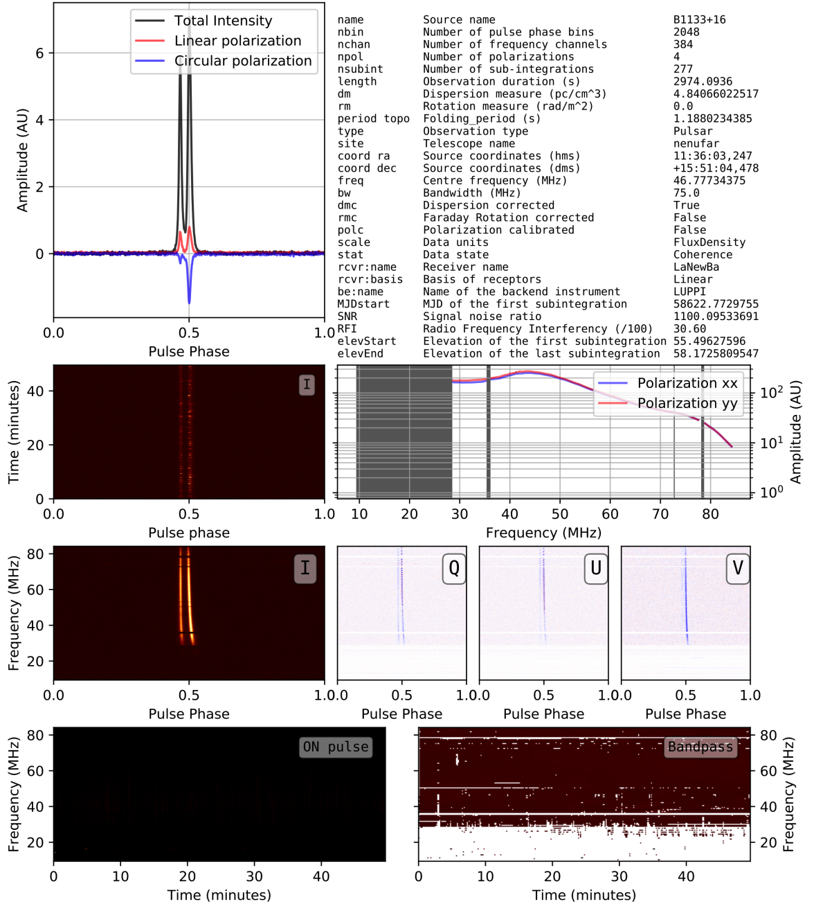
FIGURE 7.15 – Exemple de quicklook d’une observation du pulsar B1133+16 (intégrée sur 50 minutes) par NenuFAR en mode repliement (voir dans le chapitre 7.5.6). De gauche à droite et haut en bas : le profil du pulsar avec la polarisation linéaire ainsi que circulaire, les metadata de l’archive, le graphique phase/temps, la bande passante pour les deux polarisations (la zone grise entre 10 et 30 MHz masque d’importantes interférences qui sont habituelles entre 8 et 22 h LT), les quatre graphiques phase/fréquence pour les quatre paramètres de Stokes (I, Q, U et V), le spectre dynamique du pulsar (dans l’"ON pulse") et le spectre dynamique de la bande passante (dans l’"OFF pulse").
