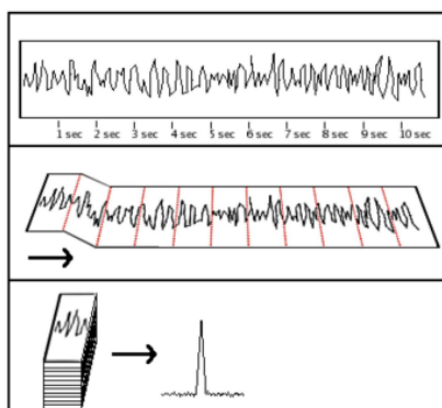
FIGURE 5.1 – Figure de Lynch (2013). Schéma de la méthode de repliement temporel. Le panneau du haut représente la série temporelle complète. Dans le panneau central les périodes du pulsar sont délimitées en rouge pour être empilées dans le dernier panneau pour augmenter le rapport signal-sur-bruit. Cependant, cette méthode demande de connaître la période du pulsar à l'avance.
