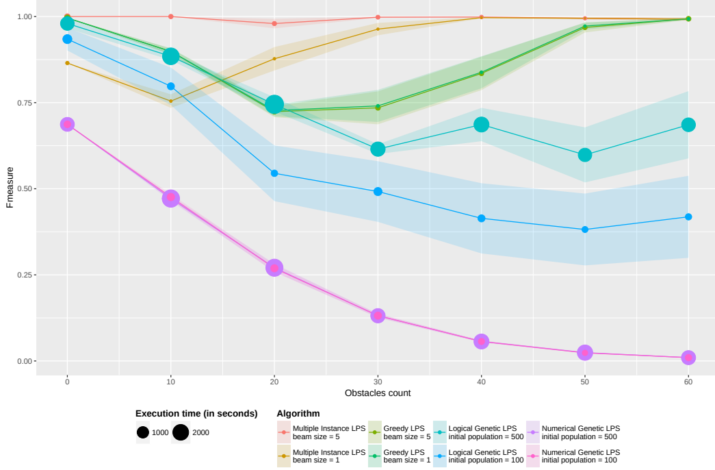
FIGURE 5.12 – Performance des algorithmes LPS pour la tâche d'apprentissage de Q_3^* .
