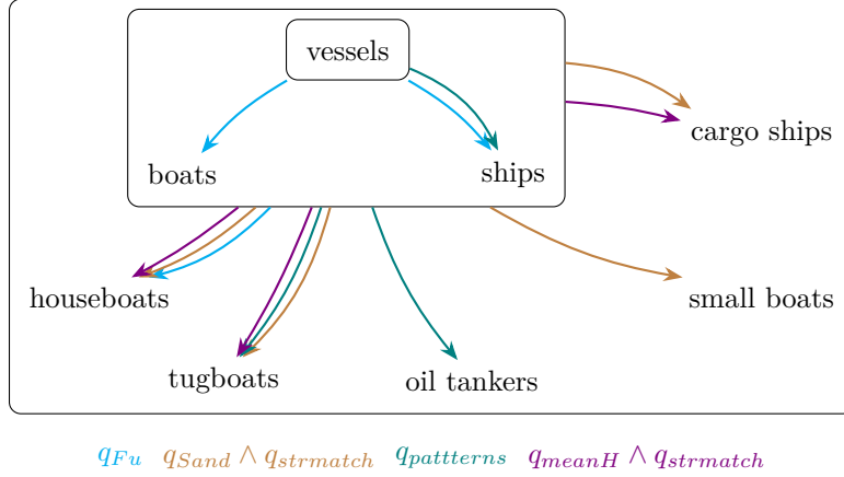
FIGURE 6.4 – Les différentes étapes de la propagation d’une relation sémantique. L’expansion démarre avec le singleton \{vessels\} .
