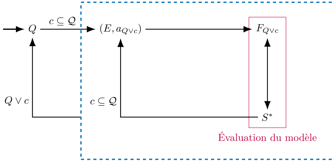
FIGURE 4.1 – L’algorithme LPS Glouton.
