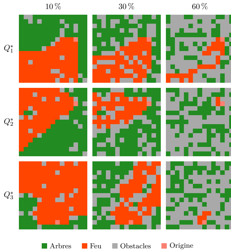
FIGURE 5.9 – Résultats de neuf simulations de propagation d'un feu de forêt. La première ligne illustre trois propagations modélisées par Q_1^* , la seconde par Q_2^* et la troisième par Q_3^* . Les grilles de la première colonne contiennent 10 % de cellules non-inflammables, la seconde 30 % et la troisième 60 %.
