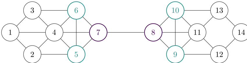
FIGURE 8.3 – Les nœuds 6, 5, 9 et 10 maximisent le critère d'intégration à la communauté \{7, 8\} .
