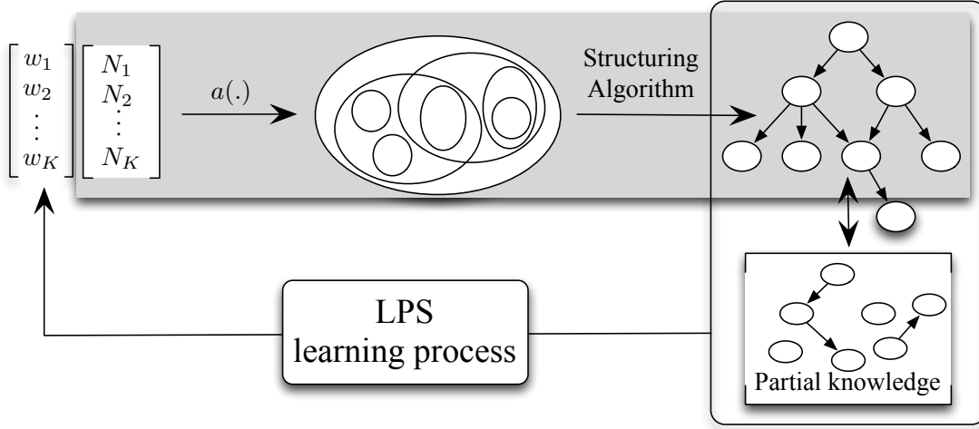
FIGURE 3.11 – Le processus d’apprentissage LPS génétique.
