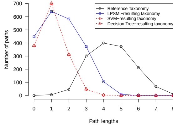
FIGURE 6.3 – Distribution de la taille des chemins sur les taxonomies du domaine food dérivées des modèles appris sur le domaine bread par différentes méthodes.
