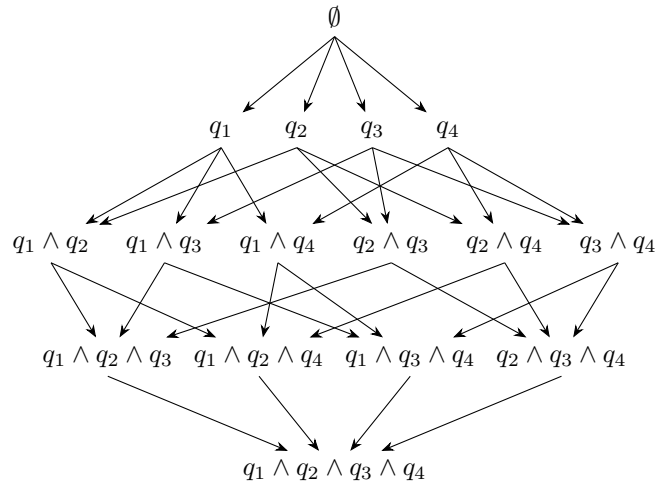
FIGURE 4.2 – Graphe de recherche de la meilleure clause conjonctive.
