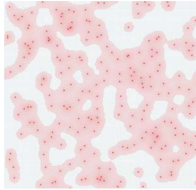
FIGURE 3.3 – Simulation de diffusion de la pollution aérienne à partir de plusieurs agents dispersés sur une grille torique.
