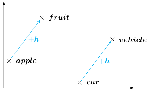
FIGURE 6.2 – L'existence du vecteur \mathbf{h} universel d'hyperonymie permettrait de passer de la représentation vectorielle d'un terme à celle de son hyperonyme direct.
