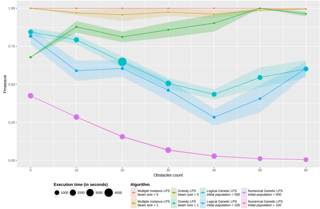
FIGURE 5.11 – Performance des algorithmes LPS pour la tâche d'apprentissage de Q_2^* .
