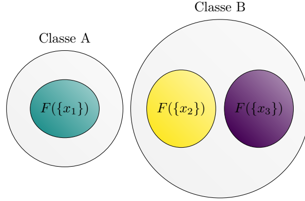
FIGURE 3.9 – Deux classes dont l’une inclut deux fermés minimaux. L’algorithme de partitionnement des k -moyennes cherchera trois groupes là où un algorithme hiérarchique permettra la fusion de F(\{x_2\}) et F(\{x_3\}) .
