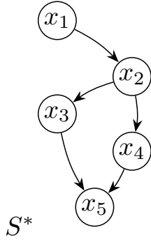
FIGURE 5.1 – Une fonction S^* de fermeture élémentaire cible et deux fonctions candidates de fermeture.
