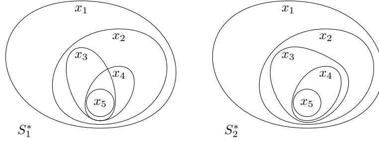
FIGURE 3.12 – Deux ensembles de fermés élémentaires S_1^* et S_2^* .
