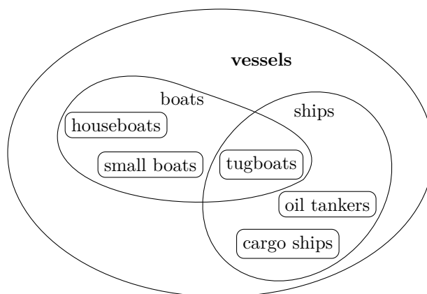
FIGURE 6.6 – Relations d’inclusion entre les fermés élémentaires d’un sous-ensemble de termes du domaine crafts . Un terme encadré représente un fermé élémentaire de taille 1 et, par conséquent, une feuille de la taxonomie lexicale.
