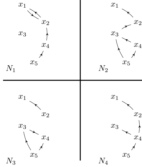
FIGURE 3.10 – Quatre relations de voisinages sur un ensemble E de cinq éléments. Une flèche depuis un élément x \in E vers un autre élément y \in E indique que y \in N(x) . Les relations réflexives sont masquées pour des raisons de lisibilité.
