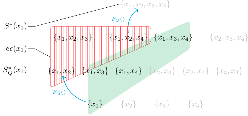
FIGURE 5.6 – Estimation des sacs positifs engendrés par x_1 et couverts par Q .
