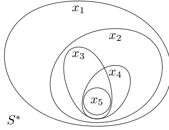
FIGURE 5.3 – Un ensemble de fermés élémentaires cibles.
