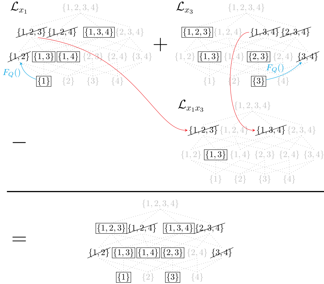
FIGURE 5.7 – Calcul du nombre de sacs positifs engendrés par la classe d'équivalence A_1 = \{x_1, x_3\} et couverts par une solution Q , avec E = \{x_1, x_2, x_3, x_4\} et S_1^* = E , F_Q(\{x_1\}) = \{x_1, x_2\} and F_Q(\{x_3\}) = \{x_3, x_4\} . La première ligne décrit la première étape du principe d'inclusion-exclusion et la seconde ligne décrit la deuxième étape. Un ensemble barré représente un sac rejeté, tandis qu'un ensemble encadré représente un sac couvert. Pour des questions de lisibilité, le « x » est masqué, l'ensemble \{1, 2\} correspond donc à \{x_1, x_2\} .
