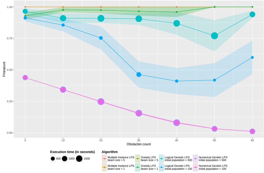
FIGURE 5.10 – Performance des algorithmes LPS pour la tâche d'apprentissage de Q_1^* .
