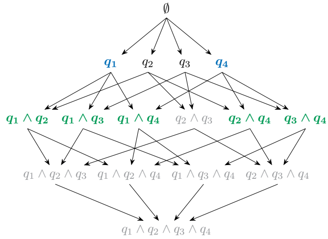
FIGURE 4.3 – Recherche avec un faisceau de taille 2 de la meilleure clause conjonctive. Les clauses bleues sont les clauses retenues lors de l'itération en cours et les clauses vertes sont les candidates de l'itération à venir.
