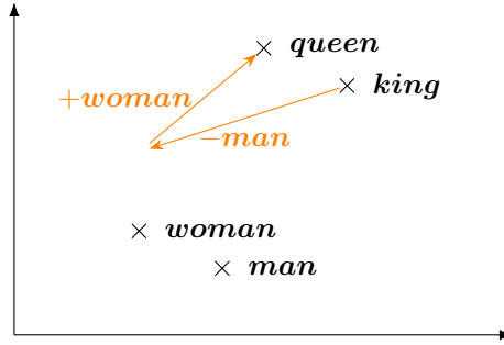
FIGURE 6.1 – Les propriétés sémantiques des termes « king », « queen », « man » et « woman » s'expriment par des opérations arithmétiques sur leurs représentations vectorielles.
