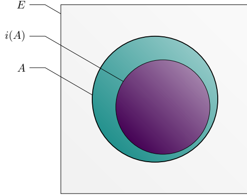
FIGURE 2.1 – L'opérateur d'intérieur permet de réduire un ensemble vers un autre, plus petit (au sens de l'inclusion).
