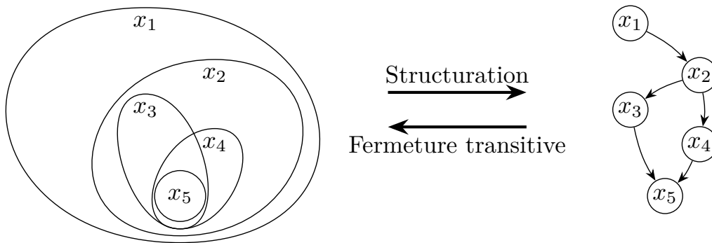
FIGURE 3.8 – Processus de structuration d'un ensemble de fermés élémentaires.
