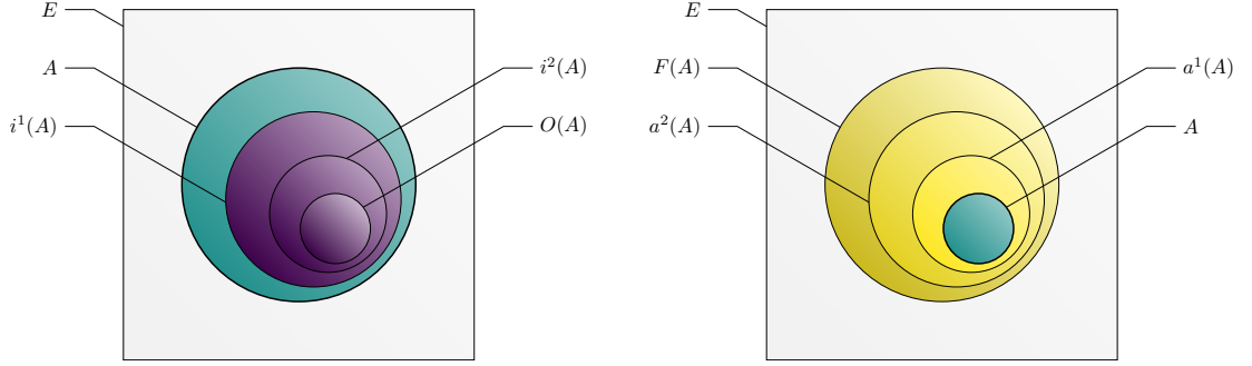
FIGURE 2.4 – Les opérateurs d’ouverture et de fermeture décrivent respectivement des processus de rétractation et d’expansion.
