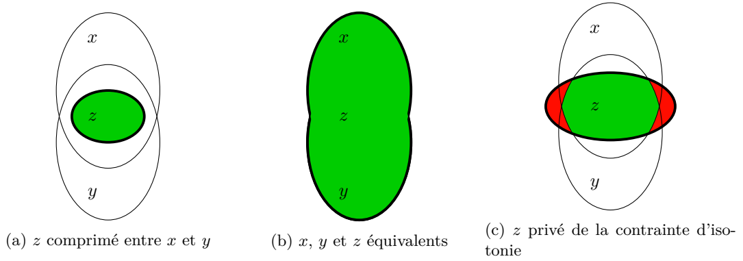
FIGURE 8.6 – Recouvrements autorisés par un espace prétopologique de type V. Le fermé de z est caractérisé par l'ellipse plus épaisse, les zones vertes et rouges représentent respectivement les sous-ensembles de F(\{z\}) autorisés et interdits dans une prétopologie de type V.
