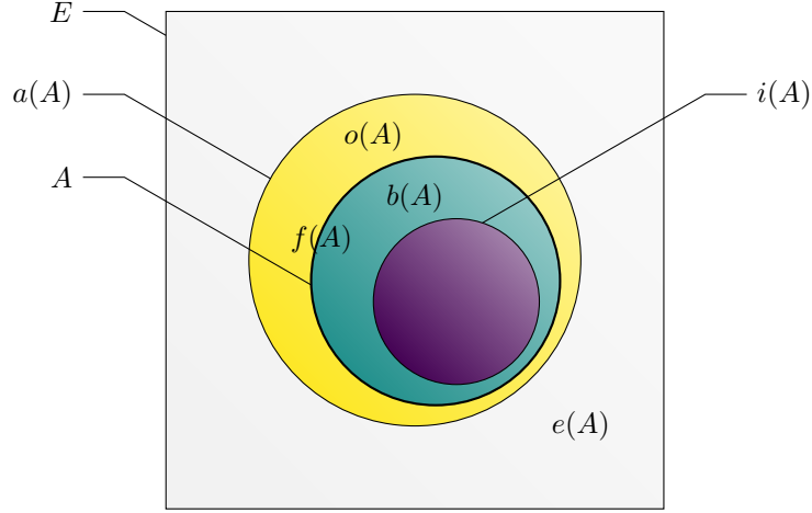
FIGURE 2.3 – Les opérateurs d’extérieur, de bord, d’orle et de frontière.
