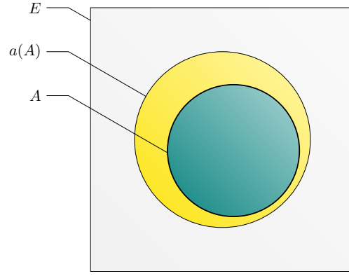
FIGURE 2.2 – L'opérateur d'adhérence permet d'étendre un ensemble vers un autre, plus grand (au sens de l'inclusion).
