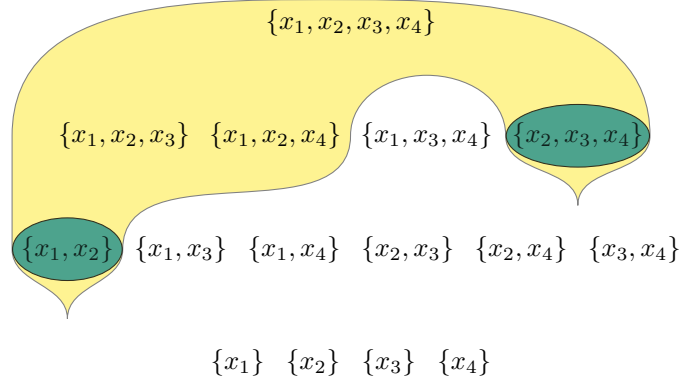
FIGURE 2.6 – En jaune, le préfiltre \mathcal{V}(x_2) et en vert une base de \mathcal{V}(x_2) . Dans cet exemple, la base est minimale.
