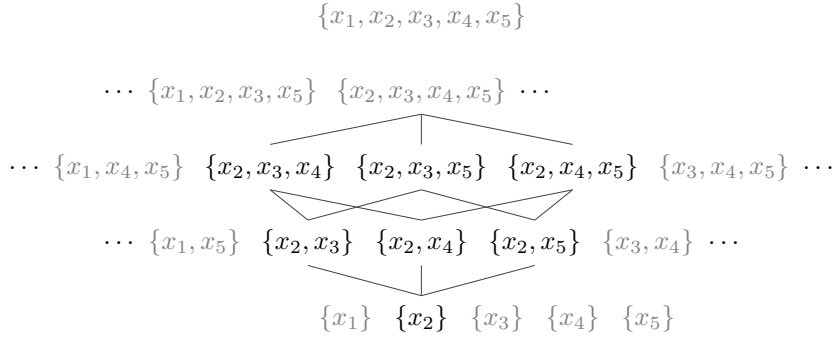
FIGURE 5.4 – Le sous-treillis \mathcal{L}[\{x_2\}, S^*(x_2)[ inclus dans le treillis Booléen sur E = \{x_1, x_2, x_3, x_4, x_5\} . Il y a une correspondance exacte entre ce sous-treillis et les sacs positifs engendrés par x_2 .
