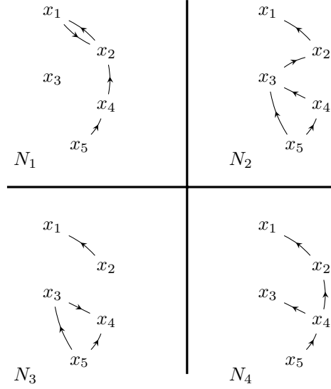
FIGURE 5.5 – Quatre relations de voisinages sur E = \{x_1, x_2, x_3, x_4, x_5\} .
