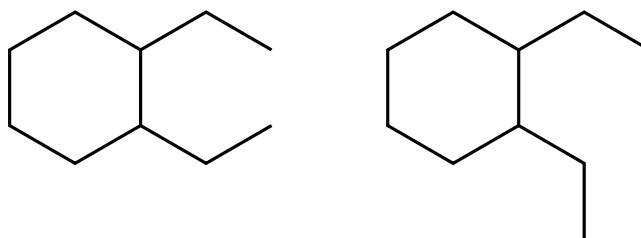
FIGURE 5.2 – Une même molécule sous différentes formes.
