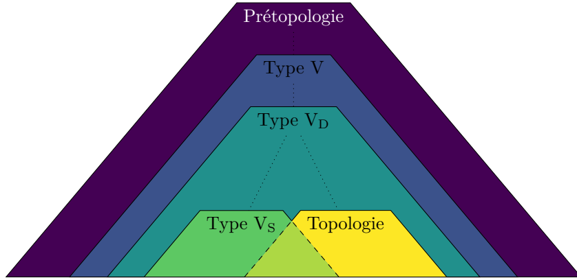
FIGURE 2.7 – Schéma d'inclusion des différentes familles d'espaces prétopologiques.
