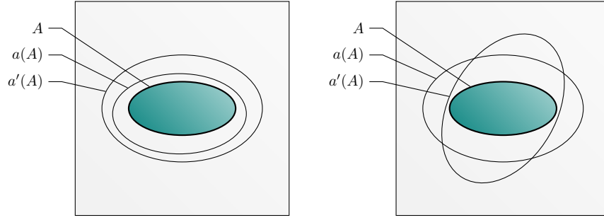
FIGURE 2.5 – À gauche, l'espace prétopologique (E, a) est plus fin que (E, a') . À droite, les deux espaces prétopologiques ne sont pas comparables.
