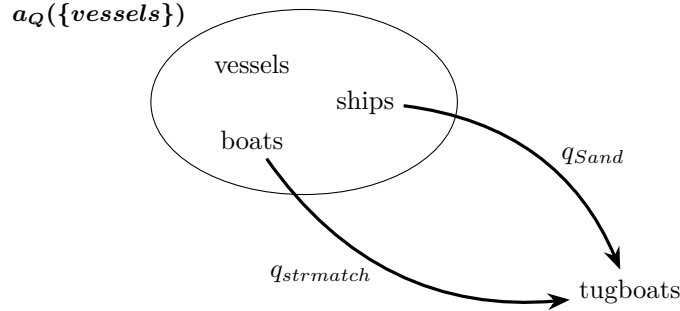
FIGURE 6.5 – Expansion de l’ensemble \{vessels, boats, ships\} vers le terme « tugboats » par la clause conjonctive q_{Sand} \wedge q_{strmatch} . Les deux littéraux capturent des relations entre différents termes : « ships » est un hyperonyme de « tugboats » selon q_{Sand} tandis que « boats » est un hyperonyme de « tugboats » selon q_{strmatch} .
