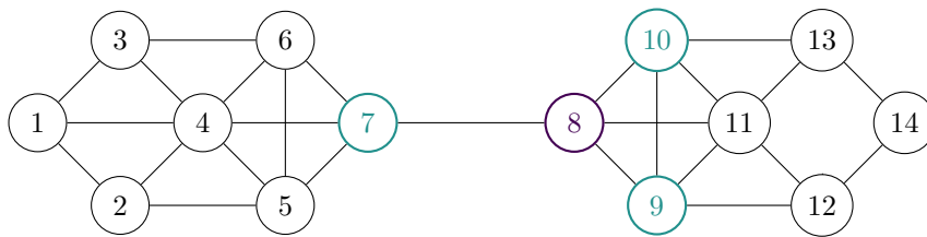
FIGURE 8.2 – Le nœud 8 est en bordure de communauté et les nœuds 7, 9 et 10 maximisent le critère d'intégration à la communauté \{8\} .
