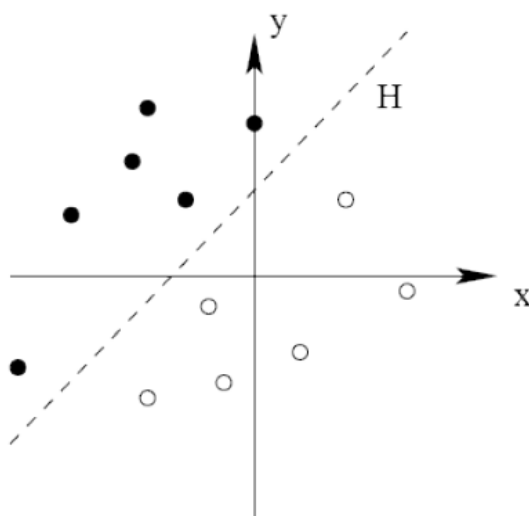
Figure 28: Illustration du fonctionnement d'un SVM – Extrait de Hasan & Boris (2006)
