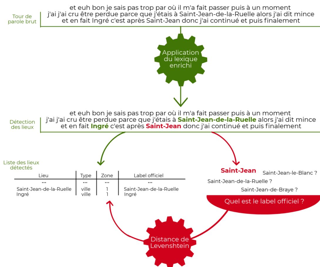
Figure 13 : Résolution de corréférence dans un tour de parole
