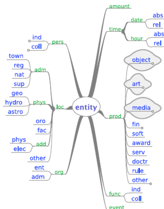
Figure 5 : Hiérarchie des entités dans la convention Quaero
