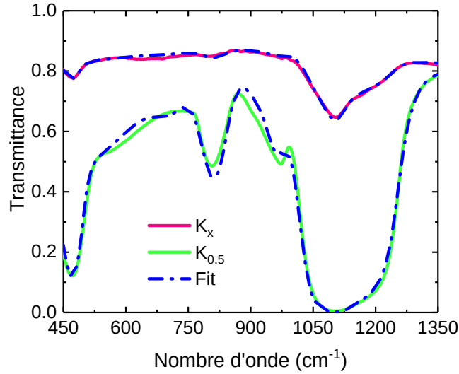
FIG. 3.6 – Mesures de transmission acquises sur des pastilles de KBr contenant 0.5% massique (courbe verte) et quelques traces notées x% (courbe rose) des nanopoudres de \text{SiO}_2 . Les courbes discontinues sont des ajustements des spectres réalisés avec l'expression de l'équation 3.1.
