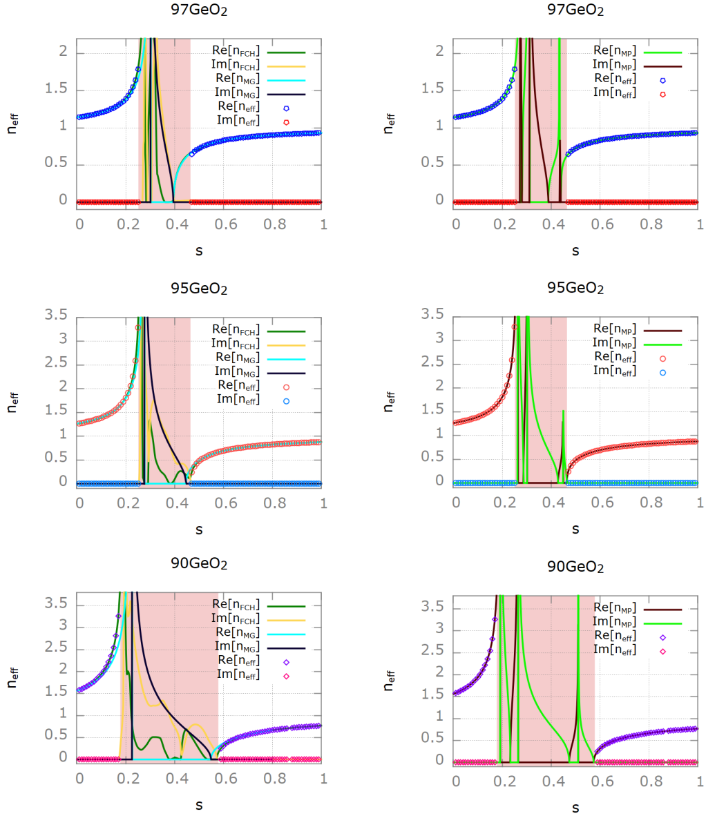
FIG. 3.30 – Indices de réfractions effectifs des systèmes 97\text{GeO}_2 , 95\text{GeO}_2 et 90\text{GeO}_2 , ajustés avec la méthode de FCH (à gauche) et la méthode MP (à droite). Comparaison avec les indices selon le modèle MG (à droite).
