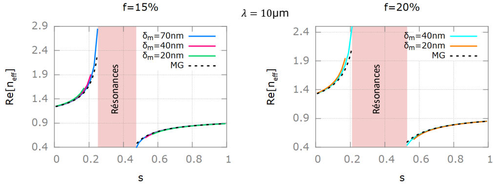
FIG. 2.13 – Partie réelle de l'indice de réfraction effectif des agglomérats de particules à des facteurs de remplissage 15% et 20%. Les calculs ont été réalisés dans les mêmes conditions que ceux de la figure 2.12 pour une longueur d'onde \lambda = 10 \mu\text{m} . Le comportement est similaire à la figure 2.12. Cela confirme la validité du régime quasi-statique à cette longueur d'onde.
