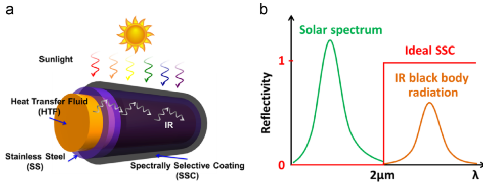
FIG. 1.2 – Revêtement spectralement sélectif (SSC) pour l'énergie solaire à concentration. (a) Schéma d'un absorbeur solaire constitué d'un tube en acier inoxydable (SS) revêtu du SSC. (b) Réflectance d'un SSC idéal. Dans le spectre solaire (courtes longueurs d'onde), la réflectance est nulle (absorbance égale à 100%) ; dans le domaine infrarouge, la réflectance est de 100% (émission nulle). Un tel SSC, considéré comme idéal, aura une absorptivité maximale pour l'énergie solaire et une perte de chaleur par rayonnement minimale [2].
