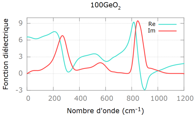
FIG. 3.22 – Parties réelle et imaginaire de la fonction diélectrique du verre 100GeO 2 .
