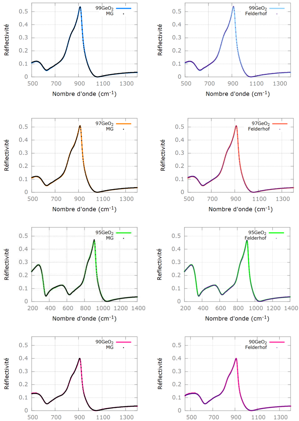
FIG. 3.23 – Réflectivités des verres ^{99}\text{GeO}_2 , ^{97}\text{GeO}_2 , ^{95}\text{GeO}_2 et ^{90}\text{GeO}_2 et leurs ajustements basés sur les modèles de MG et Felderhof. L'ajustement du ^{95}\text{GeO}_2 est réalisé sur une gamme spectrale plus large.
