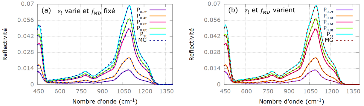
FIG. 3.14 – Ajustements de la réflectivité des pastilles obtenus à différentes pressions de compactage avec le modèle de MG. (a) les facteurs de remplissage f_{MD} (obtenus par la mesure de densité) sont fixés et \epsilon_i varie. (b) les deux quantités varient.
