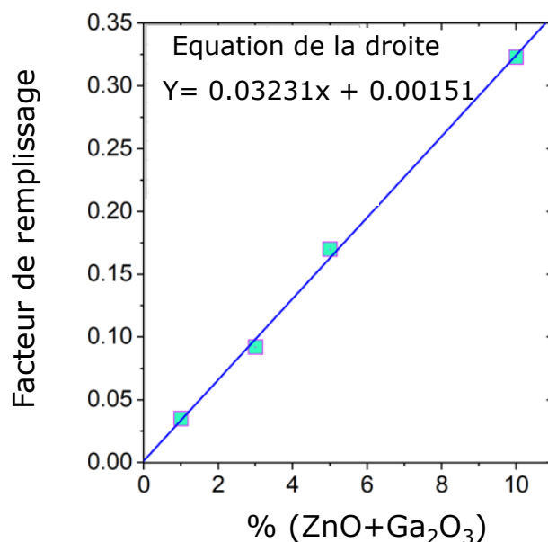
FIG. 3.24 – Facteurs de remplissage de Felderhof en fonction de %ZnGa 2 O 4 , ajustés par une droite de régression linéaire (bleu). Cette droite passant par l'origine indique le faible pourcentage de %ZnGa 2 O 4 dans la matrice GeO 2 .
