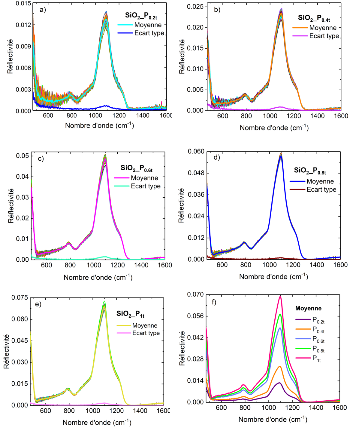
FIG. 3.4 – Réflectivités spéculaires des pastilles de \text{SiO}_2 amorphe compactées à différents niveaux de pression. Les lignes épaisses sont les moyennes et les écarts types d'un total de 25 spectres enregistrés pour chaque échantillon. (f) présente la moyenne des 25 spectres acquis pour chaque échantillon.
