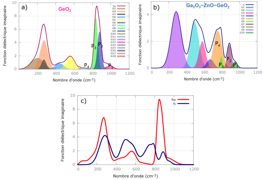
FIG. 3.25 – Parties imaginaires des fonctions diélectriques du verre de \text{GeO}_2 (a) et de la nanophase (b) ainsi que leurs décompositions en contributions gaussiennes.(c) Comparaison de (a) et (b).
