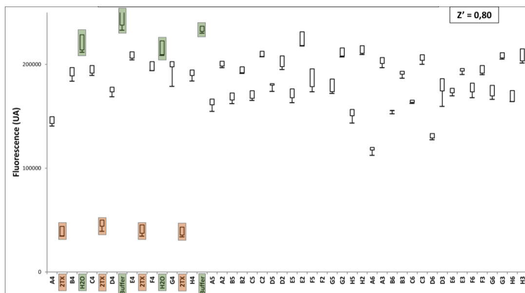
Figure 67 : Criblage « manuel » d'une plaque de GP sur LIFpg
