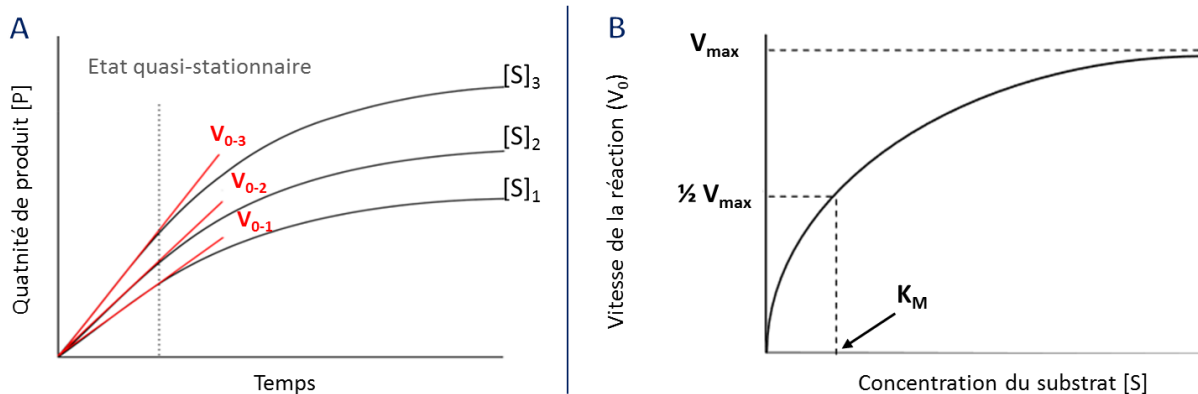
Figure 52 : Courbes théoriques pour l'évaluation de la cinétique d'une réaction enzymatique - A) Tracé de l'apparition du produit en fonction du temps, permettant avec la tangente à l'origine de déterminer les vitesses initiales. Chaque courbe correspond à une quantité de substrat différente et une quantité de protéine identique, suivant l'ordre [S]_3 > [S]_2 > [S]_1 . B) Tracé des valeurs des v_0 en fonction de la concentration du substrat associé. Avec l'équation de Michaelis-Menten, nous pouvons déterminer les valeurs de V_{max} et de K_M .
