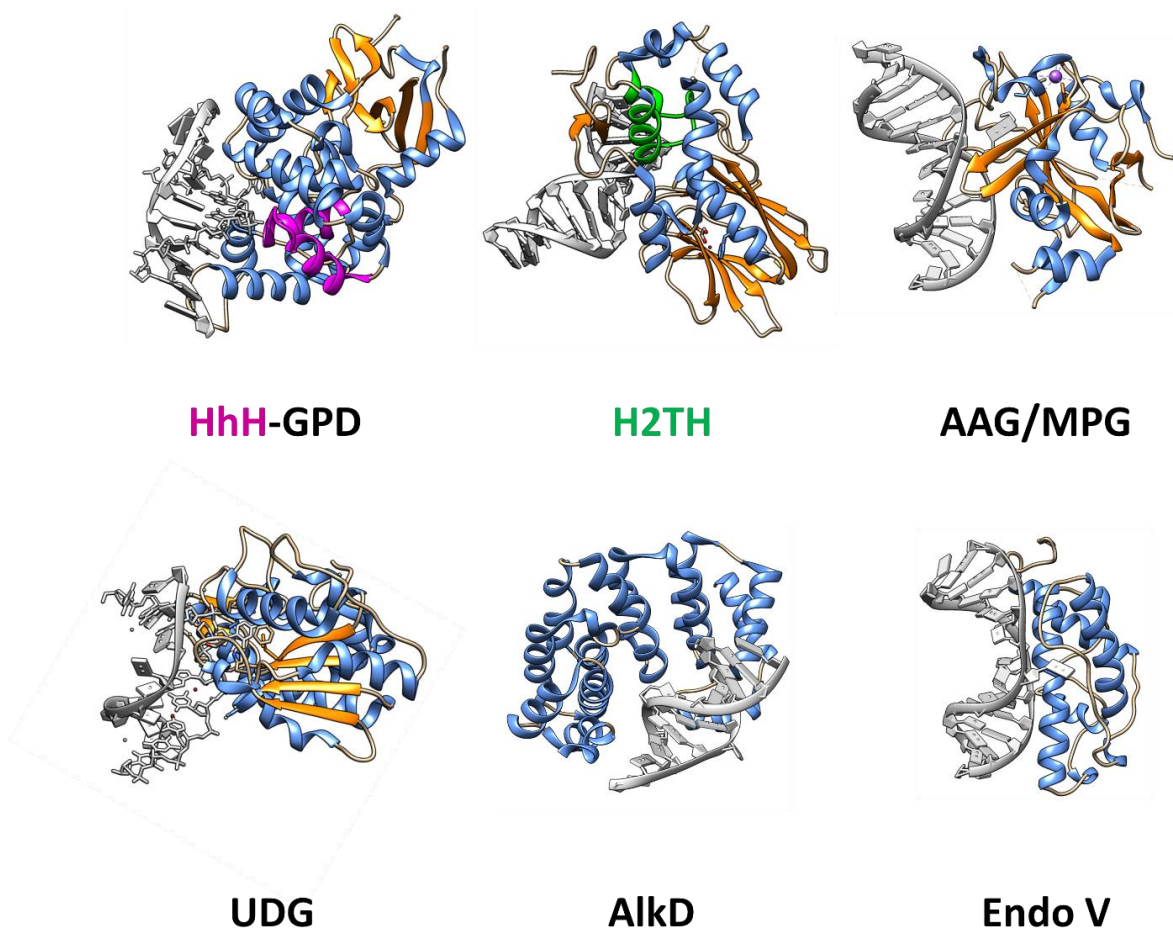
Figure 13 : Les différentes familles structurales des ADN glycosylases en interaction avec l'ADN - Les hélices \alpha sont colorées en bleu, les brins \beta en orange, le domaine HhH en magenta et H2TH en vert. Les modèles sont : HhH-GPD, OGG1 humaine (1YQK) ; H2TH, NEIL1 humaine (5ITT) ; AAG/MPG, AAG humaine (1EWN) ; UDG, UDG humaine (1EMH) ; ALK, AlkD de Bacillus cereus (3JXZ) ; Endo V, T4 pyrimidine dimer Endo V (1VAS).
