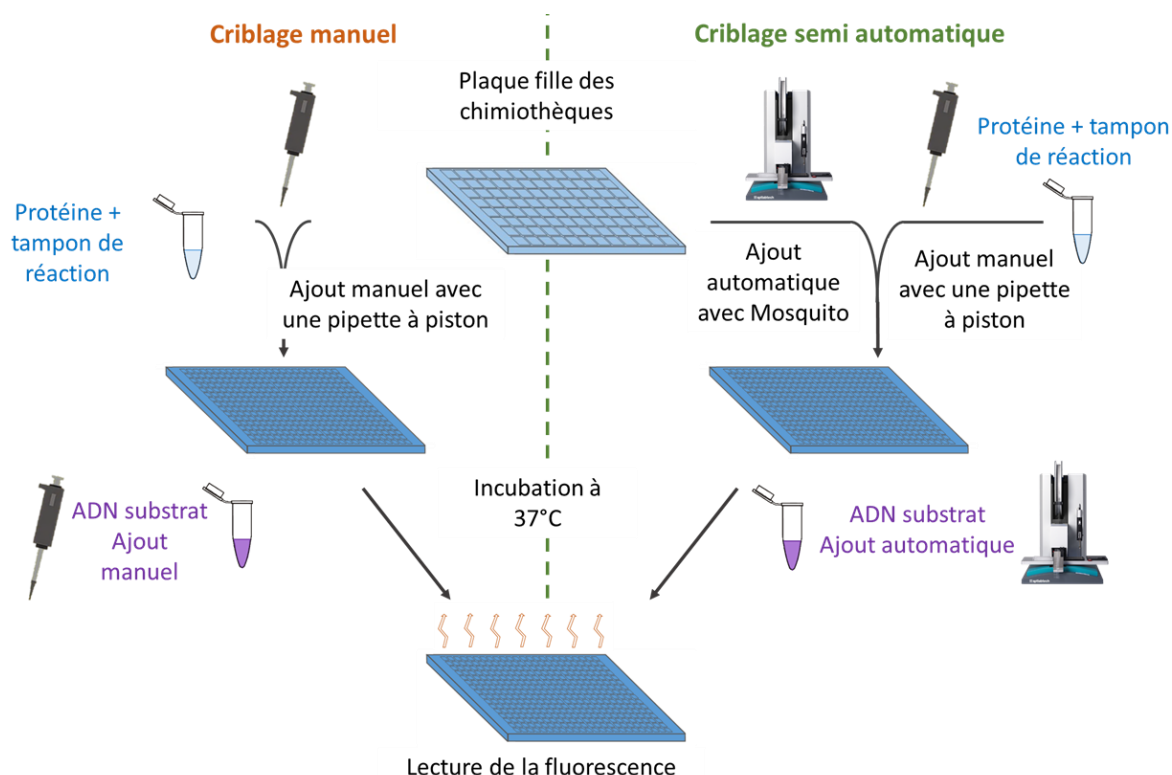
Figure 46 : Schéma du criblage primaire manuel ou semi-automatique
