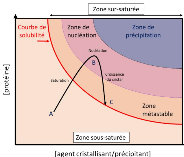
Figure 60 : Diagramme de phases à deux dimensions d'une macromolécule (adapté de Sauter et Giegé, 2010) [460] - A) Macromolécule soluble, B) Nucléation du cristal et C) Cristal final stable.
