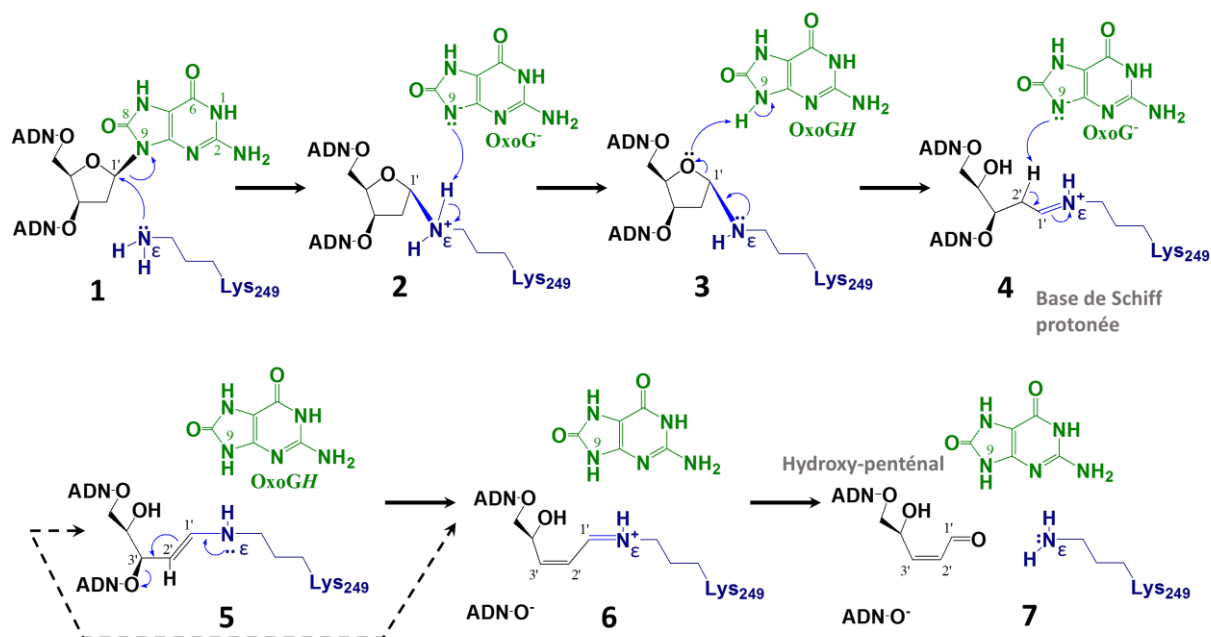
Figure 27 : Mécanisme suggéré de l'activité catalytique de hOGG1 sur la 8-oxoG par Fromme et al. , 2003 [312]
