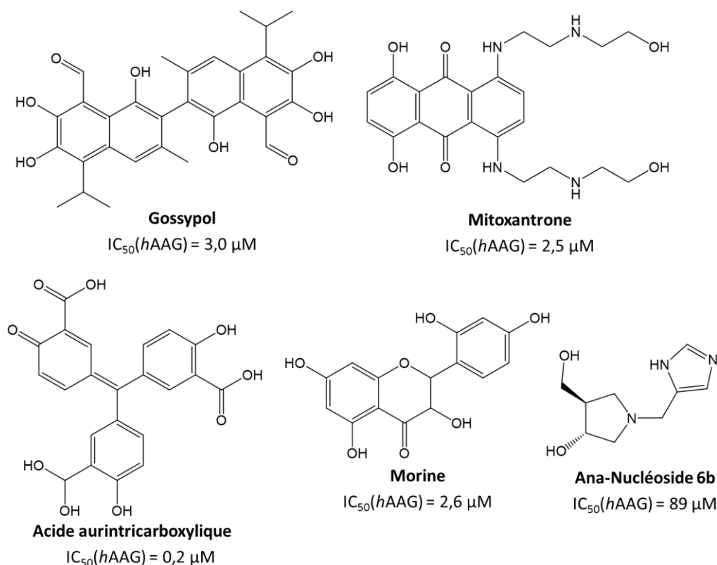
Figure 20 : Inhibiteurs de MPG
