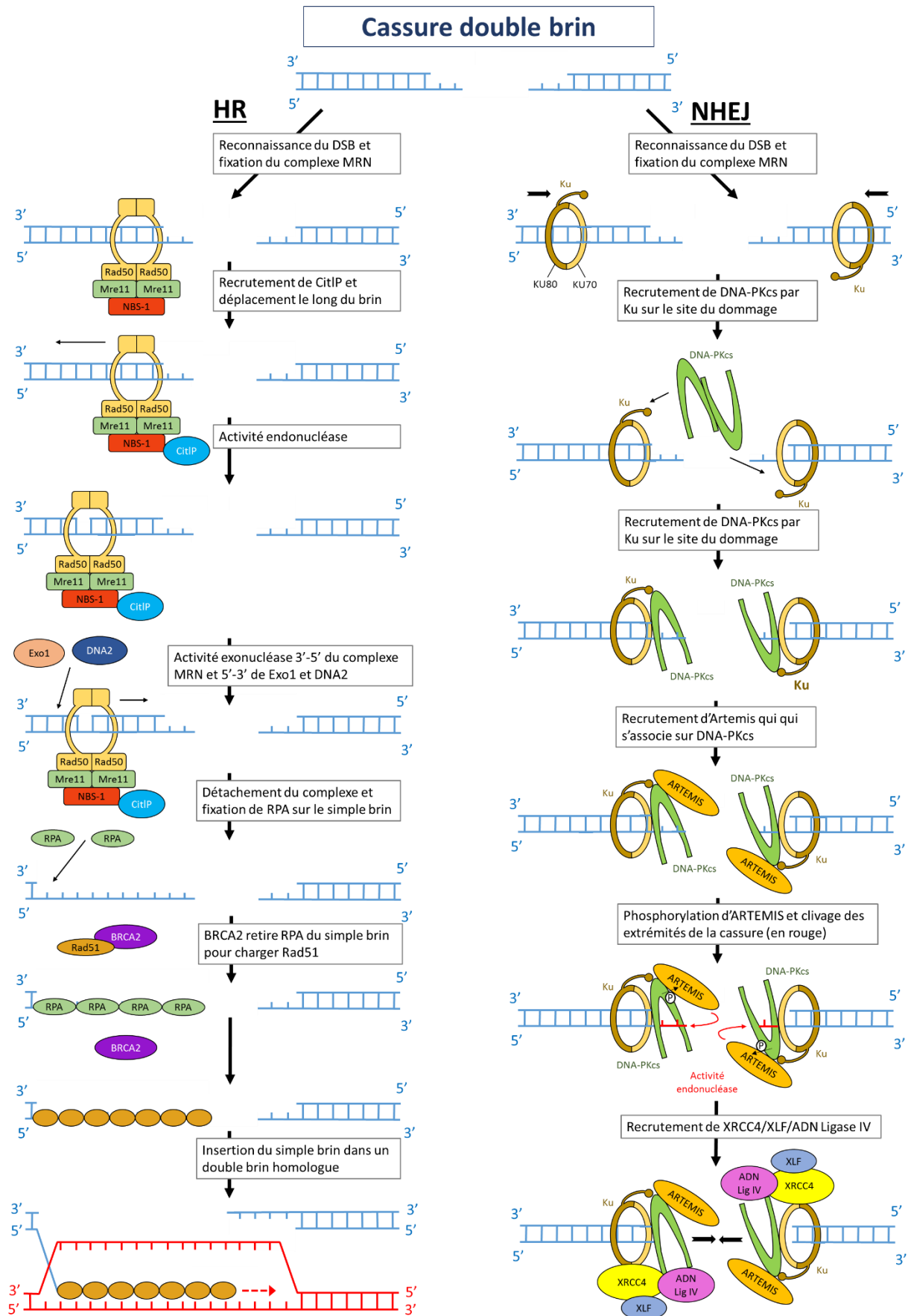
Figure 9 : Schéma du mécanisme général de HR et NHEJ
