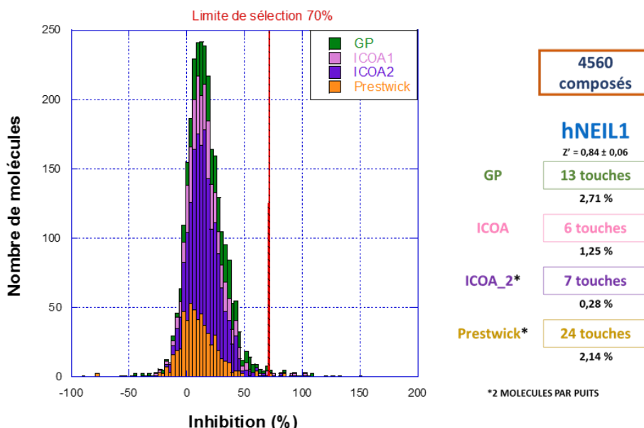
Figure 75 : Distribution du pourcentage d'inhibition des composés du criblage primaire sur hNEIL1
