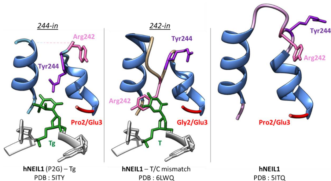
Figure 35 : Comparaison de la boucle LCL de hNEIL1 en conformation 244-in/242-in (conformations fermées) ou de la protéine non complexée à l'ADN (conformation ouverte)
