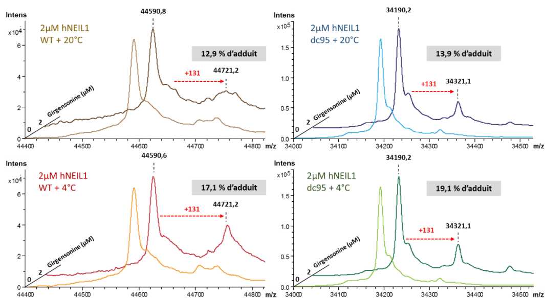
Figure 90 : Spectres déconvolués de l'adduit formé par la girsensonine en fonction de la température
