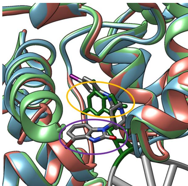
Figure 109 : Structure cristallographiques de hOGG1 seule (turquoise), complexée avec un duplex d'ADN contenant une 8-oxoG (saumon) ou avec TH5487 (vert pale) - L'ADN est en gris clair, la 8-oxoG en vert foncé, et TH5487 en gris foncé. La partie analogue de 8-oxoG de TH5487 est entourée d'un cercle violet, tandis que la 8-oxoG extrahélicale est entourée d'un cercle jaune. Les codes PDB sont 1KO9 (hOGG1 seule), 1EBM (hOGG1 complexée à l'ADN) et 6RLW (hOGG1 avec TH5487).
