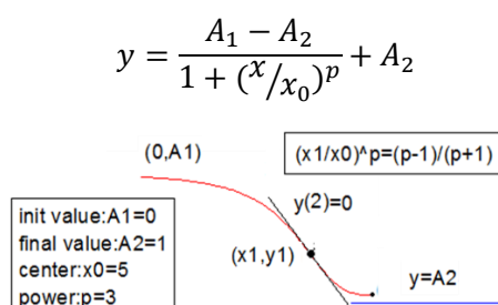
Equation 3 : Equation du « fitting » des courbes d'inhibition des inhibiteurs et calcul d'IC 50 - A 1 étant la valeur en ordonnée initiale (0 % d'activité dans notre cas), A 2 la valeur finale attendue (100 % d'activité). La valeur d'IC 50 est donc la valeur en ordonnée pour x= (A 1 +A 2 )/2 (50 % dans le cas d'un IC 50 , mais le principe est le même pour les IC 20 ou IC 80 ). p représente le coefficient de Hill.
