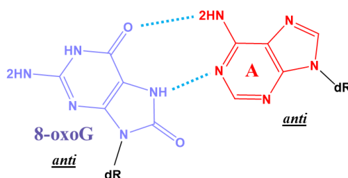
Figure 6 : Propriétés d'appariements de type Hoogsteen de la 8-oxoG avec une adénine - Les liaisons hydrogène sont indiquées en bleu clair.
