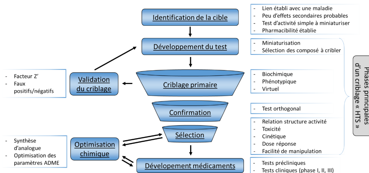
Figure 38 : Schéma des étapes principales d'un criblage classique pour le développement d'un médicament
