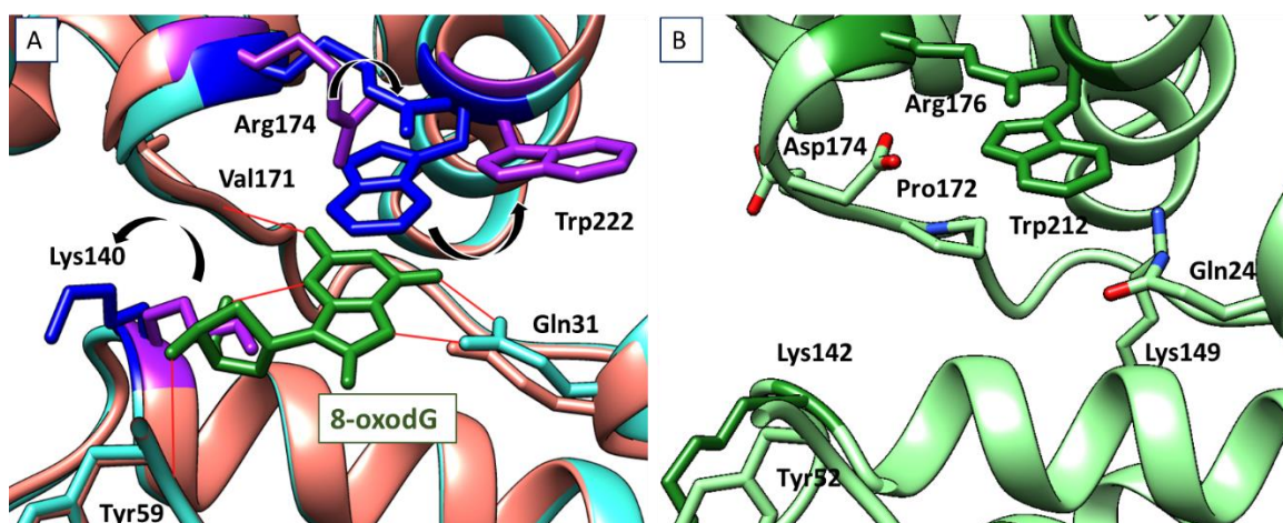
Figure 119 : Changement conformationnel suite à la complexation de PaeAGOG avec la 8-oxodG - A) Changement conformationnel entre la poche du site actif de PaeAGOG seul (en saumon, PDB 1XQO) et PaeAGOG complexée (en bleu clair, PDB 1XQP) à la 8-oxodG (en vert foncé). Les résidus dont la position change sont indiqués en bleu foncé (enzyme complexée) et en violet (enzyme libre), et la direction du changement est indiquée par des flèches noires. B) Site actif de l'enzyme PabAGOG, avec les acides aminés très bien conservés par rapport à PaeAGOG.
