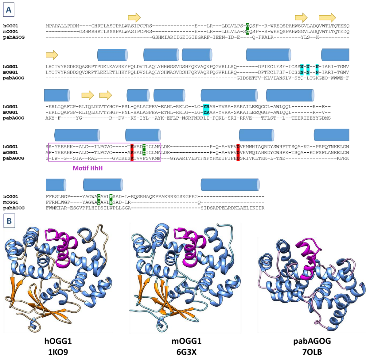
Figure 116 : Comparaison structurale entre hOGG1, PabAGOG et mOGG1 - A) Alignement de séquence de PabAGOG, mOGG1 et hOGG1 basé sur la structure de ces protéines. Les hélices \alpha conservées sont indiquées en bleu foncé. Les brins \beta conservés chez mOGG1 et hOGG1 sont représentés par des flèches orange. Les résidus catalytiques sont indiqués sur fond rouge, les résidus d'intercalation en cyan, et ceux interagissant avec la base opposée en vert. B) Structure cristallographique de ces enzymes. Les hélices \alpha sont colorées en bleu, les brins \beta en orange et le domaine HhH en magenta. Les PDB utilisées pour hOGG1, mOGG1 et PabAGOG sont indiquées sur la figure.
