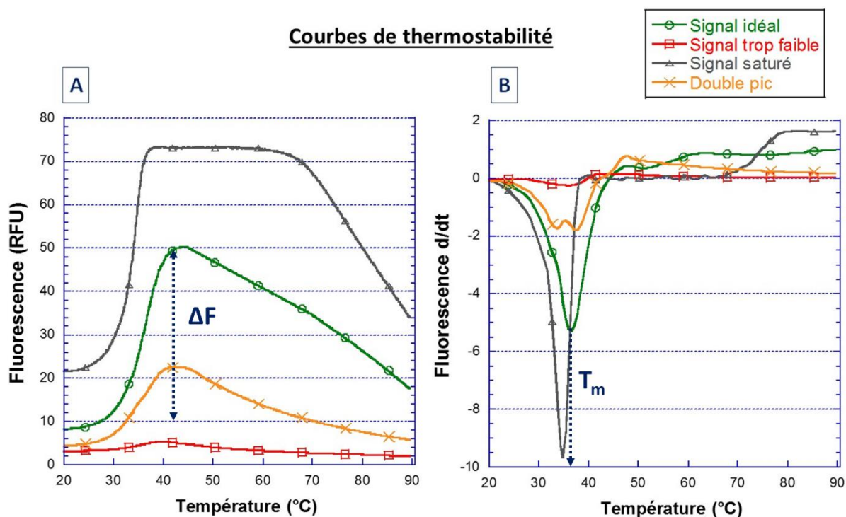
Figure 55 : Courbe de TSA théorique et évaluation de la température de fusion d'une protéine - A) La fluorescence produite par le Sypro Orange est lue en fonction de la température de l'échantillon. La différence entre le signal minimal et le maximum de fluorescence est noté \Delta F . 4 courbes sont indiquées : une courbe avec un \Delta F trop faible pour une lecture correcte en rouge, une courbe dont la fluorescence est trop élevée et fait saturer le lecteur en noir, et une courbe en orange dont le sommet est mal formé et possède deux maxima différents. Enfin en vert est représentée une courbe idéale. B) Sur le graphique est indiquée la dérivée de chacune des 4 courbes précédentes. Le minimum obtenu permet en abscisse d'obtenir la valeur du T_m .
