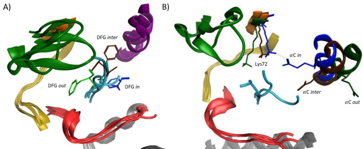
Figure 21 : Différentes conformations pouvant être prises par le motif DFG (A) et par l'hélice \alpha C (B). La phénylalanine du motif DFG et la glutamine de l'hélice \alpha C sont coloriées en bleu dans leur position « in », en vert dans leur position « out » et en marron dans leur position intermédiaire. D'après la thèse de Colin Bournez 2 .
