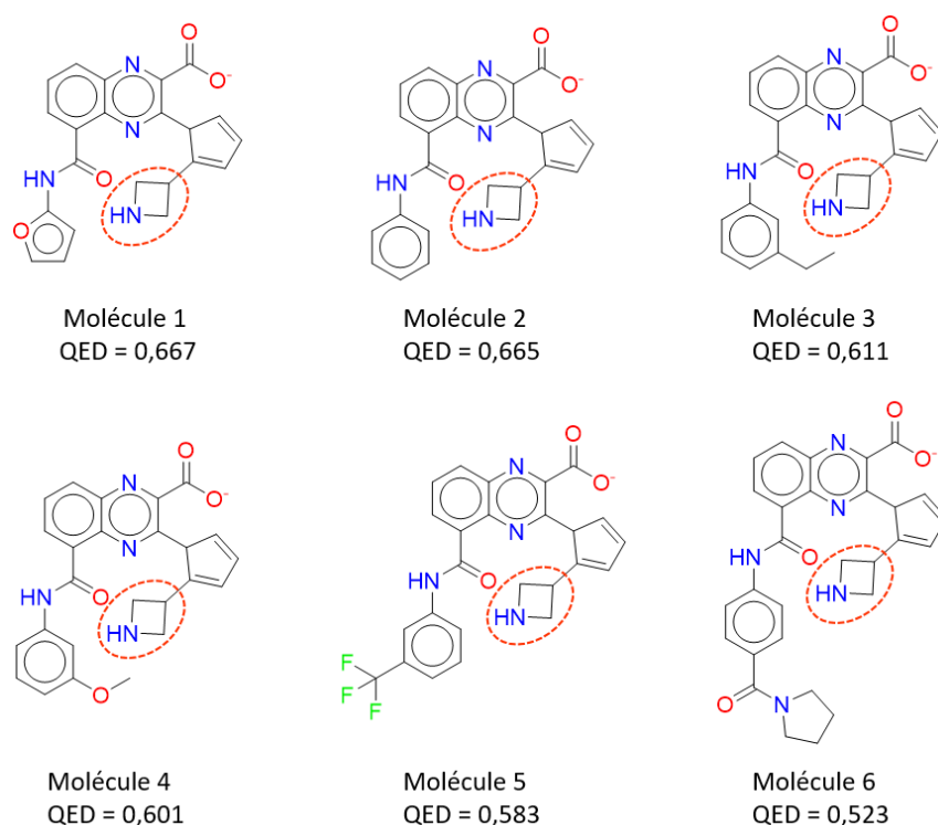
Figure 76 : Structures 2D des 6 molécules du groupe 1 ayant un score QED > 0,5. Le groupement azétidine qui pose problème pour la synthèse des molécules est entouré en rouge.
