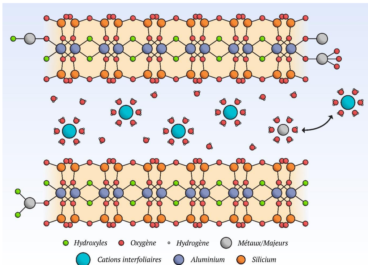
Figure 1.14. Mécanismes de sorption (adsorption, échange d'ions) prenant place sur une argile de type smectite.
