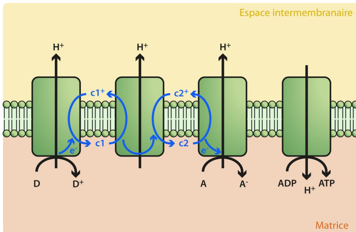
Figure 1.15. Représentation simplifiée d'une chaîne respiratoire générant de l'ATP. D = Donneur d' e^- , A = Accepteur d' e^- , c = coenzyme. (Mertz, inspiré de Jin and Bethke, 2002).
