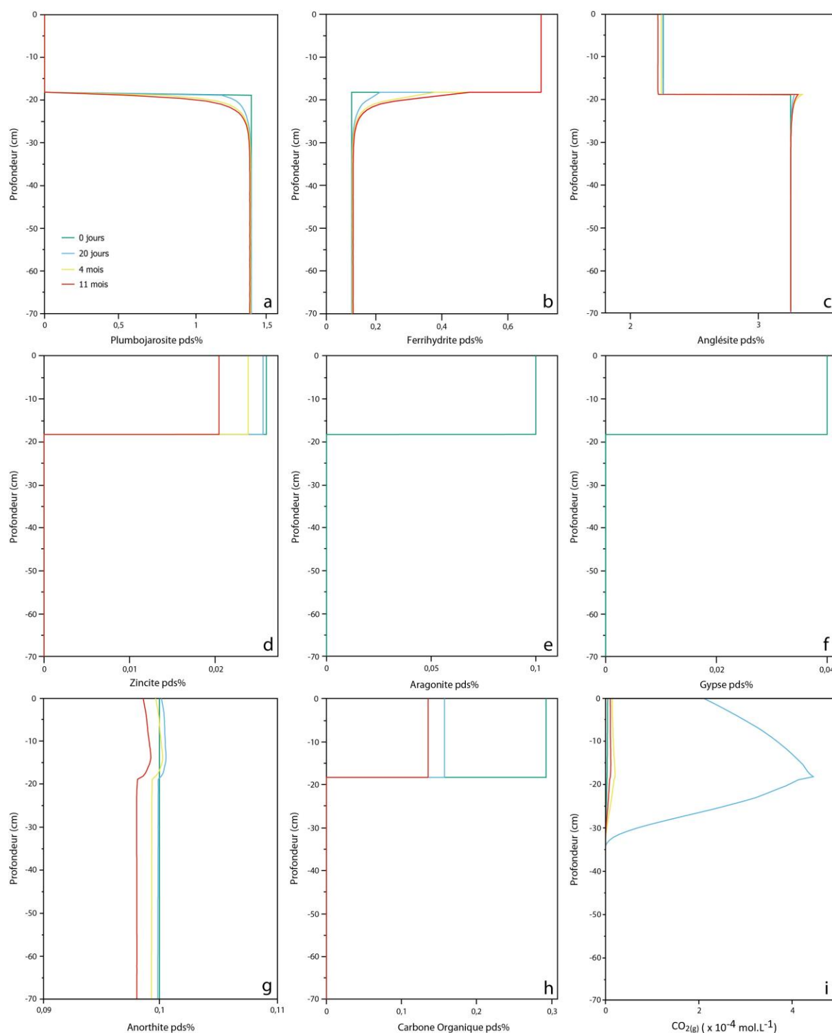
Figure 4.6. Evolution suivant la profondeur de la quantité des phases minérales/organiques et de la concentration en \text{CO}_2(\text{g}) présentes dans les tailings : plumbojarosite (a), ferrihydrite (b), anglésite (c), zincite (d), aragonite (e), gypse (f), anorthite (g), carbone organique (h) et concentration en \text{CO}_2(\text{g}) (i).
