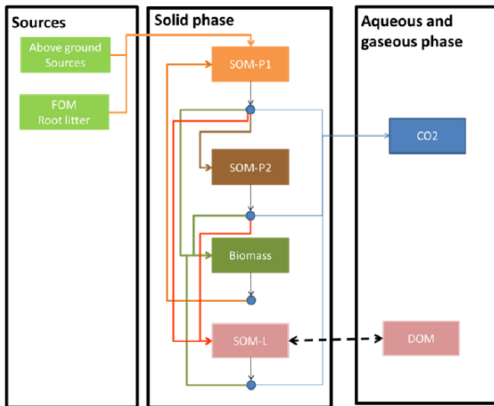
Figure 1.11 : Dynamique de la MO dans les sols. Les lignes orange indiquent la décomposition en matières organiques du sol facilement décomposable (SOM-P1), les lignes marron
