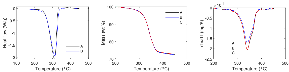
(b) 50 wt%.
