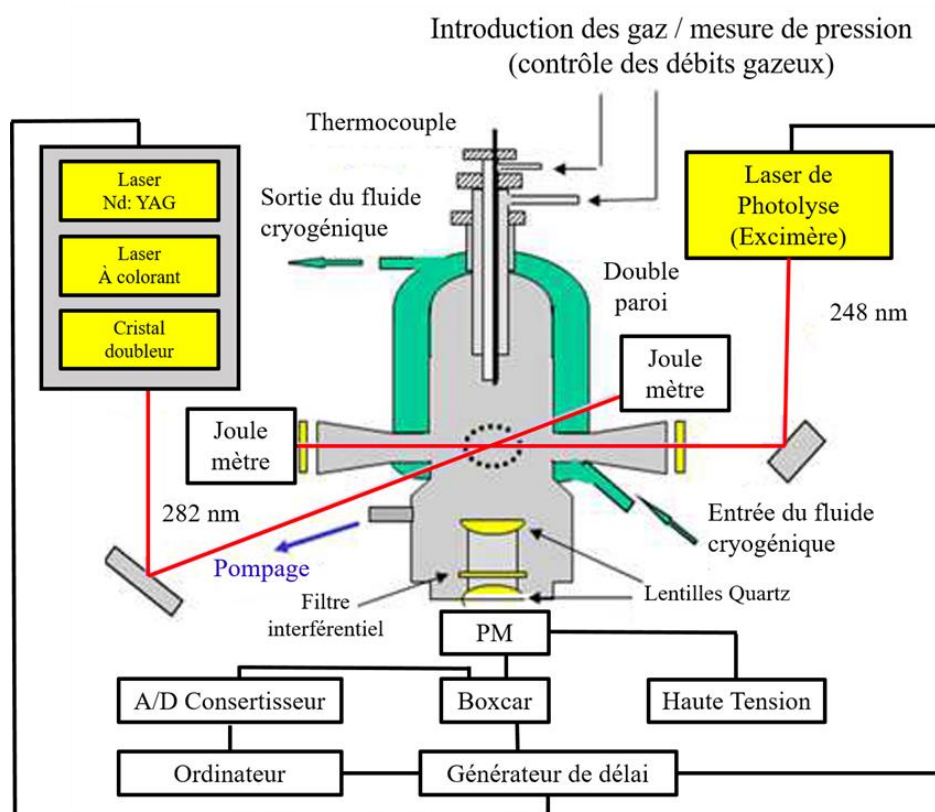
Figure 2-4 Schéma du dispositif expérimental de PLP-FIL
