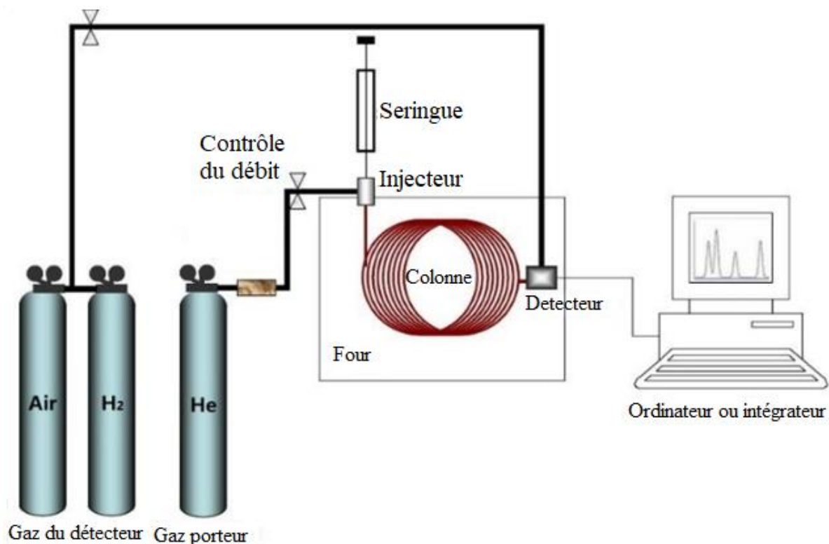
Figure 2-6 Schéma du système de la chromatographie en phase gazeuse avec détection FID
