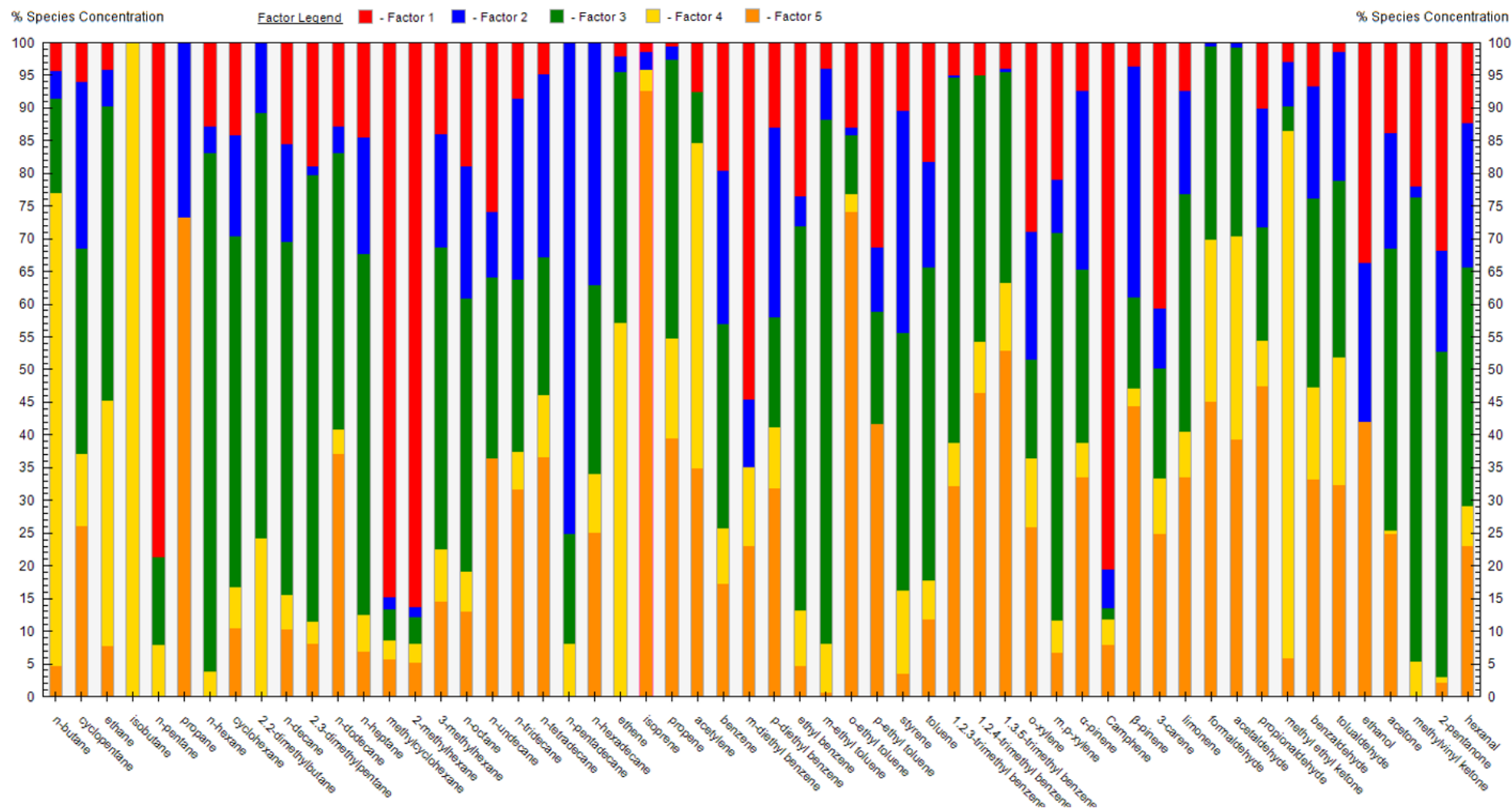
Figure 5-6 Profils de sources résolus à partir du modèle de factorisation matricielle positive (PMF).
