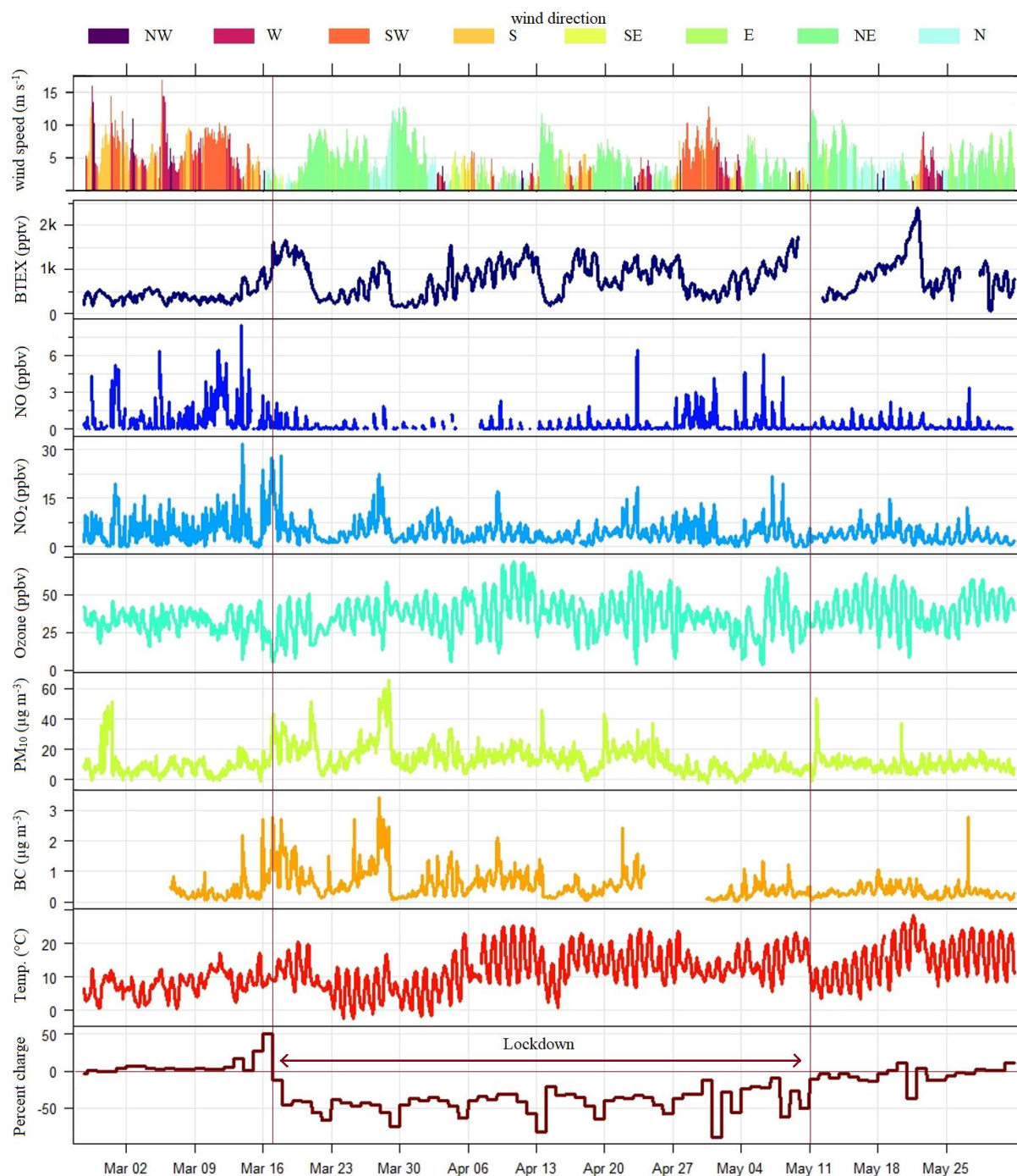
Figure 4-2 Série temporelle des valeurs de BTEX (pptv), NO (ppbv), NO 2 (ppbv), ozone (ppbv), PM 10 ( \mu\text{g m}^{-3} ), Black Carbon ( \mu\text{g m}^{-3} ) et température ( ^{\circ}\text{C} ) à Orléans pendant la période étudiée, avec le "pourcentage de variation dans les déplacements quotidiens vers les épiceries et les pharmacies", et la paramètres météorologiques (vitesse du vent en \text{m s}^{-1} , direction du vent avec un code couleur).
