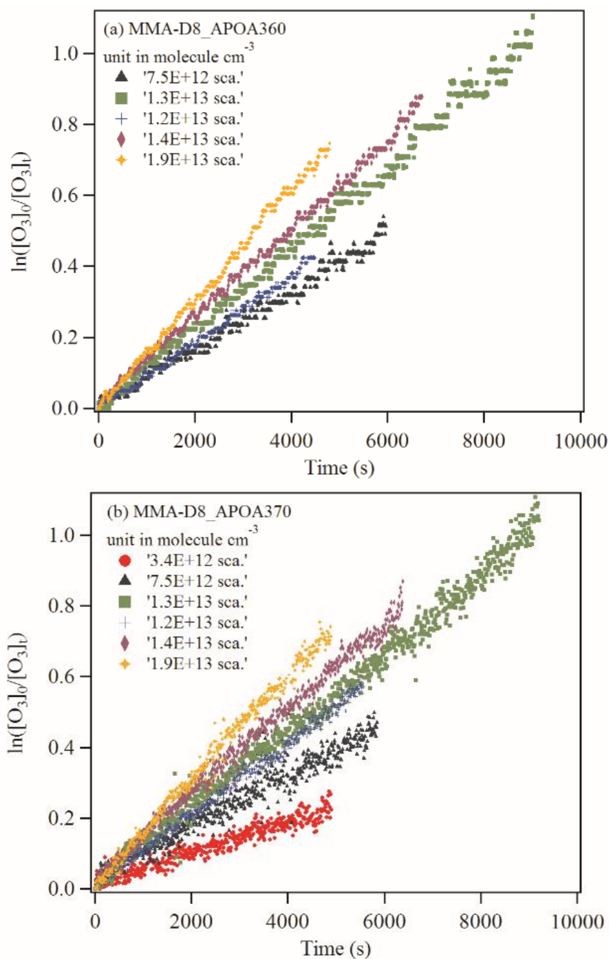
Figure 3-12 Exemple de graphiques de la consommation d' O_3 en fonction du temps de réaction en présence de différentes concentrations de MMA-D8 en utilisant deux types de moniteur de O_3 (APOA360 et APOA370). Note : CO sca. = expériences en présence de CO comme piègeur.
