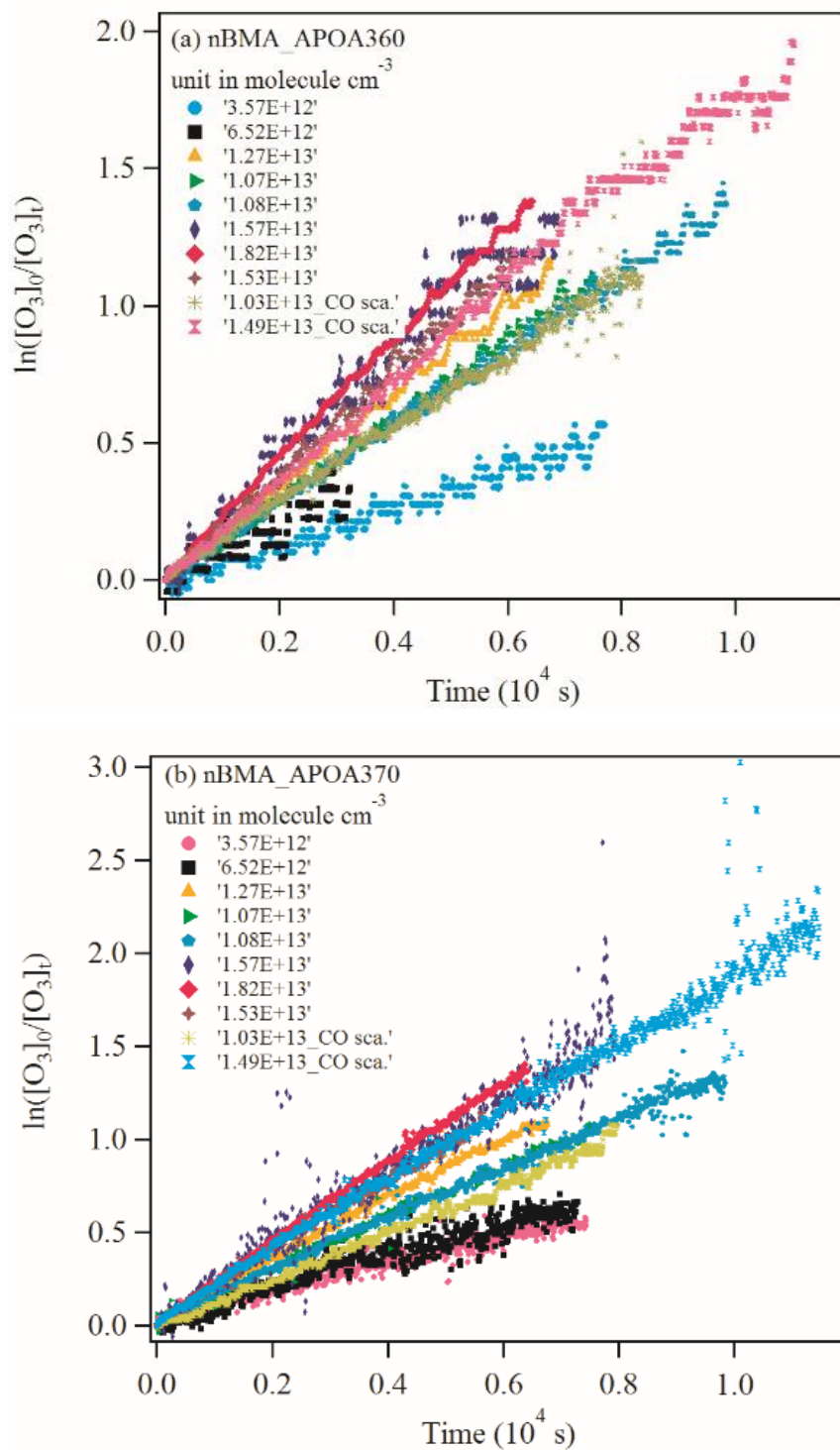
Figure 3-10 Exemple de graphiques de la consommation d' O_3 en fonction du temps de réaction en présence de différentes concentrations de nBMA en utilisant deux types de moniteur de O_3 (APOA360 et APOA370). Note : CO sca. = expériences en présence de CO comme piègeur.
