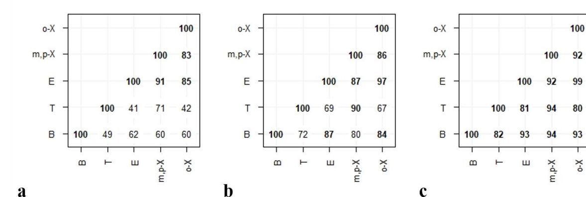
Figure 4-5 Coefficients de corrélation en pourcentage entre le benzène, le toluène, l'éthylbenzène, le m,p-Xylène et le o-Xylène (a) avant, (b) pendant et (c) après le confinement.
