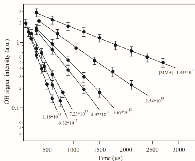
Figure 3-1 Profils typiques du signal de OH en fonction du temps de réaction pour différentes concentrations de MMA (unité en molécule \text{cm}^{-3} ) à T = (297 \pm 1) \text{ K} .
