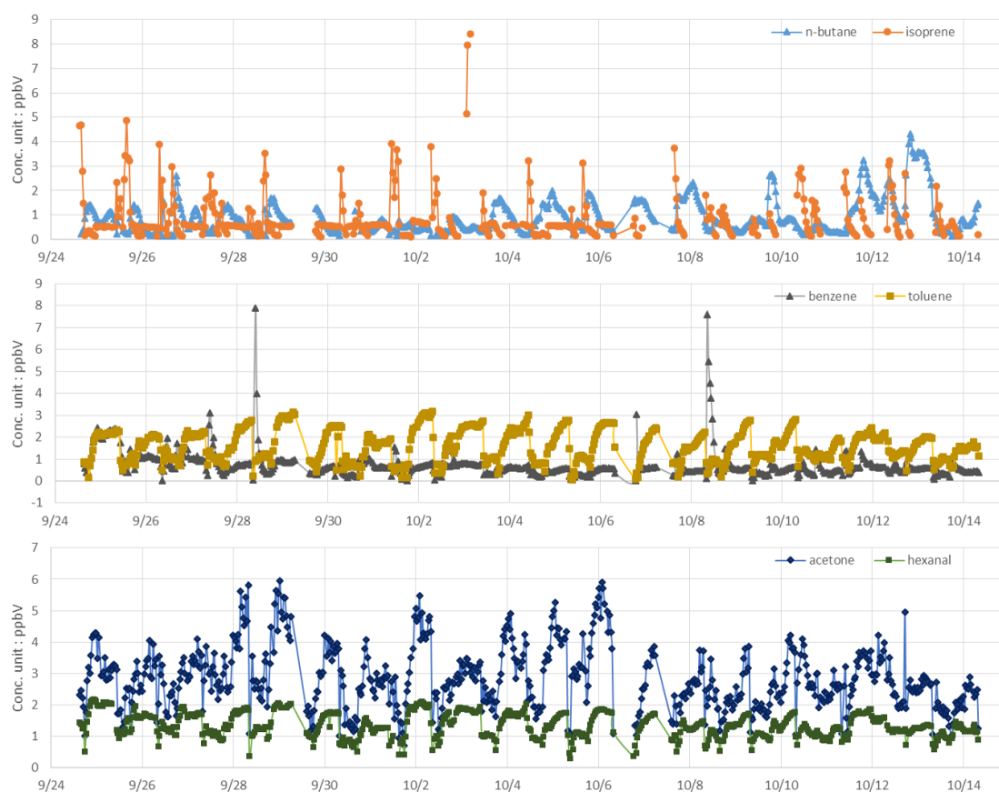
Figure 5-3 Séries temporelles des concentrations horaires moyennes de n-butane, d'isoprène, de benzène, de toluène, d'acétone et d'hexanal.
