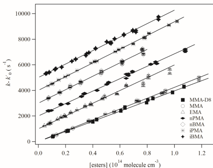
Figure 3-2 (k'_1 - k'_0) à (k'_7 - k'_0) , en fonction de la concentration en ester à température (297 \pm 2) \text{ K} (remarque, k'_1 - k'_0 = k_{\text{OH\_MMA}} \times [\text{MMA}] , k'_0 = k_{\text{H}_2\text{O}_2} \times [\text{H}_2\text{O}_2] + k_{\text{diff}} ). Les lignes représentent l'ajustement linéaire des moindres carrés. Pour une meilleure vue d'ensemble, les tracés obtenus pour l'EMA, le nPMA, le nBMA, l'iPMA et l'iBMA sont décalés verticalement de 1000, 2000, 3000, 4000 et 5000 \text{s}^{-1} , respectivement.
