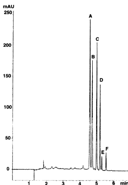
Figure 8 : Séparation par SFC de 6 flavones avec un gradient de co-solvant de 10 à 30%, repris de [166]
