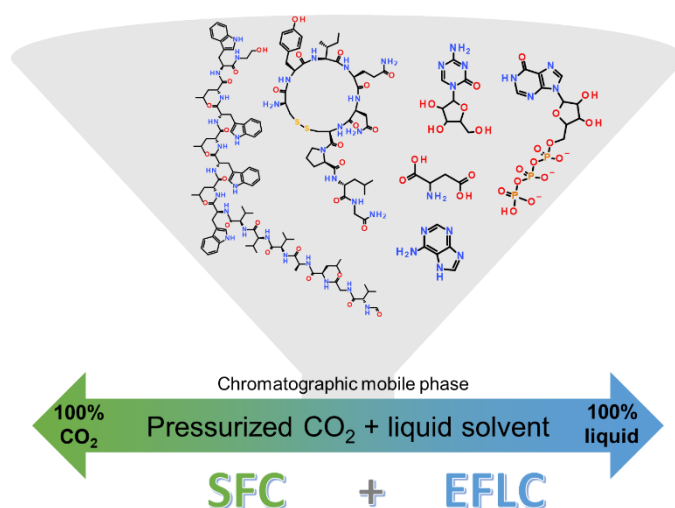
Figure 9 : Schématisation de l'analyse par UC des biomolécules étudiées, repris du résumé graphique de [169]
