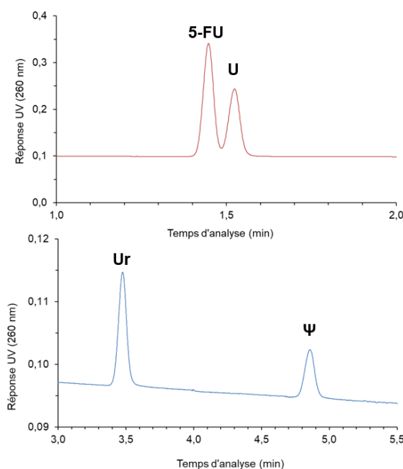
Figure 17 : Analyses par chromatographie unifiée de deux paires de bases nucléiques.
