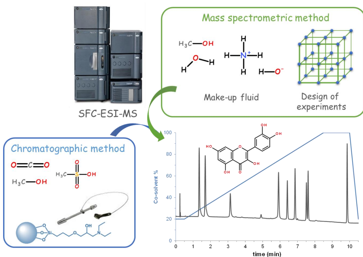
Figure 13 : Schématisation du développement de la méthode et de l'analyse de flavonoïdes par UC , repris du résumé graphique de [172]
