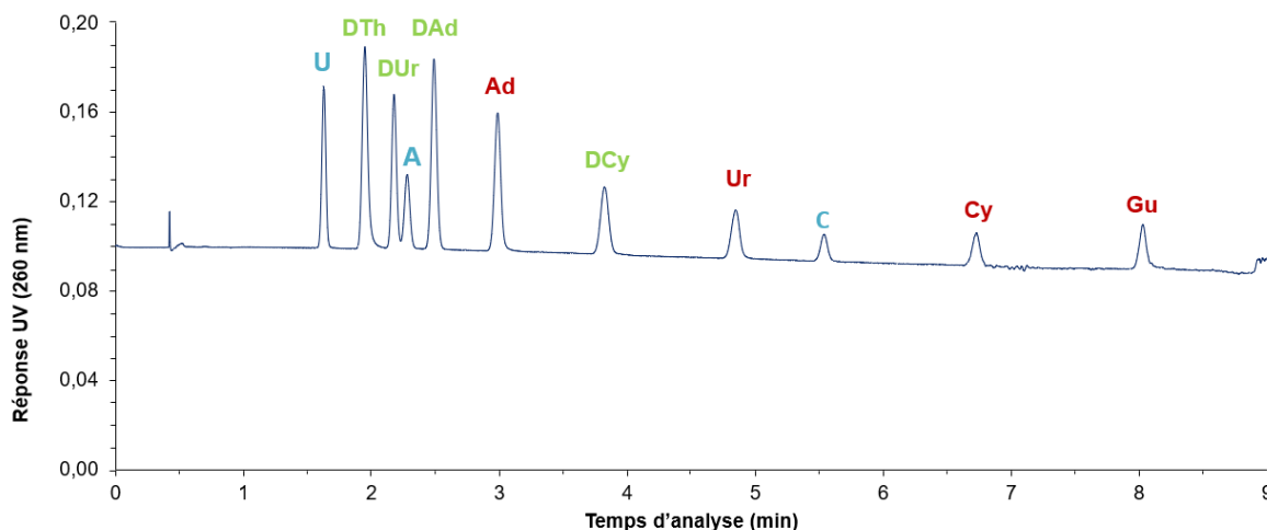
Figure 16 : Chromatogramme UV du mélange de 11 standards de bases nucléiques par UC.
