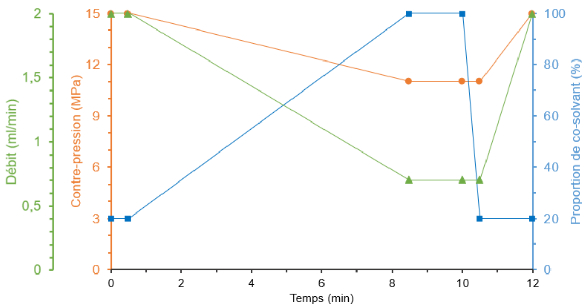
Figure 12 : Application d'une méthode UC-MS avec un gradient de pression inverse et un gradient de débit inverse, repris de [171]
