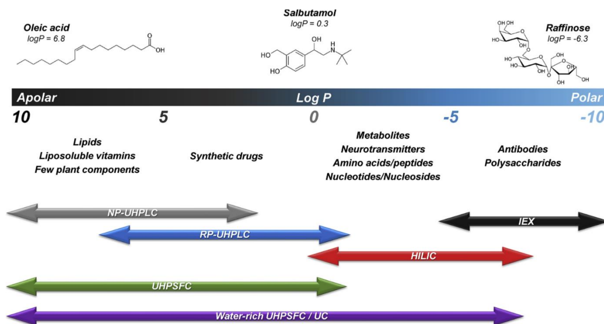
Figure 10 : Gamme de polarité des composés analysables selon la technique chromatographique, repris de [127]
