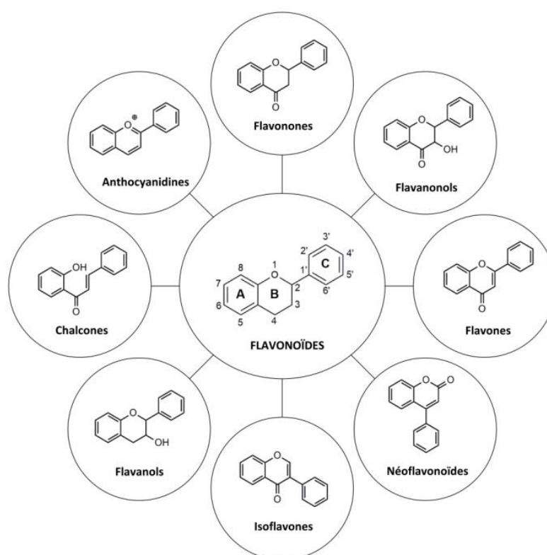
Figure 7 : Familles de flavonoïdes dérivées de la structure centrale, repris de [161]
