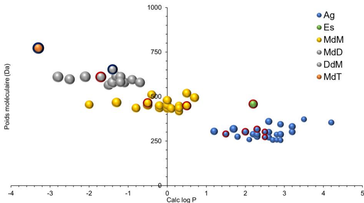
Figure 11 : Répartition des flavonoïdes sous formes d'hétérosides ou aglycones selon le poids moléculaire et la polarité, la taille des bulles représente la TPSA ou surface totale polaire.
