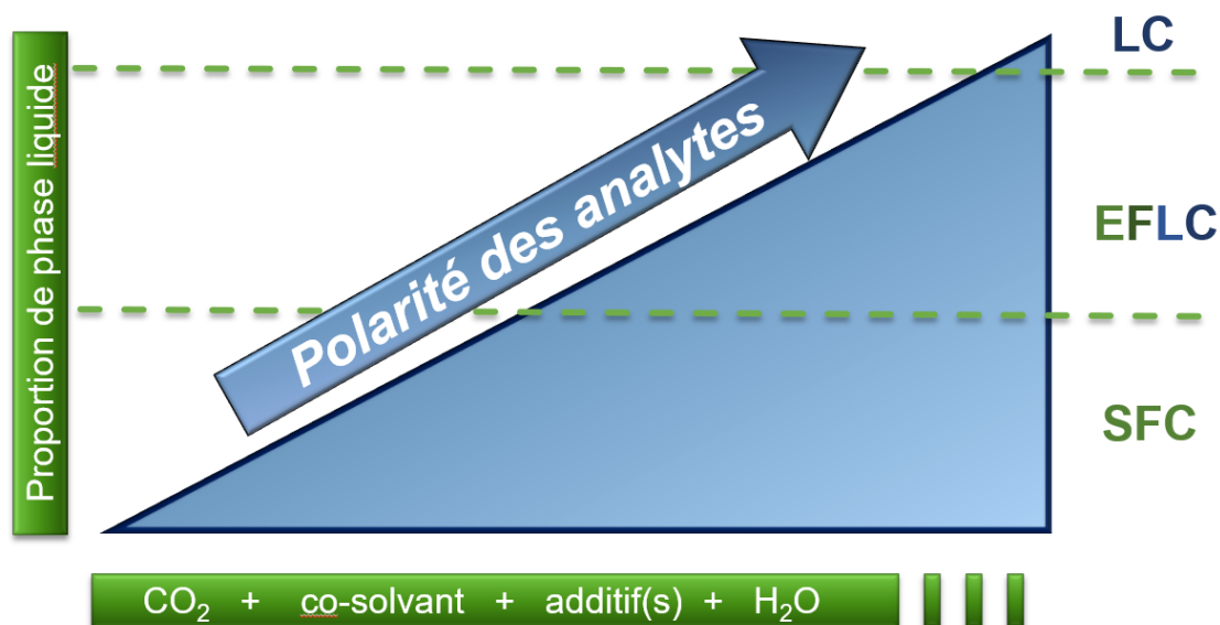
Figure 5 : Représentation des deux possibilités pour analyser des composés plus polaires, en abscisse selon la nature du co-solvant et en ordonnée selon la proportion de phase liquide.
