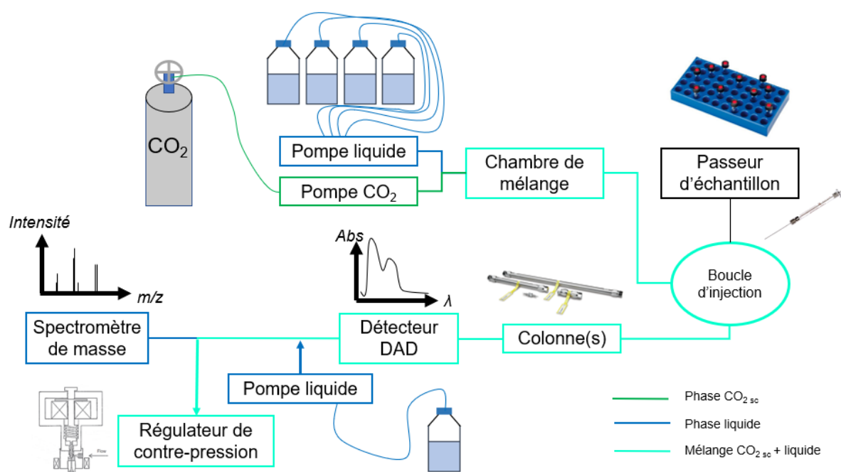
Figure 3 : Schéma du système SFC-UV-MS (UPC 2 Waters), adapté de [61], [71]
