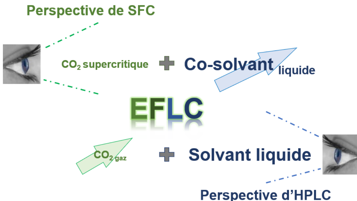
Figure 4 : Composition de la phase mobile en EFLC selon l'angle d'utilisation instrumental
