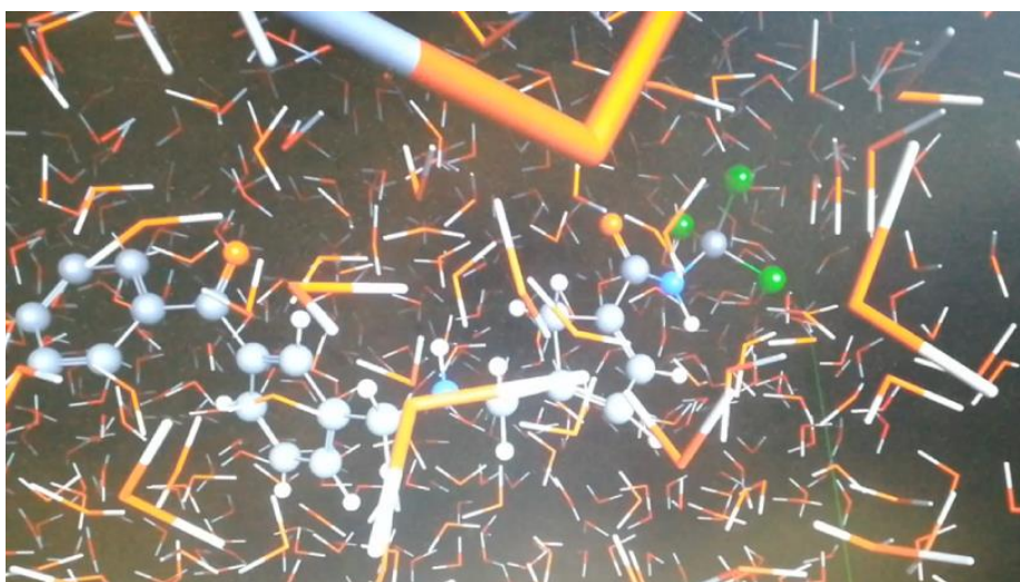
Figure 18 : Représentation d'une molécule synthétique dans un solvant (l'eau) simulé lors du calcul des conformations d'énergie minimale.
