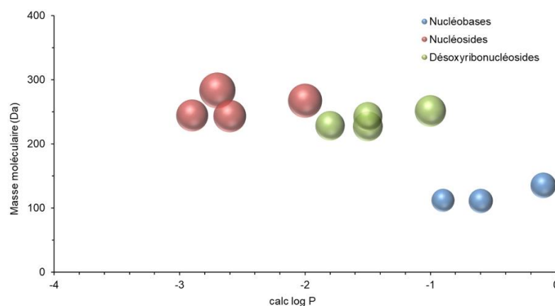
Figure 15 : Répartition des bases nucléiques étudiées selon le poids moléculaire et la polarité. La taille des bulles représente la TPSA ou surface topologique polaire
