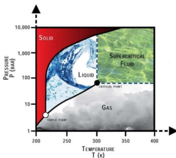
Figure 1 Diagramme d'état du dioxyde de carbone (repris sur powermag.com le 15/10/2021)
