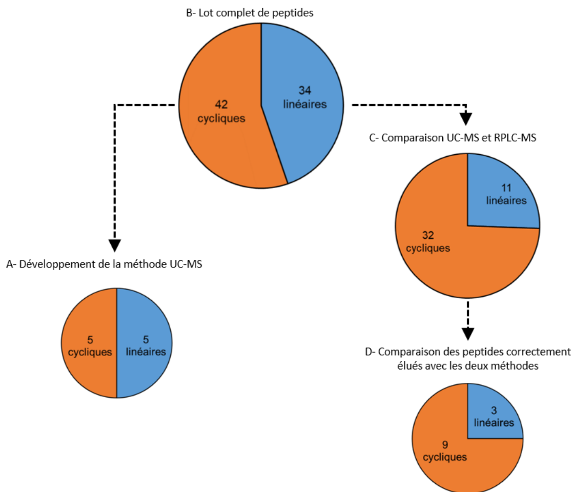
Figure 14 : Composition du set de « petits » peptides selon l'étape d'avancement du travail
