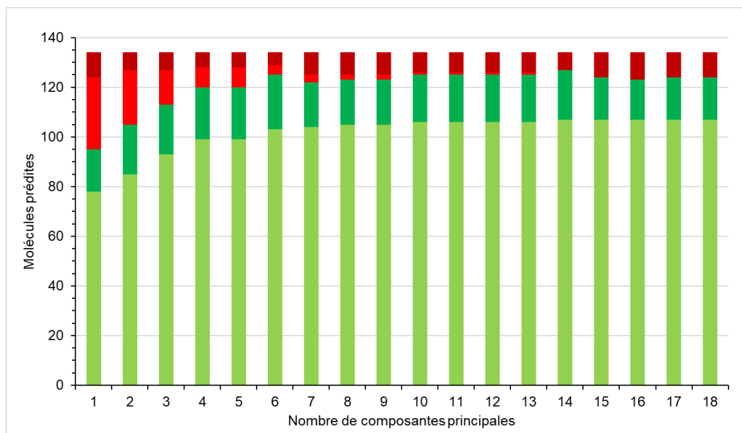
Figure 19 Qualité de la prédiction des molécules en fonction du nombre de composantes après calcul par PLS-R
