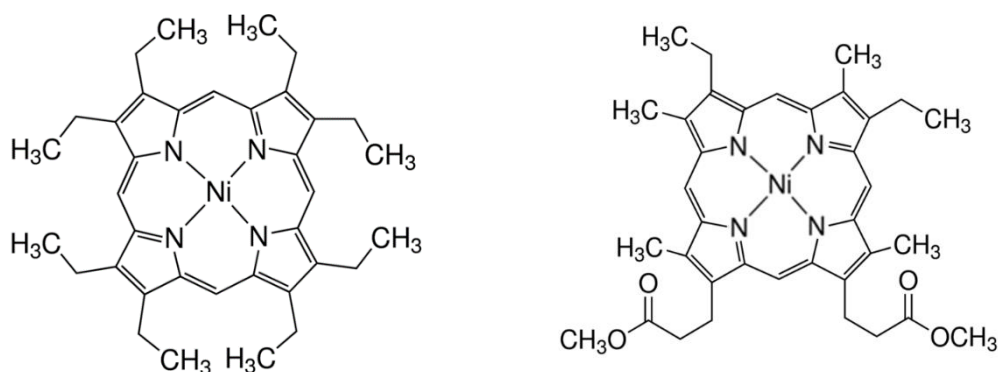
Figure 2 Structure des 2 porphyrines séparées par HPGC [38] – A gauche : Etioporphyrin II nickel et à droite : Mesoporphyrin IX dimethylester nickel
