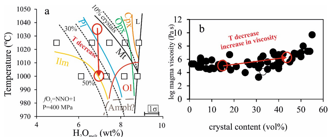
Figure 7-18: Diagramme de phase d'une andésite à 4 kbr. L'augmentation de la teneur en cristaux lorsque la température diminue de 35 °C (modifié d'après Andújar et al. 2017). b) Evolution de la viscosité en fonction de la teneur en cristaux dans les magmas (modifié d'après Andújar and Scaillet 2012).
