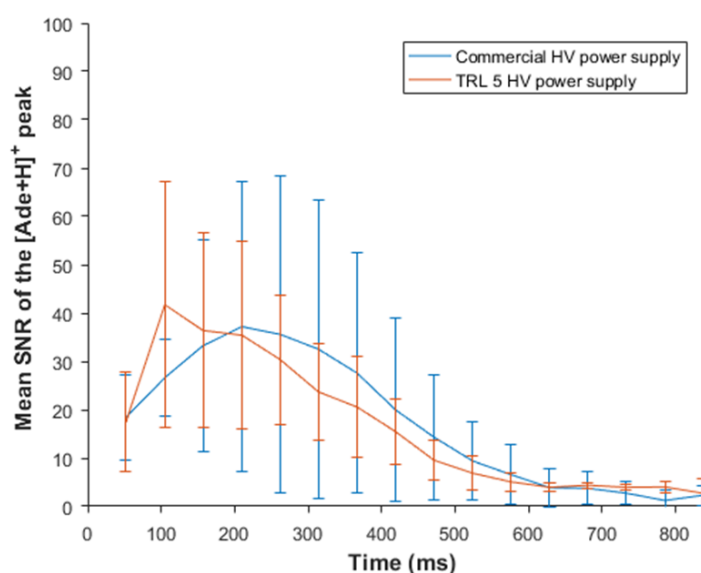
Figure 3-6 : variation du SNR moyen des pics attribués à [Ade+H]^+ mesurés à partir de 4 spectres de masse distincts acquis en mode d'ions positifs. Le même montage expérimental a été utilisé pour chaque alimentation HV. La barre d'erreur représente l'écart-type des valeurs à chaque pas de temps. Figure tirée de Cherville et al., soumis.
