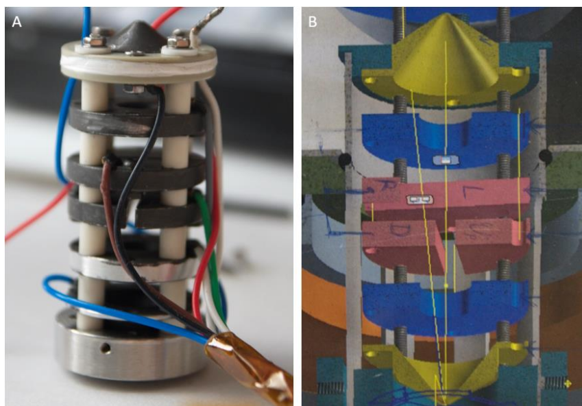
Figure 4-4 : (A) photographie de l'optique ionique de l'instrument OLYMPIA et (B) schéma de cette optique (crédit photo : B. Gaubicher).
