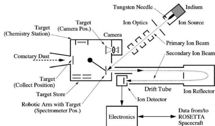
Figure 1-8 : schéma de l'instrument COSIMA, tiré de Kissel et al. , 2007
