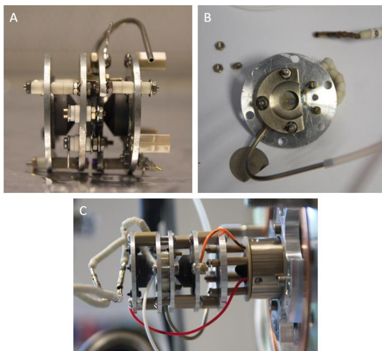
Figure 4-3 : photographies de : (A) la source d'ions par impact électronique, (B) la chambre d'ionisation ouverte et (C) la source montée sur l'instrument OLYMPIA (crédit photos : B. Gaubicher).
