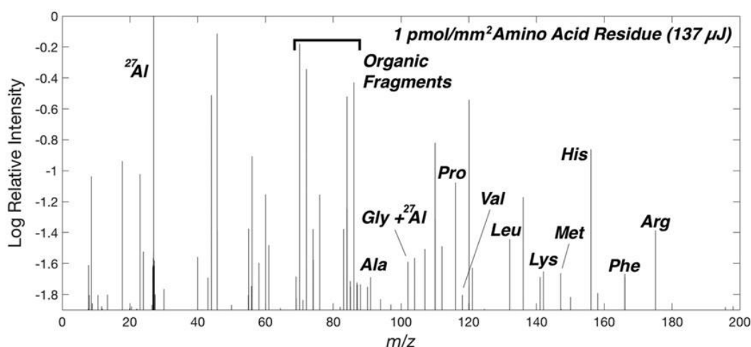
Figure 3-2 : spectre en masse issu de l'analyse par le LAb-CosmOrbitrap du résidu sec d'un échantillon de 10 \mu L d'un mélange de 16 acides aminés déposé sur une surface d'Aluminium. Parmi ces acides aminés, 12 ont été détectés avec un SNR supérieur à 3 et un écart à la masse exacte inférieur à 3 ppm. Cette figure est issue d'Arevalo Jr. et al. , 2018.
