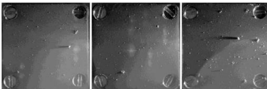
Figure A-2 : images des cibles 1D0, 2D0 et 3D0 de l'instrument Cometary Secondary Ion Mass Analyzer présent à bord de la sonde Rosetta, tirées de Langevin et al. , 2016. La lumière vient de la droite de l'image, permettant de distinguer les poussières collectées.
