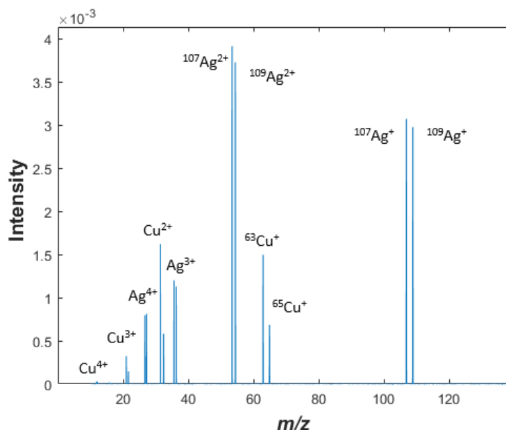
Figure 4-15 : spectre en masse d'un alliage AgCu mode d'ions positifs issu d'un signal de 20 ms obtenu à l'aide de l'instrument LILBID-OLYMPIA et calibré sur le pic attribué à l'ion ^{109}\text{Ag}^+ . L'échantillon est un fil métallique ionisé par ablation laser. Les pics correspondant aux différents ions détectés sont indiqués avec un écart à la masse exacte inférieur à 30 ppm.
