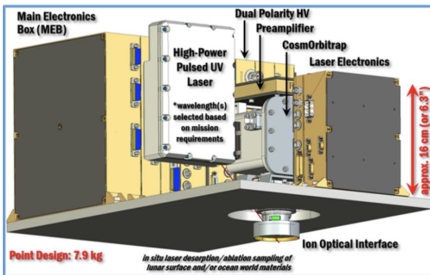
Figure 2-14 : modèle mécanique de l'instrument CRATER (crédit image : Univ. du Maryland/R. Arevalo)
