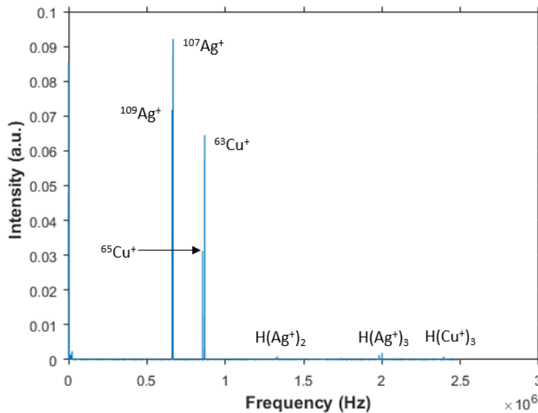
Figure 2-8 : spectre en fréquence issu du signal présenté sur la figure 2-7, issu de l'analyse d'un alliage 72% Ag/28% Cu en mode d'ions positifs grâce à l'instrument LAb-CosmOrbitrap. Les harmoniques liées à l'ion M^+ d'ordre x sont notées H(M^+)_x . Les harmoniques d'ordre 2 et 3 des pics de fréquence 0,66 MHz sont visibles aux fréquences 1,3 et 2,0 MHz. Les harmoniques d'ordre 3 des pics de fréquence 0,8 MHz sont visible à la fréquence 2,4 MHz.
