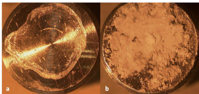
Figure 2-19 : photos de deux portes échantillons utilisés avec le LAB-CosmOrbitrap, (a) solution contenant 16 acides aminés ( 10^{-3} mol.L ^{-1} ) et 1 wt% \text{MgSO}_4 séchée sur surface d'Aluminium, (b) poudre d'Adénine commerciale pressée sur surface d'Indium
