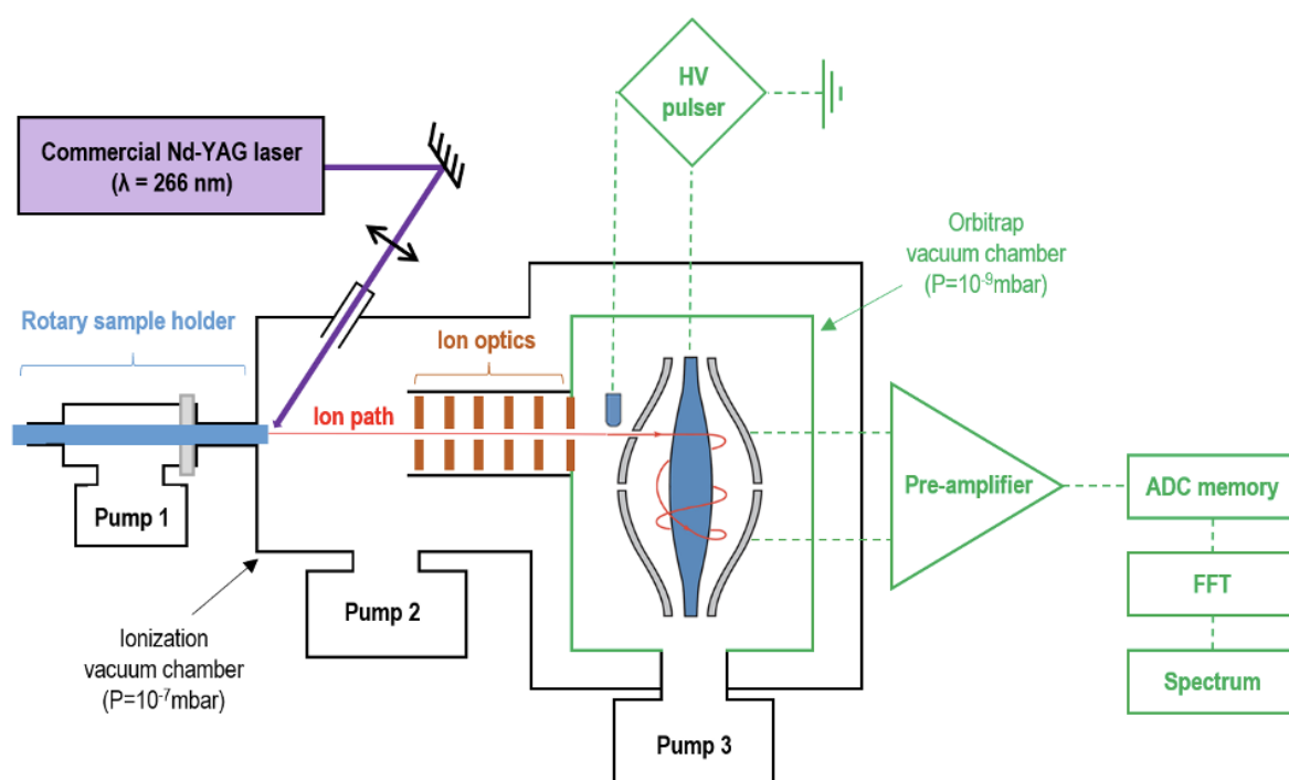
Figure 2-15 : Schéma de fonctionnement du LAb-CosmOrbitrap. Les parties en vert sont les éléments du CosmOrbitrap en cours de développement, les autres éléments sont commerciaux. Tiré de Cherville et al., soumis.
