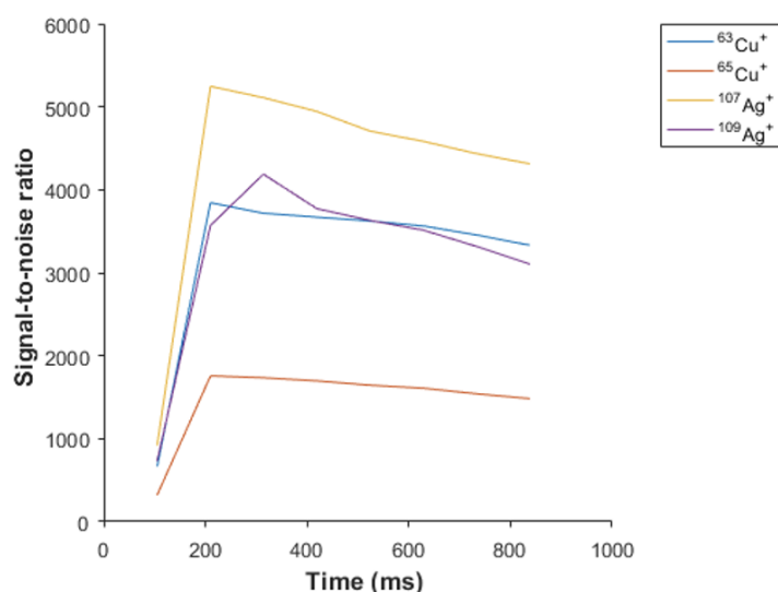
Figure 2-10 : rapport signal sur bruit des pics attribués aux ions ^{63}\text{Cu}^+ , ^{65}\text{Cu}^+ , ^{107}\text{Ag}^+ et ^{109}\text{Ag}^+ du spectre présenté sur la figure 2-9 en fonction du temps. Le signal initial a été découpé en 8 parties de même dimension et calibrées sur le pic de fréquence 666,5 kHz, attribué à la masse de ^{107}\text{Ag}^+ .
