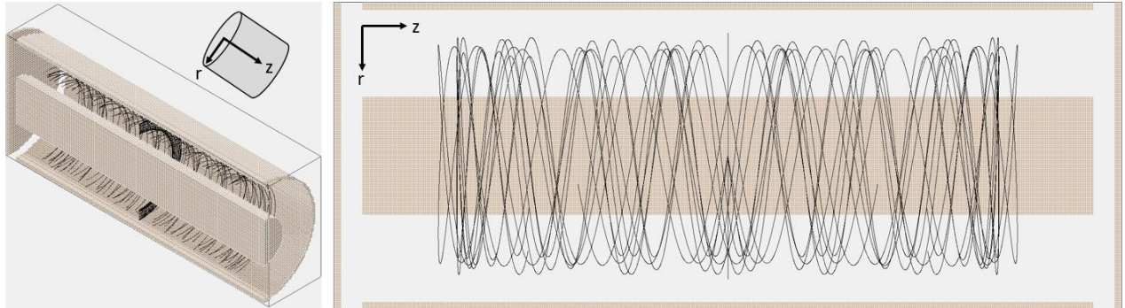
Figure 2-1 : simulation SIMION d'un piège de Kingdon. Les courbes noires correspondent aux déplacements de 8 ions distincts ( m/z et énergie cinétique initiale différentes). Le piège est visualisé selon une coupe longitudinale pour une représentation plus claire du dispositif. Un des disques à l'extrémité du piège a été retiré de la représentation de gauche.
