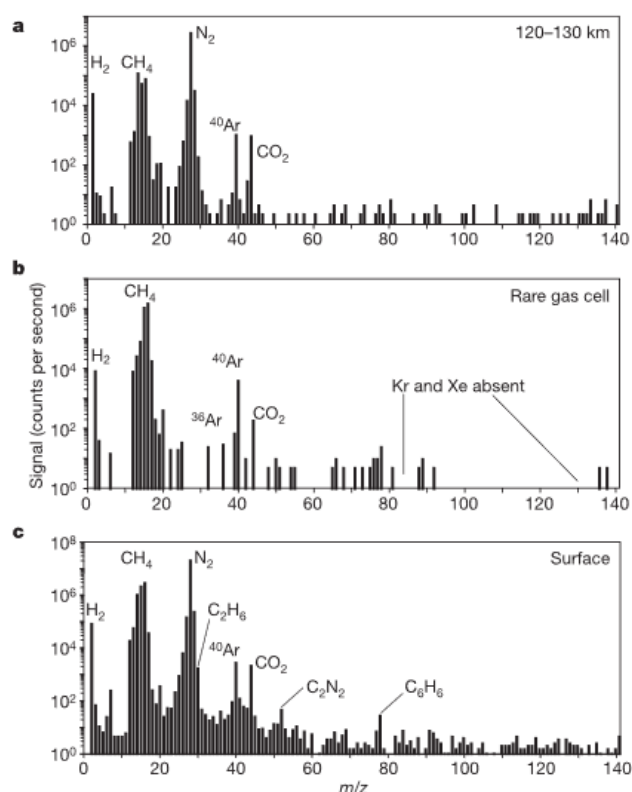
Figure 1-15 : spectres de masse issus de l'instrument de spectrométrie de masse présent à bord de l'atterrisseur Huygens. (a) moyenne de 104 spectres acquis entre 120 et 130 km d'altitude, (b) moyenne de 43 spectres issus de la cellule consacrée à l'analyse des gaz rares, (c) moyenne de 432 spectres acquis à la surface de Titan. Tiré de Niemann et al. , 2005.
