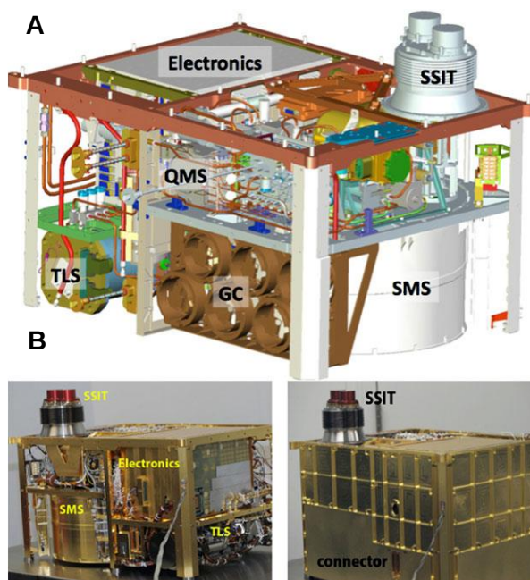
Figure 1-7 : modèle de l'instrument SAM. A) modèle numérique, B) photographies de l'instrument sans et avec les plaques latérales. TLS : Tunable Laser Spectrometer ; QMS : Quadrupole Mass Spectrometer ; GC : Gas Chromatograph ; SSIT : Solid Sample Inlet Tube ; SMS : Sample Manipulation System. Tiré de Mahaffy et al., 2012.
