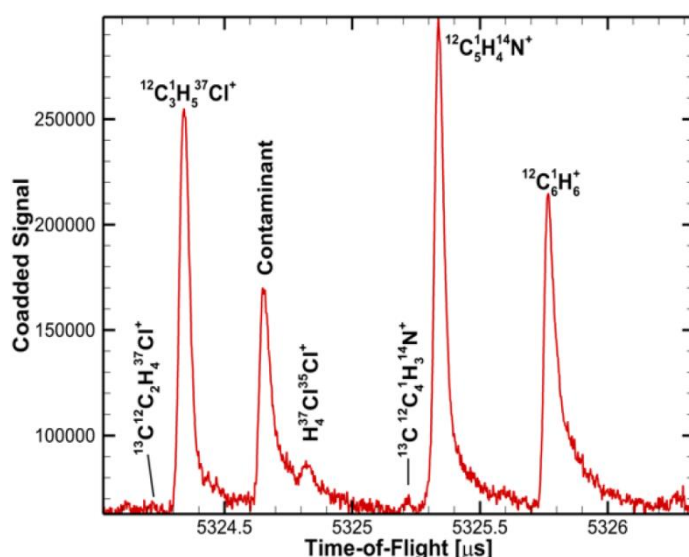
Figure 1-21 : détail du spectre de masse d'un mélange de 1,2-dichloropropane, pyrimidine et benzène obtenu par l'instrument MASPEX centré autour de la masse 78. La résolution donnée pour ce spectre est de 55000, mesurée à mi-hauteur du pic. Tiré de Waite et al. , 2019.
