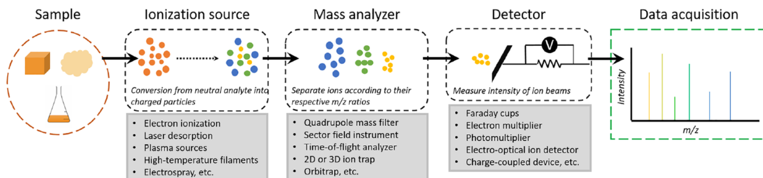
Figure 1-2 : schéma synthétique des différents composants d'un instrument de spectrométrie de masse. La modularité des différents sous-systèmes permet de réaliser un certain nombre de permutations dans la conception des spectromètres de masse, définissant ainsi des combinaisons uniques adaptées aux objectifs scientifiques de l'instrument. Tiré d'Arevalo Jr et al., 2020.
