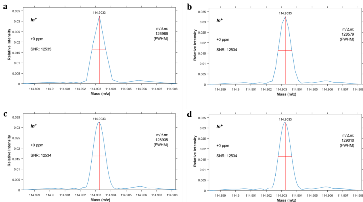
Figure 2-27 : détail du pic attribué à l'ion ^{115}\text{In}^+ du signal considéré après application d'un zero-padding de : (a) 0 ; (b) 1 ; (c) 3 ; (d) 6. La calibration a été effectuée sur ce pic. La résolution m/\Delta m est calculée à partir de la largeur à mi-hauteur représentée par le segment rouge horizontal et la valeur désignée par le sommet du pic et représentée par le segment rouge vertical.
