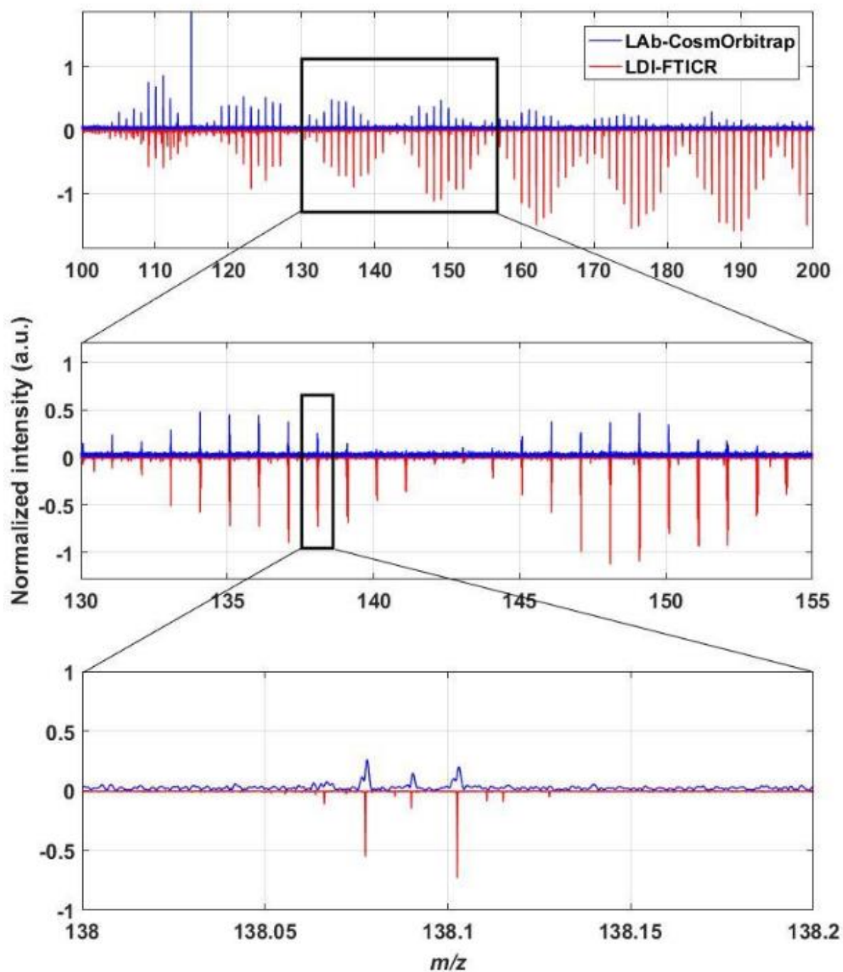
Figure 3-3 : spectres en masse issu de l'analyse de tholins avec le Lab-CosmOrbitrap (en bleu) et un LDI-FTICR commercial (en rouge). Le panneau supérieur montre les spectres sur la gamme de masse [100;200], le panneau central sur la gamme de masse [130;155] et le panneau inférieur sur la gamme de masse [138;138,2]. Cette figure est tirée de Selliez et al., 2020.
