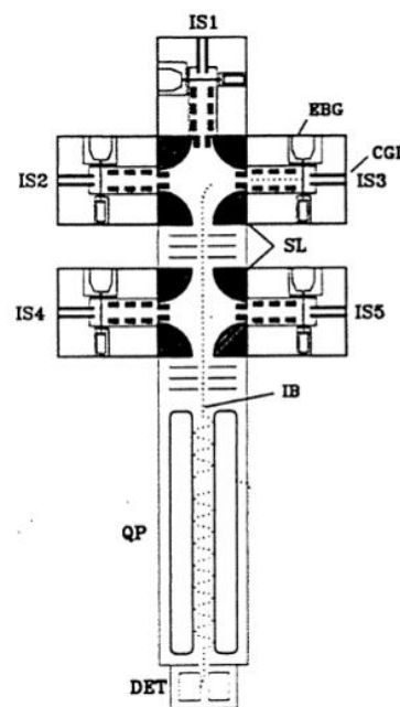
Figure 1-14 : schéma de l'instrument de spectrométrie de masse couplé au dispositif de chromatographie en phase gazeuse présent à bord de l'atterrisseur Huygens, adapté de Niemann et al. , 1997.
