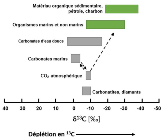
Figure 1-24 : anomalie isotopique en ^{13}\text{C} moyenne en fonction des processus à l'œuvre. Les barres vertes indiquent les processus d'origine biotiques. Adaptée de Hand et al. , 2017 et de Hoefs, 2018.
