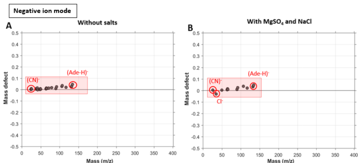
Figure 3-13 : défaut de masse des pics détectés en fonction de m/z dans les échantillons d'adénosine pure et d'adénosine + MgSO 4 + NaCl. La FFT a été appliquée sur les signaux entre 10 et 838 ms. Le panneau A correspond à l'analyse en mode d'ions négatifs de l'échantillon d'adénosine pure ; le panneau B à l'analyse en mode d'ions négatifs de l'échantillon d'adénosine + MgSO 4 + NaCl. Les pics caractéristiques tels que le pic pseudomoléculaire, Cl - et CN - ont été mis en évidence.
