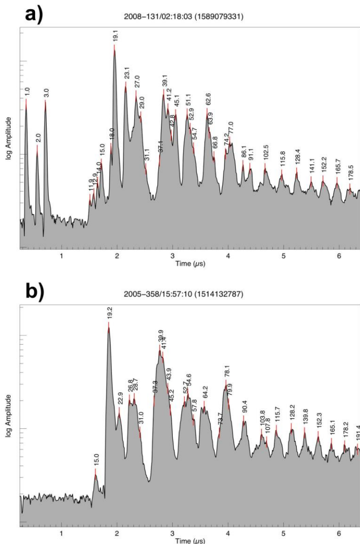
Figure 1-19 : spectres typiques montrant la présence de composés organiques massifs, tirés Postberg et al. , 2018.
