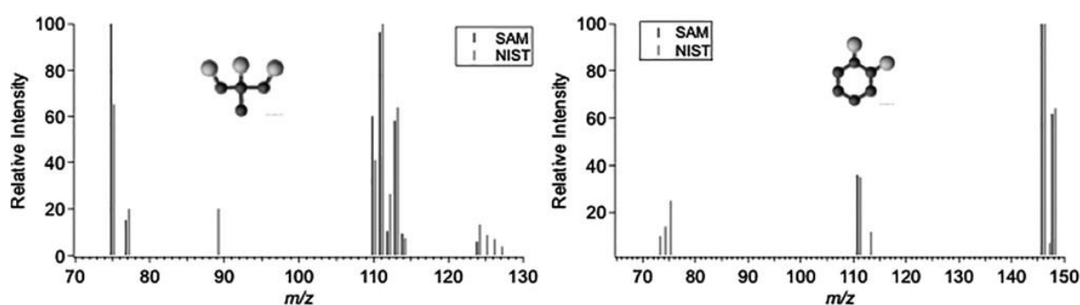
Figure A-9 : spectres de masse normalisés de 1,2,3-trichloro-2-méthylpropane et de 1,2-dichlorobenzène issus de l'échantillon CB-5 de l'instrument Sample Analysis at Mars, tirés de Szopa et al. , 2020. Les spectres de référence issus de la National Institute of Standards and Technology sont représentés sur le même graphique pour permettre une comparaison avec les résultats de l'instrument SAM.
