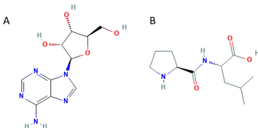
Figure 3-9 : structures de la molécule (A) d'adénosine et (B) de proline-leucine, tirées de la bibliothèque PubChem.
