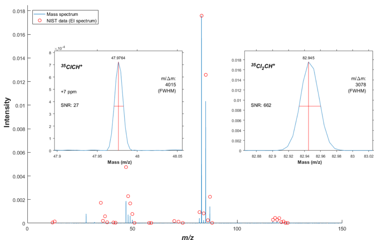
Figure 4-8 : spectre en masse de chloroforme acquis en mode d'ions positifs. Les points rouges indiquent l'amplitude des pics du spectre de masse issu de la bibliothèque de spectres du NIST, normalisés sur l'amplitude du pic le plus intense du spectre acquis grâce à l'instrument EI-OLYMPIA. Les panneaux latéraux montrent des détails des pics attribués aux pics de ^{35}\text{ClC}^+ et ^{35}\text{Cl}_2\text{CH}^+ .
