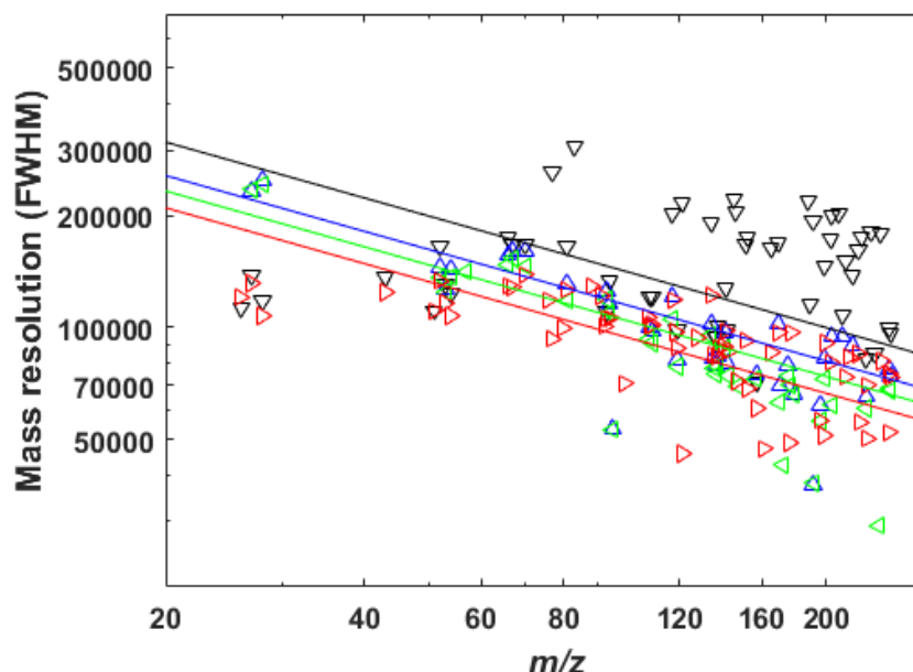
Figure 2-23 : résolution en masse (calculée à mi-hauteur de chaque pic) en fonction du rapport m/z pour les pics détectés sur le spectre issu du signal auquel a été appliqué la fenêtre rectangulaire (en noir), la fenêtre de Hann (en bleu), la fenêtre de Blackman (en vert) et la fenêtre nouvellement développée dans le cadre de cette thèse (en rouge). Les points représentent chaque valeur individuelle, la droite correspond à la loi de décroissance décrite par l'équation 2-16.
