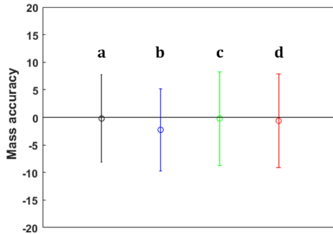
Figure 2-26 : écart à la masse exacte moyen pour les pics détectés sur le spectre issu du signal auquel a été appliqué la fenêtre rectangulaire (en noir), la fenêtre de Hann (en bleu), la fenêtre de Blackman (en vert) et la fenêtre nouvellement développée dans le cadre de cette thèse (en rouge). La barre d'erreur correspond à l'écart-type des valeurs.
