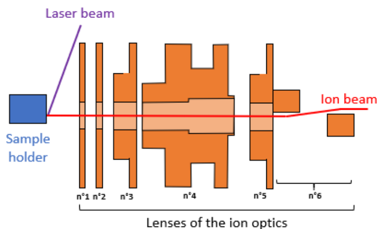
Figure 2-17 : schéma de l'optique ionique du LAB-CosmOrbitrap
