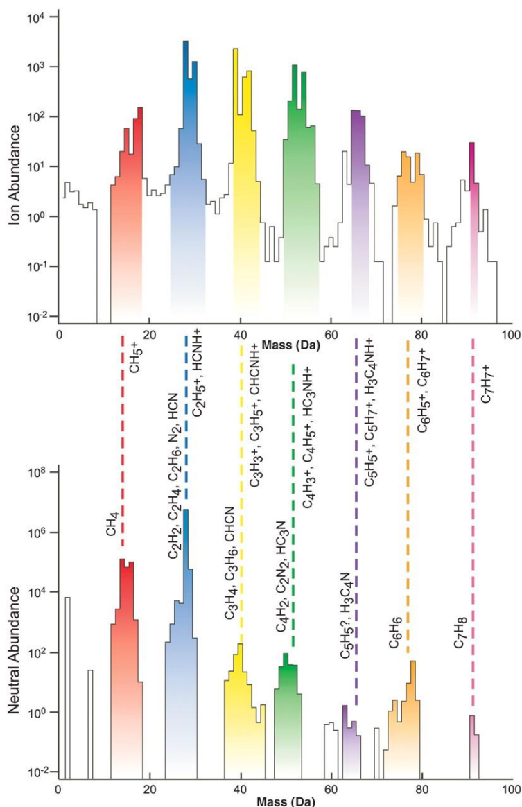
Figure 1-12 : spectres en masse moyen mesuré par l'instrument INMS lors du 19 ème survol de Titan par la sonde Cassini. L'altitude de la sonde était comprise entre 950 et 1000 km. La partie supérieure correspond aux ions détectés, la partie inférieure aux espèces neutres détectées. Différentes familles correspondant aux molécules possédant un nombre d'atomes de Carbone différents ont été mises en évidence, ainsi que l'identification supposée des molécules détectées. Tiré de Waite et al. , 2007.
