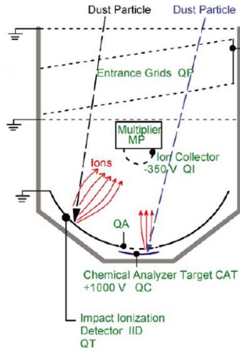
Figure 1-16 : schéma de l'instrument CDA, adapté de Srama et al. , 2004.
