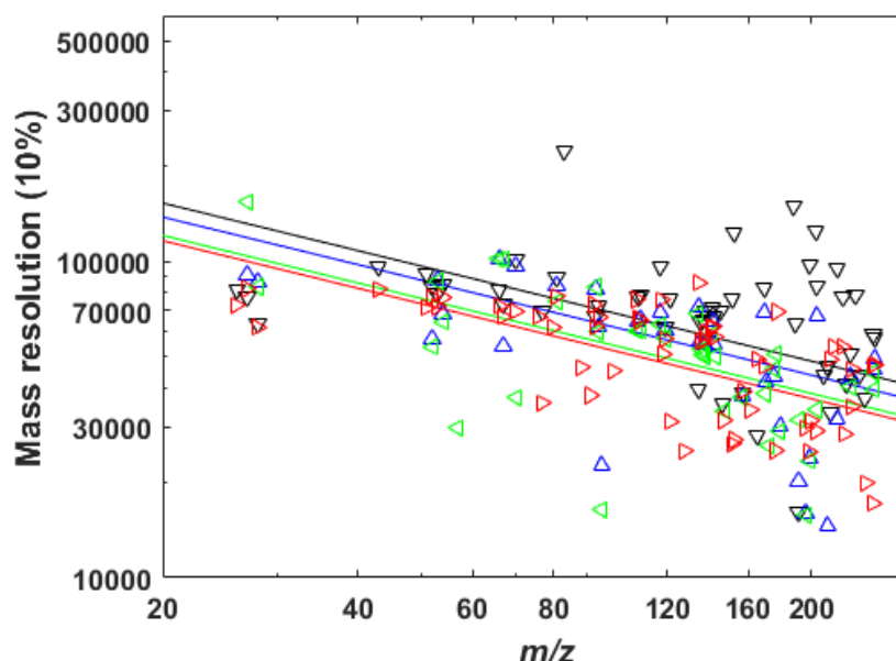
Figure 2-24 : résolution en masse (calculée à 10 % de la hauteur de chaque pic) en fonction du rapport m/z pour les pics détectés sur le spectre issu du signal auquel a été appliqué la fenêtre rectangulaire (en noir), la fenêtre de Hann (en bleu), la fenêtre de Blackman (en vert) et la fenêtre nouvellement développée dans le cadre de cette thèse (en rouge). Les points représentent chaque valeur individuelle, la droite correspond à la loi de décroissance décrite par l'équation 2-16.
