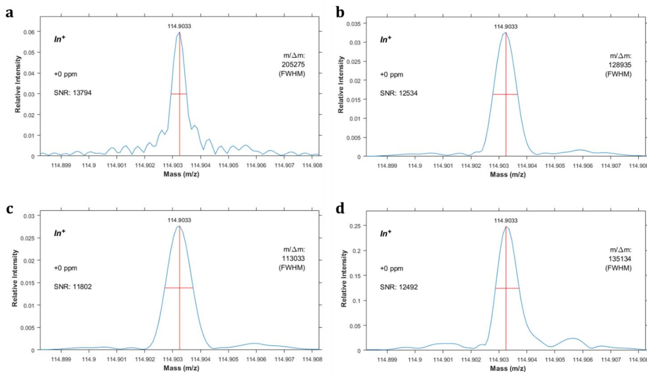
Figure 2-22 : détail du pic attribué à l'ion ^{115}\text{In}^+ du signal considéré après application d'une fonction d'apodisation : (a) fenêtre rectangulaire ; (b) fenêtre de Hann ; (c) fenêtre de Blackman ; (d) fenêtre nouvellement développée dans le cadre de cette thèse. La calibration a été effectuée sur ce pic. La résolution m/\Delta m est calculée à partir de la largeur à mi-hauteur représentée par le segment rouge horizontal et la valeur désignée par le sommet du pic et représentée par le segment rouge vertical.
