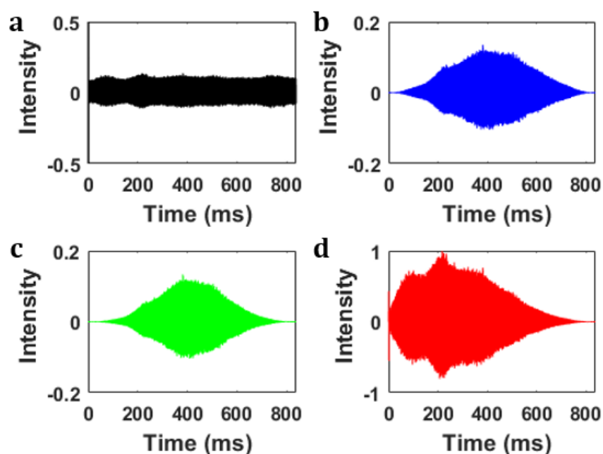
Figure 2-21 : signaux étudiés après application d'une fonction d'apodisation : (a) fenêtre rectangulaire ; (b) fenêtre de Hann ; (c) fenêtre de Blackman ; (d) fenêtre nouvellement développée dans le cadre de cette thèse
