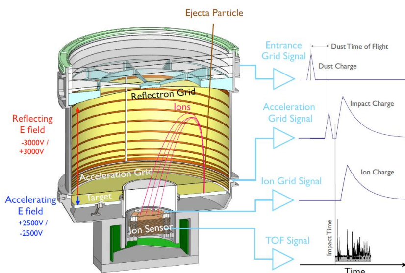
Figure 1-20 : représentation des différents éléments constituant l'instrument SUDA avec le détail des différentes mesures effectuées, tirée de Kempf et al. , 2014.
