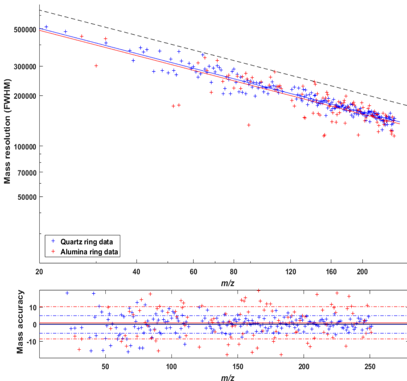
Figure 3-8 : comparaison des performances analytiques du LAB-CosmOrbitrap utilisant les deux bagues séparatrices des électrodes externes de la cellule Orbitrap. Panneau supérieur : résolution en masse (calculée à mi-hauteur de chaque pic) moyenne des pics détectés de même attribution chimique des différents spectres de chaque série d'expériences effectuée en fonction du rapport m/z . Les points en bleu correspondent aux données issues de la série d'expériences effectuée en utilisant une cellule Orbitrap équipée d'une bague séparatrice en quartz, les points en rouge aux données issues de la série d'expériences effectuée en utilisant la même cellule équipée d'une bague séparatrice en alumine. Les droites bleue et rouge correspondent respectivement à la loi de décroissance décrite par l'équation 3-5 pour les séries d'expériences effectuée avec la bague séparatrice en quartz et celle effectuée avec la bague séparatrice en alumine. La droite en pointillés noirs correspond à la résolution maximale pour un signal de 832 ms échantillonné à 5 MHz. Panneau inférieur : écart à la masse exacte moyen des mêmes pics en fonction du rapport m/z . Les points en bleu correspondent aux données issues de la série d'expériences effectuée en utilisant une cellule Orbitrap équipée d'une bague séparatrice en quartz, les points en rouge aux données issues de la série d'expériences effectuée en utilisant la même cellule équipée d'une bague séparatrice en alumine. Les droites pleine rouge et pleine bleue correspondent respectivement à la valeur d'écart à la masse exacte des valeurs issues de la série d'expériences effectuée avec la bague séparatrice en quartz et à la valeur d'écart à la masse exacte des valeurs issues de la série effectuée avec la bague séparatrice en alumine. Les droites en points-pointillés correspondent à l'écart-type des valeurs par rapport à la moyenne ; les couleurs des droites en points-pointillés suivent le même code couleur que les droites pleines.
