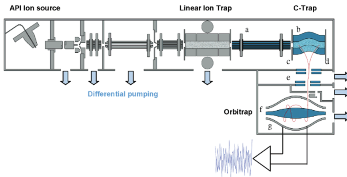
Figure 2-11 : schéma de l'instrument LTQ-Orbitrap. (a) Octapôle de transfert, (b) C-trap, (c) Electrode d'entrée, (d) Electrode de piégeage, (e) Optique ionique, (f) Electrode centrale l'Orbitrap, (g) Electrode externe de l'Orbitrap. Les flèches indiquent les interfaces avec le système de pompage. Tiré de Makarov et al. 2006.
