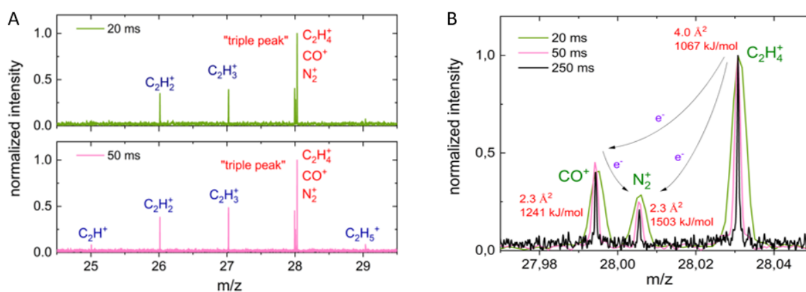
Figure 4-9 : (A) spectres en masse du mélange de gaz CO/N_2/C_2H_4 obtenus à partir d'un signal de 20 ms (en vert) et d'un signal de 50 ms (en rose) acquis en mode d'ions positifs grâce à l'instrument EI-OLYMPIA, (B) détail des pics présents à la masse nominale 28 obtenus à partir d'un signal de 20 ms (en vert), d'un signal de 50 ms (en rose) et d'un signal de 250 ms (en noir) acquis en mode d'ions positifs grâce à l'instrument EI-OLYMPIA. Ces figures sont issues de Zymak et al., in prep.
