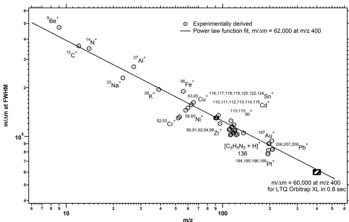
Figure 3-1 : résolution en masse mesurée à mi-hauteur des pics en fonction du rapport m/z , mesurée à partir des différents spectres obtenus grâce à différents échantillons inorganiques, en mode d'ions positifs à l'aide du LAB-CosmOrbitrap. La droite correspond à la loi de décroissance décrite dans Makarov, 2000 et Perry et al., 2008. Cette figure est tirée de Briois et al., 2016.
