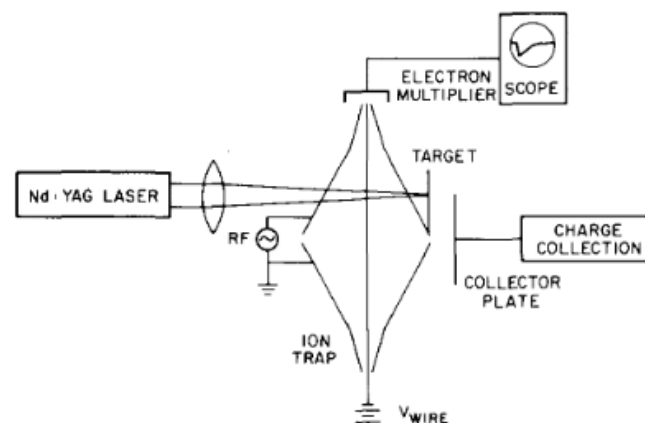
Figure 2-2 : schéma du piège de Knight. Tiré de Knight, 1981
