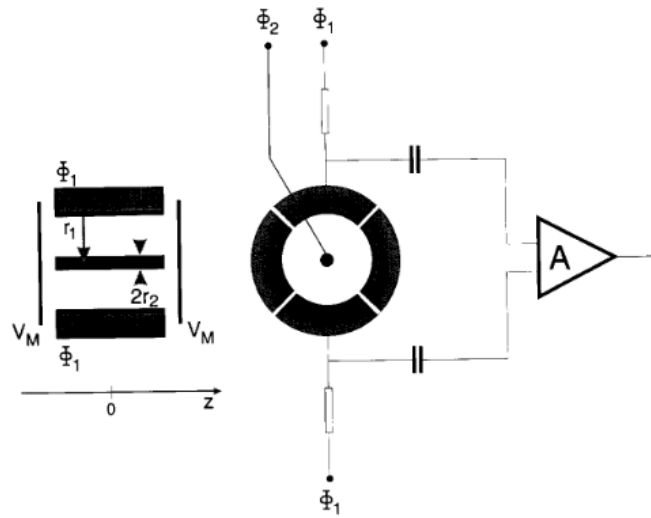
Figure 2-3 : schéma du dispositif proposé comme modèle d'analyseur en masse par Oksman. Tiré de Oksman, 1995.
