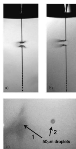
Figure 4-10 : a) et b) photographies du faisceau d'eau au sein du dispositif LILBID prises lors de l'impact laser, c) détail des gouttelettes. Tiré de Charvat and Abel, 2007.
