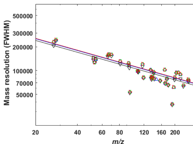
Figure 2-28 : résolution en masse (calculée à mi-hauteur de chaque pic) en fonction du rapport m/z pour les pics détectés sur le spectre issu du signal auquel a été appliqué un zero-padding de 0 (en noir), 1 (en bleu), 3 (en vert) et 6 (en rouge). Les points représentent chaque valeur individuelle, la droite correspond à la loi de décroissance décrite par l'équation 2-16.
