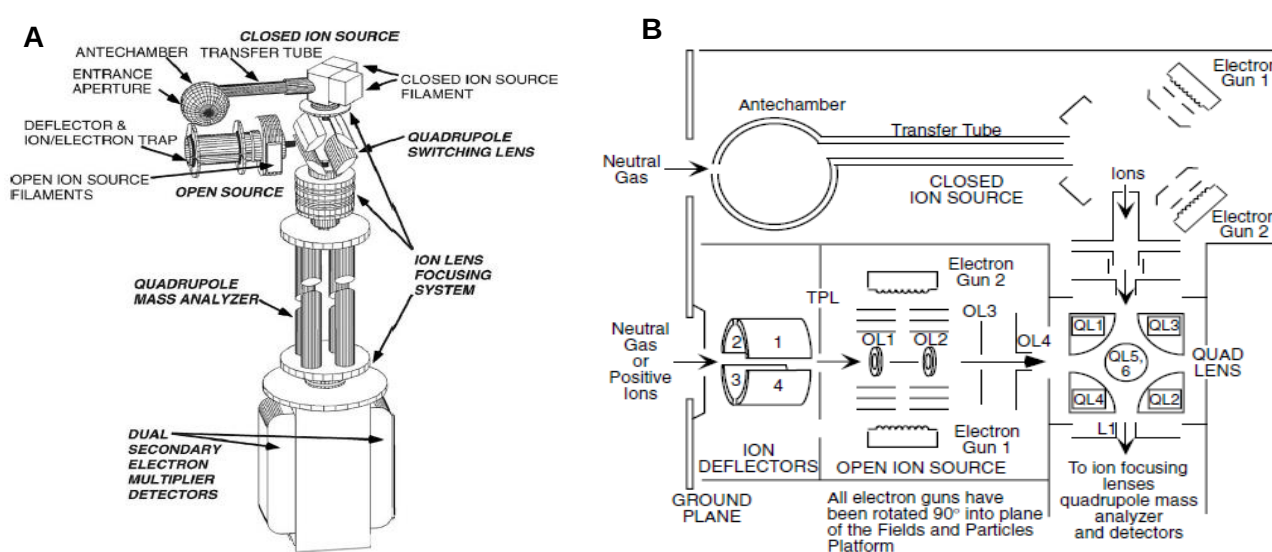
Figure 1-10 : schémas illustrant les différents composants de l'instrument INMS. A) différents éléments de l'instrument global, B) sources d'ionisation et le système d'injection des ions dans l'analyseur en masse. tirés de Waite et al. , 2004
