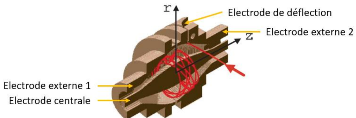
Figure 2-5 : schéma de la cellule Orbitrap. La flèche rouge représente l'injection des ions, le trait rouge leur trajectoire dans la cellule. Adapté de Hu et al., 2005.
