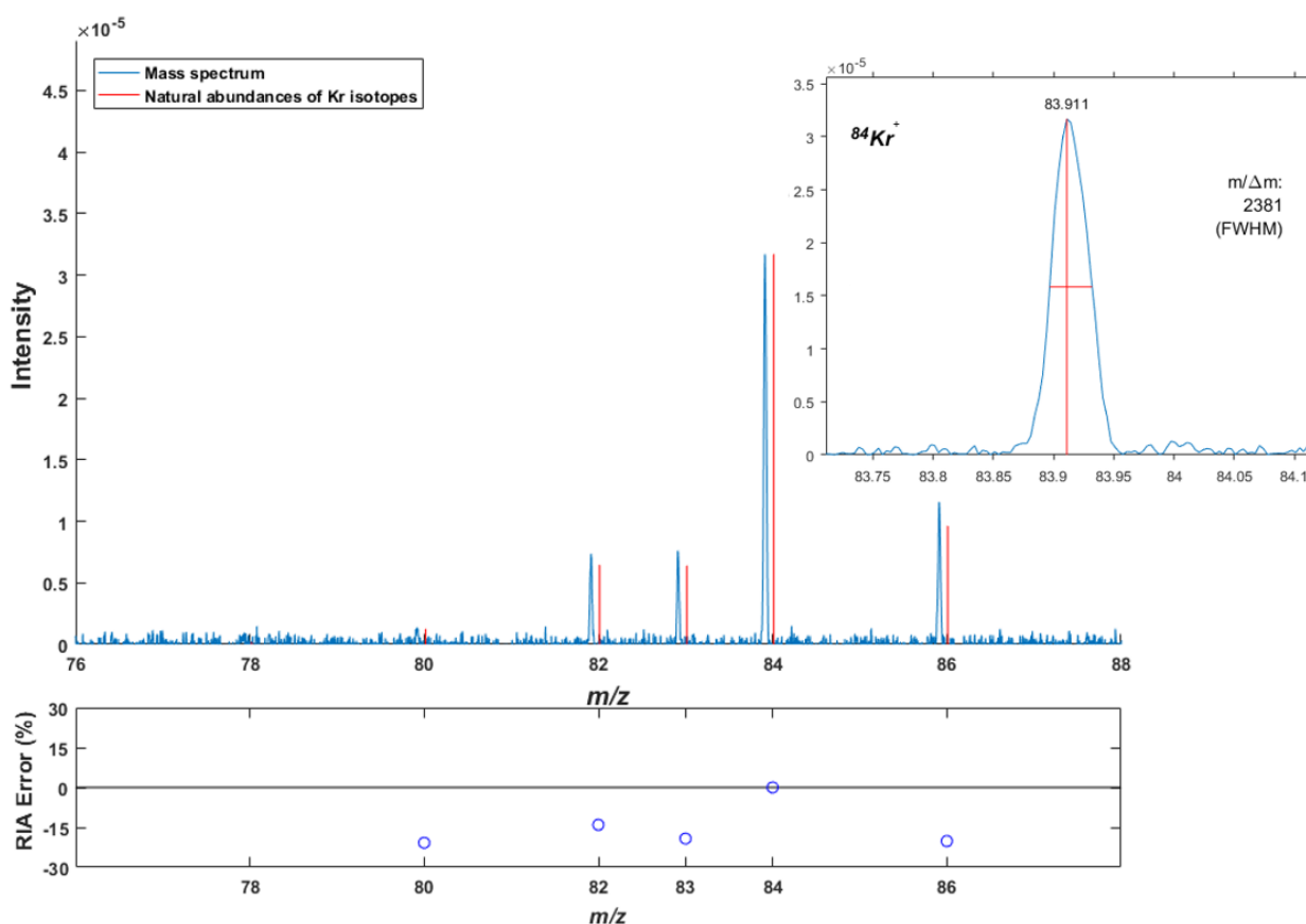
Figure 4-7 : Spectre en masse de Krypton acquis grâce à l'instrument EI-OLYMPIA Panneau supérieur : spectre en masse de Krypton acquis en mode d'ions positifs. Les barres verticales rouges correspondent à l'intensité relative théorique des 5 isotopes détectés par l'instrument EI-OLYMPIA. Le panneau à droite montre un détail du pic attribué à l'ion ^{84}\text{Kr}^+ . Panneau inférieur : erreurs sur les abondances isotopiques relatives calculées à partir du spectre.
