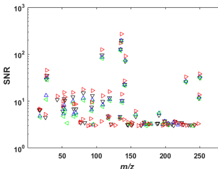
Figure 2-25 : SNR en fonction du rapport m/z pour les pics détectés sur le spectre issu du signal auquel a été appliqué la fenêtre rectangulaire (a, en noir), la fenêtre de Hann (b, en bleu), la fenêtre de Blackman (c, en vert) et la fenêtre nouvellement développée dans le cadre de cette thèse (d, en rouge). Chaque point correspond à un pic détecté. L'amplitude considérée est la valeur maximum atteinte par le pic. Le niveau de bruit considéré est la valeur d'intensité moyenne de tous les points de la gamme de masse 1-800.
