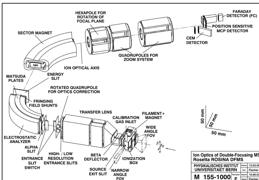
Figure A-4 : vue des différents éléments de l'instrument DFMS-ROSINA, tiré de Balsiger et al., 2007.
