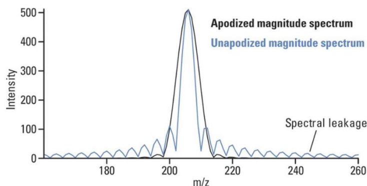
Figure 2-20 : exemple d'un spectre simulé avec application d'une fonction d'apodisation de type Hann (en noir) et application d'une fonction d'apodisation rectangulaire (en bleu). Tiré de Scigelova et al., 2011.
