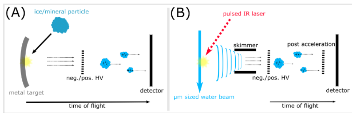
Figure 4-12 : comparaison de l'ionisation par (A) impact de poussière hyper vélocité sur une surface métallique, analogue à celle au sein de l'instrument CDA et par (B) source LILBID. La seconde est une méthode considérée comme analogue à la première. Adaptée de Klenner et al., 2019.
