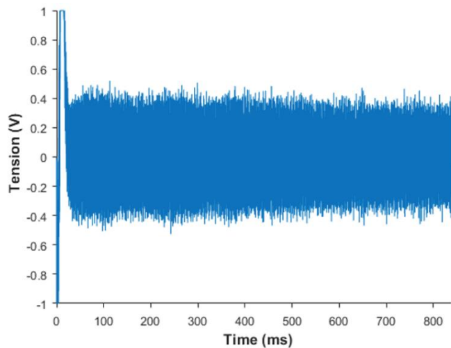
Figure 2-7 : signal mesuré par une cellule Orbitrap. Ce signal spécifique est issu de l'analyse d'un alliage 72% Ag/28% Cu en mode d'ions positifs grâce à l'instrument LAb-CosmOrbitrap décrit à la section 2.3.
