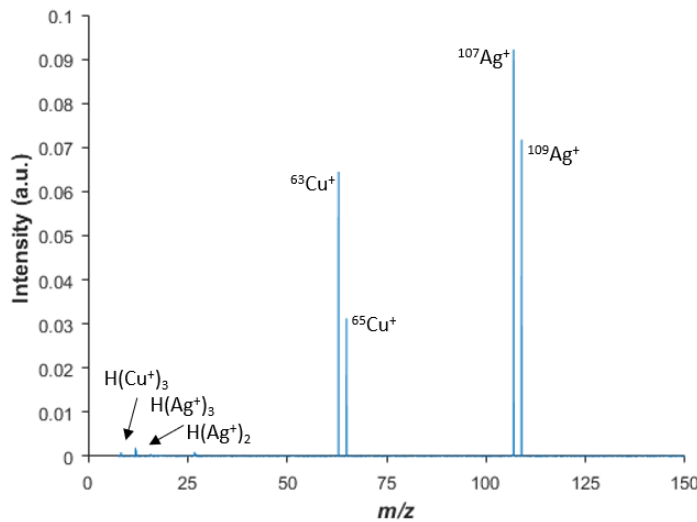
Figure 2-9 : spectre en masse issu du spectre en fréquence présenté sur la figure 2-7, issu de l'analyse d'un alliage 72% Ag/28% Cu en mode d'ions positifs grâce à l'instrument LAb-CosmOrbitrap. La calibration a été effectuée sur le pic de fréquence 666,5 kHz, attribué à la masse de 107 Ag + . Les harmoniques liées à l'ion M + d'ordre x sont notées H(M + ) x .
