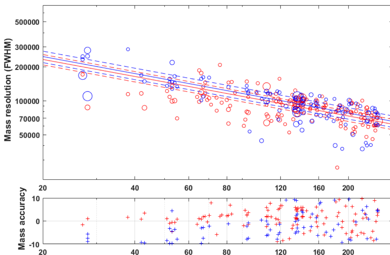
Figure 3-7 : comparaison des performances analytiques du Lab-CosmOrbitrap utilisant les deux types d'alimentation HV pour l'électrode centrale de la cellule Orbitrap. Panneau supérieur : résolution en masse (calculée à mi-hauteur de chaque pic) en fonction du rapport m/z pour les pics détectés sur les différents spectres de masse considérés. Les points en bleu sont issus d'analyses avec l'alimentation HV commerciale TF, les points en rouge d'analyses avec l'alimentation HV TRL5 du CosmOrbitrap. La taille des points est proportionnelle au SNR du pic correspondant. Les droites rouge et bleue correspondent respectivement à la loi de décroissance décrite par l'équation 3-5 pour les alimentations HV commerciale et TRL5. Il s'agit des droites moyennées de 4 spectres de masse. Les droites en pointillées rouges et bleus correspondent aux écart-types des droites de décroissance de la couleur correspondante. Panneau inférieur : écart à la masse exacte des pics détectés sur les 4 spectres de masse issu d'analyses avec l'alimentation HV commerciale TF (en bleu) et celle du CosmOrbitrap à niveau TRL5 (en rouge).
