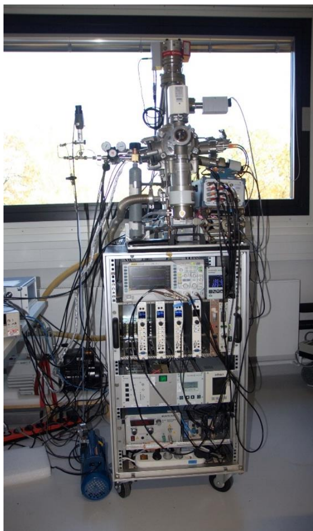
Figure 4-1 : Photographie de l'instrument EI-OLYMPIA, l'expérience OLYMPIA fonctionnelle équipée ici d'un système d'ionisation par Electron Impact (EI) et connectée à un système d'introduction de gaz. (crédit photo : B. Gaubicher ; photo prise lors d'une campagne de tests à l'IOM de Leipzig)
