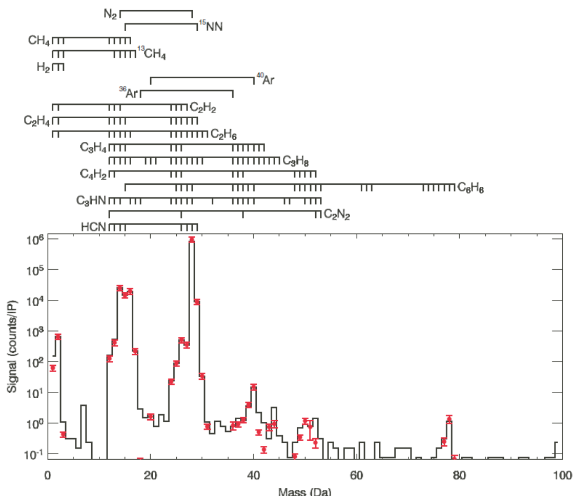
Figure 1-11 : spectre en masse moyen mesuré par l'instrument Ion Neutral Mass Spectrometer lors du premier survol de Titan par la sonde Cassini. L'altitude de la sonde était comprise entre 1174 et 1230 km. La partie supérieure de la figure montre les pics caractéristiques des différentes molécules et atomes pour cet instrument. Tiré de Waite et al. , 2005.
