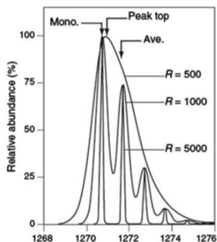
Figure 1-4 : effet de la résolution sur l'apparence d'un pic et sur l'intensité relative. Spectre en masse de C_{60}H_{86}N_{16}O_{15} à différentes résolutions en masse R (mesurées à 10 % du maximum du pic) (Mono.: pic monoisotopique, Ave.: masse moyenne), adapté de Zhang et al., 2010.
