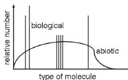
Figure 1-23 : comparaison des distributions biogéniques (biological) et non-biogéniques (abiotic) des molécules. Les processus abiotiques produisent une distribution régulière des matériaux organiques, alors que les processus biotiques sélectionnent quelques molécules spécifiques. Tirée de McKay, 2004
