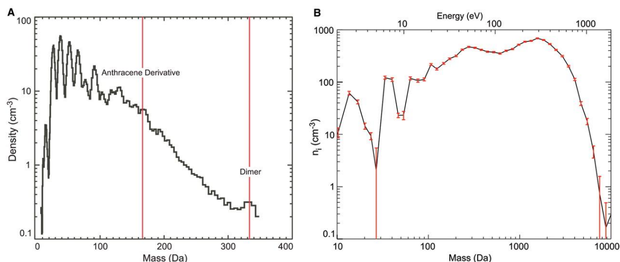
Figure 1-13 : (A) Spectre d'ions positifs de 1 à 350 daltons déduit des mesures d'énergie/charges effectuées par l'instrument IBS-CAPS pendant le 18 ème survol de Titan par la sonde Cassini, à une altitude d'environ 1000 km. La détection possible de l'anthracène et de son dimère est mise en évidence. (B) Spectre des ions négatifs de 10 à 10 000 daltons déduit des mesures d'énergie/charges effectuées par l'instrument ELS-CAPS de CAPS pendant le 18 ème survol de Titan par la sonde Cassini, à une altitude d'environ 1000 km. Tirée de Waite et al. , 2007.
