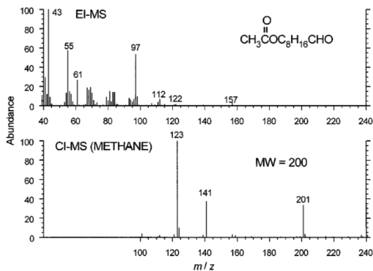
Figure 1-3 : spectres en masse du 9-acetyloxynonanal , obtenu après impact électronique (panneau supérieur, abrégé en EI-MS pour Electron Impact Mass Spectrometry) ou ionisation chimique (panneau inférieur, abrégé en CI-MS pour Chemical Ionization Mass Spectrometry), tiré de Cossé et al., 2002.
