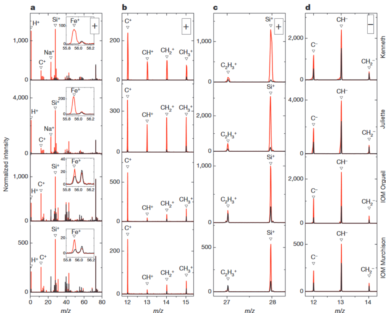
Figure A-3 : comparaison des spectres de masse cométaires (grains Kenneth et Juliette) et météoritiques (matière organique insoluble des météorites Murchison et Orgueil) acquis par temps de vol couplé à une ionisation par faisceau d'ions secondaires, en rouge, tirée de Fray et al. , 2016. Les spectres en noir correspondent au support des grains de poussières ou au substrat sur lequel les échantillons de matière organique insoluble météoritique ont été préparés. (a), spectre en ions positifs, (b) et (c), zooms de (a), (d), spectres en ions négatif.
