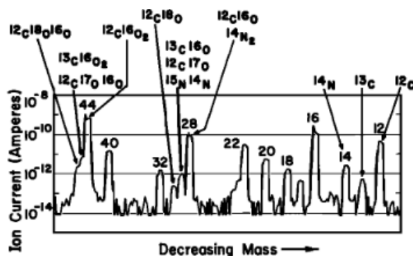
Figure A-8 : spectre de masse acquis à une altitude de 140 km lors de la descente de l'atterrisseur de la mission Viking 1, tiré de Nier et McElroy, 1977.
