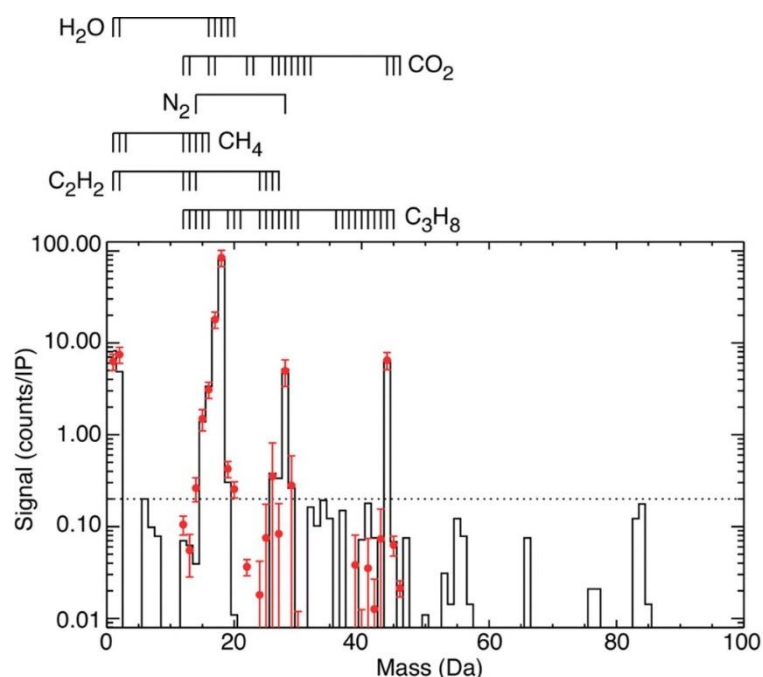
Figure 1-18 : spectre en masse moyen mesuré par l'instrument INMS lors du survol d'Encelade par la sonde Cassini. L'altitude de la sonde était inférieure à 500 km. La partie supérieure de la figure montre les pics représentatifs des différentes molécules pour cet instrument. Tiré de Waite et al. , 2006.
