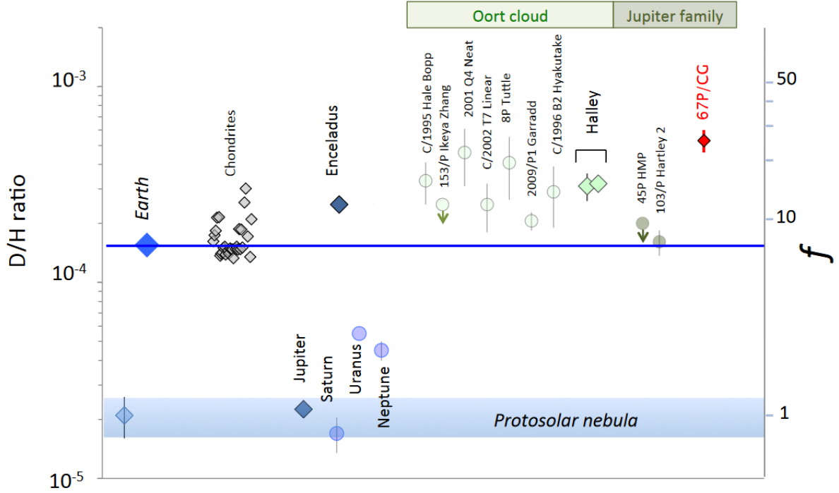
Figure A-5 : graphique représentant les rapports D/H de différents corps du Système Solaire, tiré d'Altwegg et al., 2015. Les références des valeurs issues de données de spectrométrie de masse (carrés) et de méthodes astronomiques (cercles) se trouvent dans la publication source.
