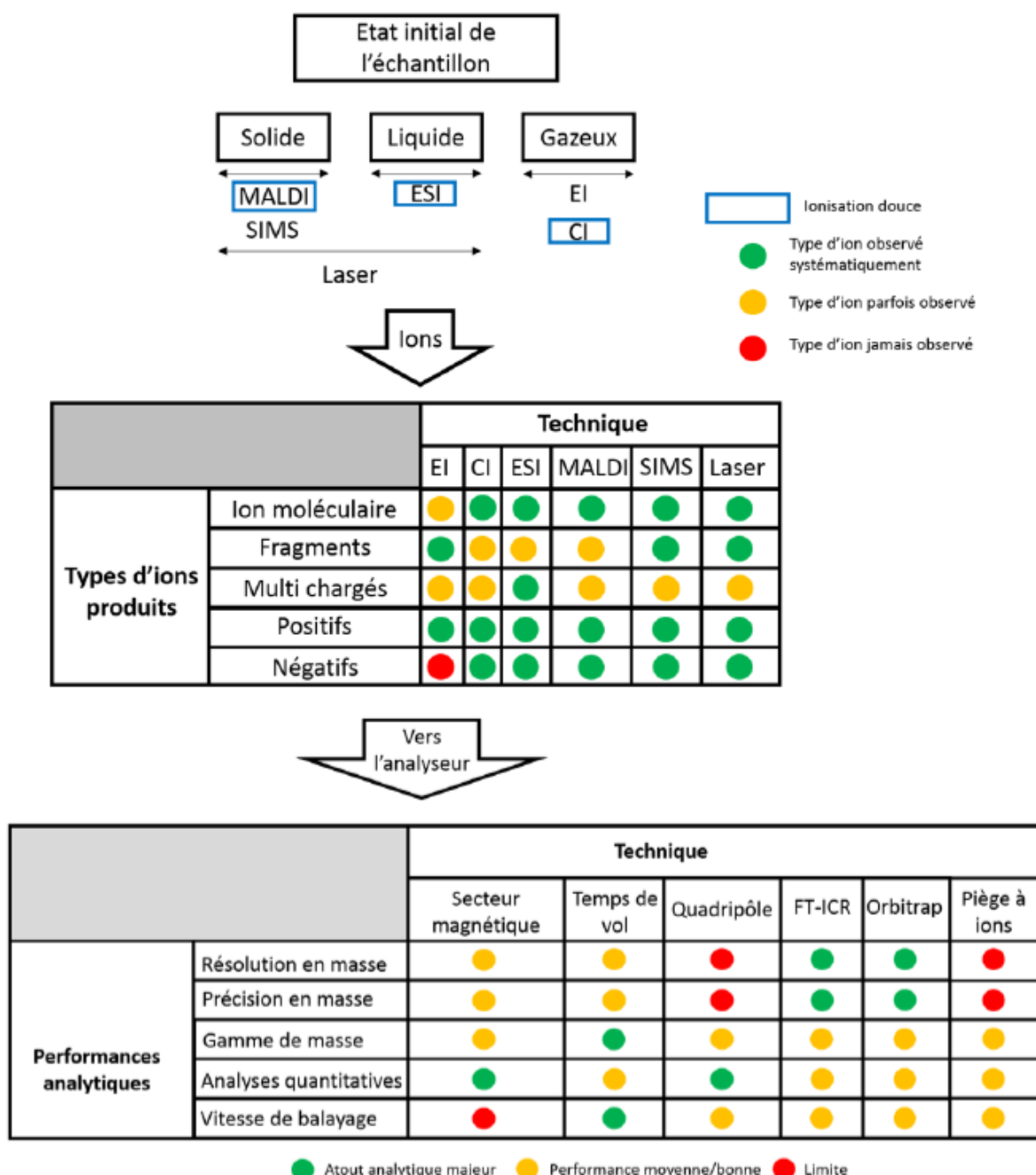
Figure 1-5 : Schéma récapitulatif des caractéristiques principales de certaines techniques d'ionisation et d'analyse en masse. Les abréviations des sources d'ions sont définies dans la section 1.2. La liste des techniques présentées est non-exhaustive. Tiré de Selliez, 2018.
