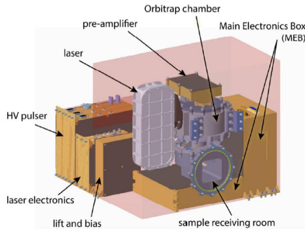
Figure 2-13 : modèle mécanique de l'instrument CORALS. Tiré de Willhite et al. , 2021.
