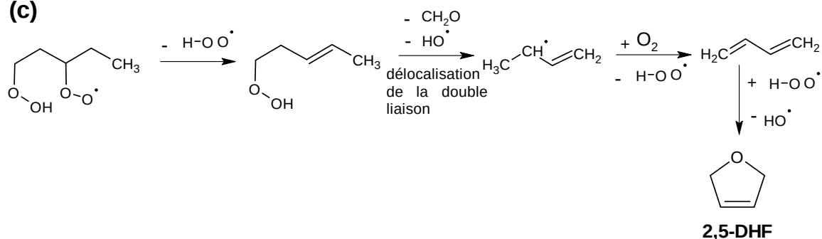
Schéma S.3. Voies réactionnelles de formation de (a) 2-butanone, (b) MVC et (c) 2,5-DHF lors de l'oxydation du n -pentane à basse température ( T = 600 K).
