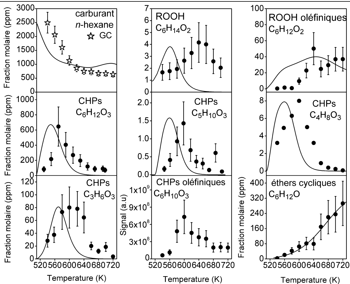
Figure V. 16. Profils d'intermédiaires d'oxydation formés lors de l'oxydation du n -hexane dans le JSR (2500 ppm, 10 atm, T = 540-720 K, \phi = 0,5 , \tau = 1.5 s). Comparaison entre les résultats expérimentaux obtenus par HRMS (symboles) et le modèle de Wang et Sarathy 1 (trait). Les données HRMS sont normalisées sur les fractions molaires des analyses GC
