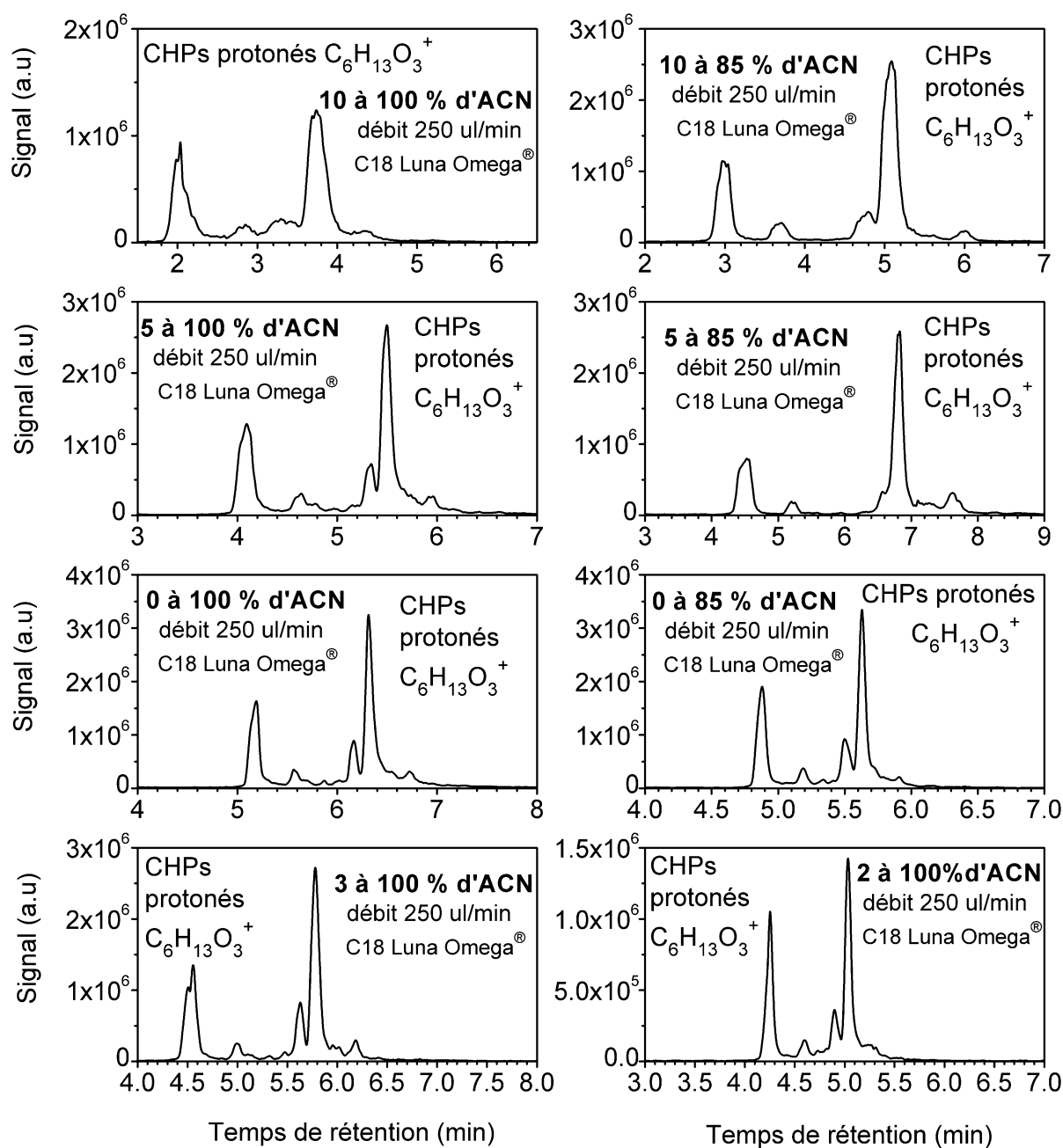
Figure S.52. Signal UHPLC/HRMS (APCI positif) d'optimisation de séparation chromatographique des CHPs. Variation de la composition de la phase mobile (ACN+H 2 O).
