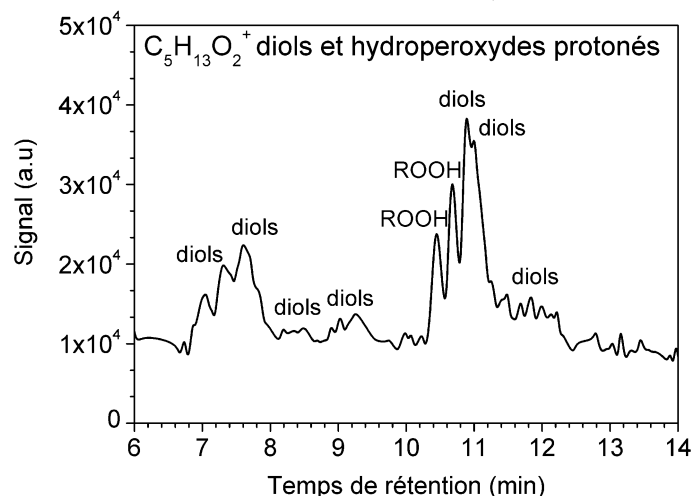
Figure V. 1. Signal UHPLC/HRMS (APCI positif) des isomères C_5H_{13}O_2^+ ( m/z 105.0906) relatifs aux diols et hydroperoxydes ( C_5H_{12}O_2 ) formés lors de l'oxydation du n -pentane dans le JSR (2500 ppm, 10 atm, T=600 K, \phi = 0,5 , \tau = 1,5 s).
