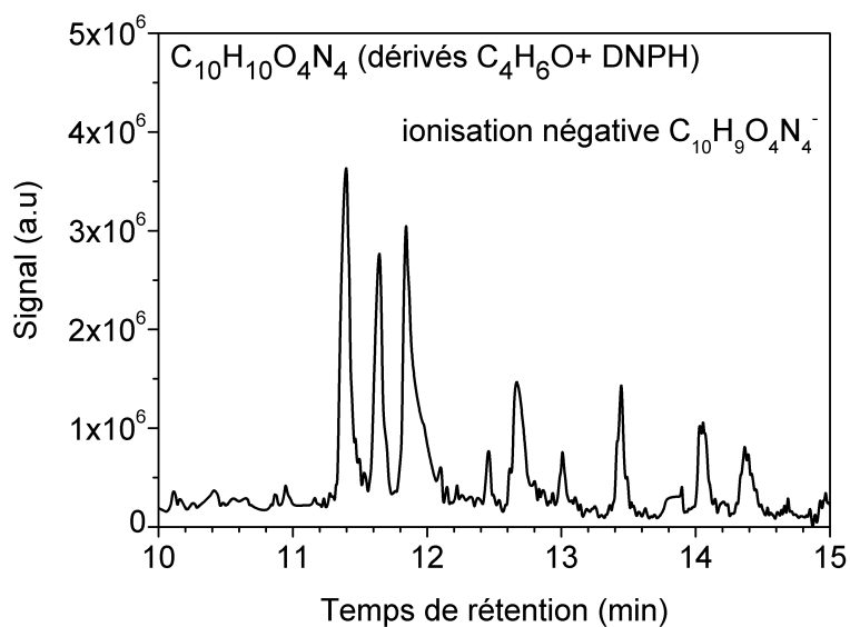
Figure S.40. Signal LC/HRMS des isomères C_{10}H_9O_4N_4^- ( m/z 249.0634) relatifs aux dérivés C_4H_6O+DNPH . Colonne C18 Luna Omega ® , phase mobile 100% H_2O (débit 100 \mu\text{l/min} ).
