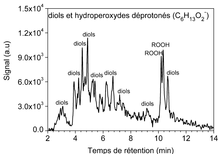
Figure V. 10. Signal UHPLC/HRMS (APCI négatif) des espèces C_6H_{13}O_2^- ( m/z 117.0923) relatives aux isomères de diols et d'hydroperoxydes ( C_6H_{14}O_2 ) formés lors de l'oxydation du n -hexane dans le JSR (2500 ppm, 10 atm, T = 600 K, \phi = 0,5 , \tau = 1,5 s).
