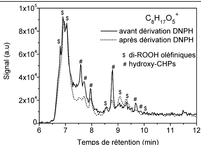
Figure IV. 10. Signal UHPLC/HRMS (APCI positif) des espèces C_8H_{17}O_5^+ ( m/z 193.1070) relatives aux isomères di-ROOH oléfiniques et hydroxy-CHPs ( C_8H_{16}O_5 ) formés lors de l'oxydation de l'éther dibutyle dans le JSR (5000 ppm, P=10 atm, T=530 K, \phi=0.5 et \tau=1 s).
