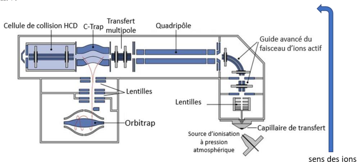
Figure II. 7. Description schématique des différents constituants du spectromètre de masse orbitrap Q-Exacte® utilisé pendant cette thèse
