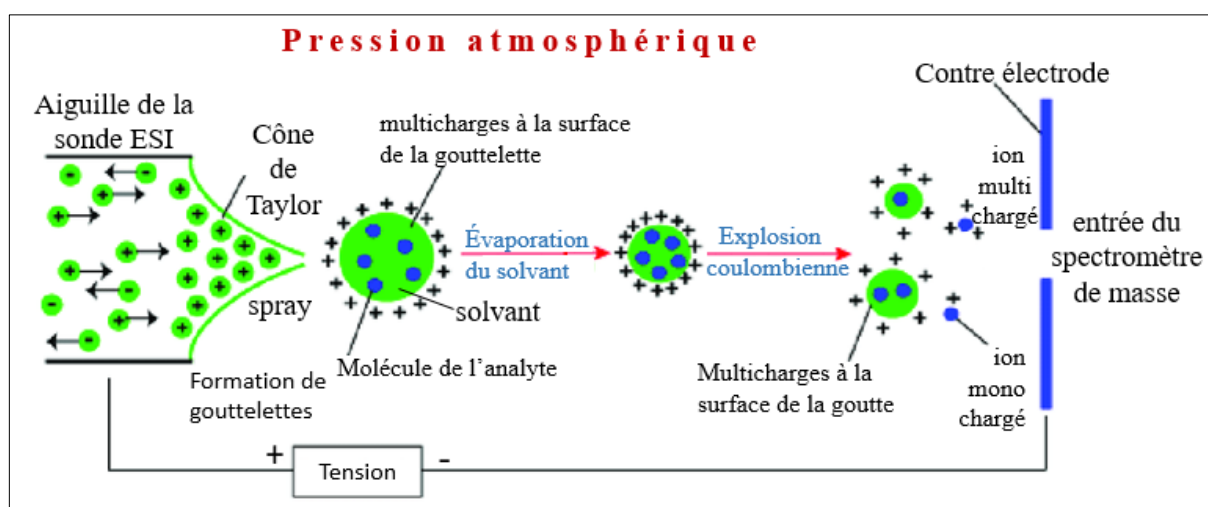
Figure S.7. Illustration descriptive de l'ionisation électrospray (ESI/HESI) : cas de l'ionisation en mode positif.
