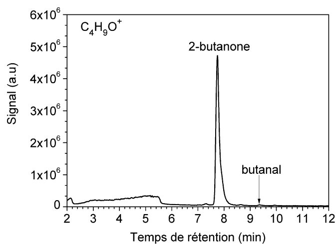
Figure S.49. Signal UHPLC/HRMS (APCI positif) des isomères C_4H_9O^+ ( m/z 73.0647) relatifs aux intermédiaires C_4H_8O formés lors de l'oxydation du n -pentane dans le JSR (2500 ppm, 10 atm, T=600 K, \phi = 0,5 , \tau = 1.5 s).
