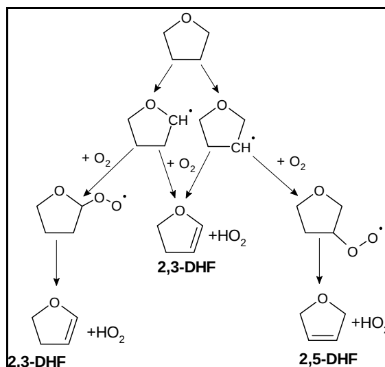
Schéma S.2. Voies de formation du 2,3-DHF et du 2,5-DHF lors de l'oxydation du THF à basse température (5000 ppm, 10 atm, T = 590\text{ K} , \phi = 0,5 , \tau = 2\text{ s} ).
