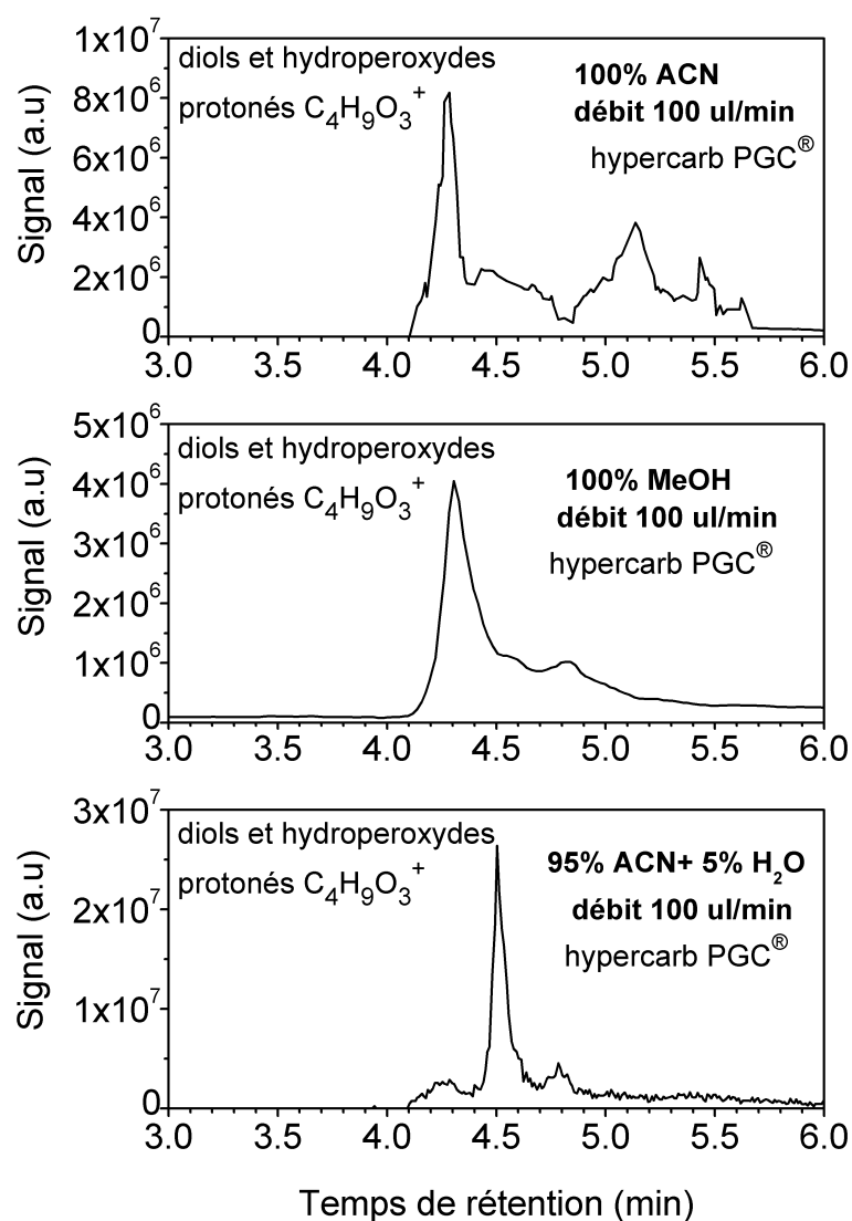
Figure S.35. Signal HPLC/HRMS des isomères C_4H_9O_3^+ ( m/z 105.0545) relatifs aux isomères diols et ROOH ( C_4H_8O_3 ) formés lors de l'oxydation du THF dans le JSR (5000 ppm, 10 atm, T=590 K, \phi = 0,5 , \tau = 2 s). Etude de l'effet de variation de la composition de la phase mobile (100% ACN, 100% MeOH et 95% ACN+5% H 2 O, débits 100 \mu l/min). Colonne chromatographique Hypercarb PGC®.
