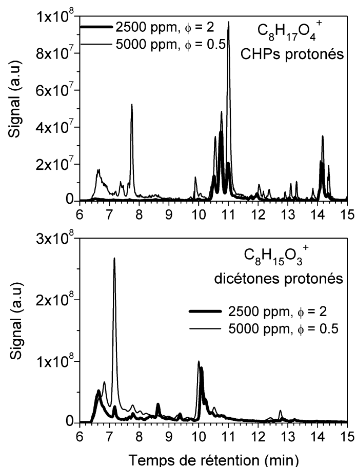
Figure S.4. Comparaison entre les intermédiaires d'oxydation (CHPs et dicétones) formés lors de l'oxydation de l'éther dibutyle dans le JSR, sous différentes conditions d'oxydation : Conditions n°1 : 5000 ppm, \phi=0.5 , \tau=1 s, P=10 atm, T=530 K et conditions n°2 : 2500 ppm, \phi=2 , \tau=1 s, P=10 atm, T=540 K. Plus d'isomères sont détecté à 5000 ppm et \phi=0.5
