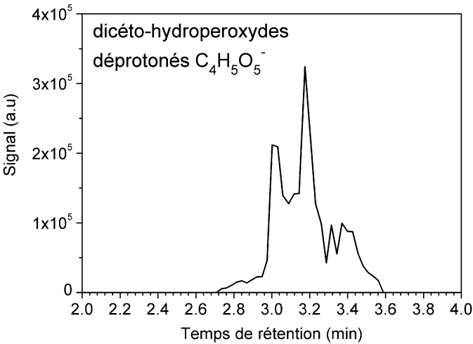
Figure IV. 3. Signal LC/HRMS (APCI négatif) des isomères C_4H_5O_5^- ( m/z 133.0142) relatifs aux dicéto-hydroperoxydes ( C_4H_6O_5 ) formés lors de l’oxydation de l’éther diéthylique dans le JSR (5000 ppm, 10 atm, T=530 K, \phi = 1 , \tau = 1 s).
