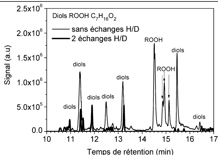
Figure V. 19. Signal UHPLC/HRMS des isomères de diols et d'hydroperoxydes ( C_7H_{16}O_2 ) formés lors de l'oxydation du n -heptane contenu dans le mélange n -heptane/iso-octane dans le JSR (2500/2500 ppm, P=10 atm, T=600 K, \phi=0.5 et \tau=1.5 s). Comparaison du signal avant C_7H_{15}O_2^- et après échanges H/D ( C_7H_{13}D_2O_2^- ).
