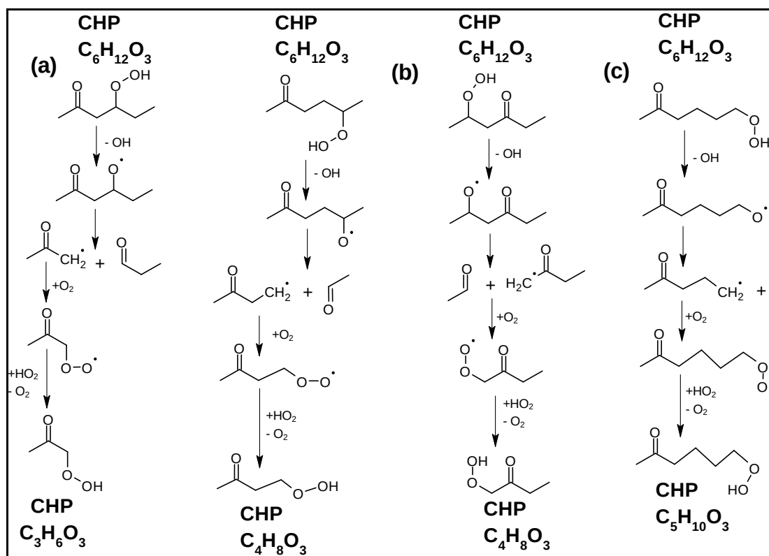
Schéma S.5. Voies réactionnelles de formation des CHPs de faibles masses (a) C_3H_6O_3 , (b) C_4H_8O_3 et (c) C_5H_{10}O_3 par décomposition des CHPs C_6H_{12}O_3 formés lors de l'oxydation du n -hexane
