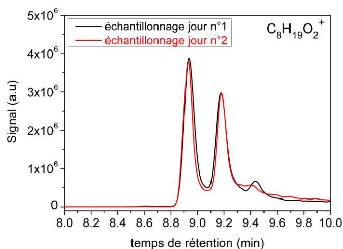
Figure II. 9. Chromatogrammes (UHPLC/HRMS APCI positif) des espèces C_8H_{19}O_2^+ ( m/z 147.1378) issus de l'oxydation de l'éther dibutylique dans le JSR (5000 ppm, P= 10 atm, T= 620 K et \phi=0.5 ). Etude de la répétabilité de la méthode d'échantillonnage en JSR (jour n°1 vs. jour n°2)
