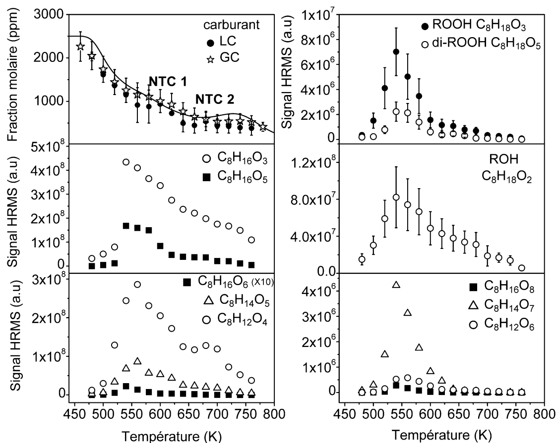
Figure IV. 26. Comparaison entre la fraction molaire (et signaux HRMS) de consommation de l'éther dibutylique obtenue par le modèle (trait) et les analyses GC et LC (symboles). Profils expérimentaux HRMS de quelques espèces poly-oxygénées formées lors de l'oxydation de l'éther dibutylique en JSR (2500 ppm, P= 10 atm, T= 460-780 K, \phi=2 et \tau=1 s). Le signal HRMS du carburant a été normalisé par rapport aux fractions molaires obtenues en GC. Les erreurs expérimentales HRMS sont estimées à 40 %.
