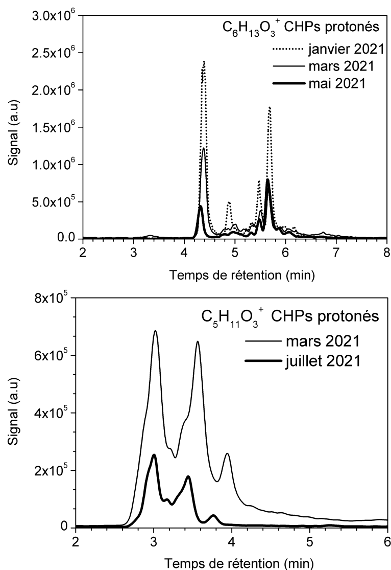
Figure S.3. Etude de la stabilité des CHPs en fonction du temps (conservation à -15\text{ }^{\circ}\text{C} ). Exemple du signal UHPLC-HRMS (APCI positif) des CHPs formés lors de l'oxydation des carburants dans le JSR : éther dibutylique ( C_8H_{17}O_4^+ , m/z 177.1121), n -heptane ( C_7H_{15}O_3^+ , m/z 147.1015), iso-octane ( C_8H_{17}O_3^+ , m/z 161.1170), n -hexane C_6H_{13}O_3^+ ( m/z 133.0856) et n -pentane ( C_5H_{11}O_3^+ , m/z 119.0702).
