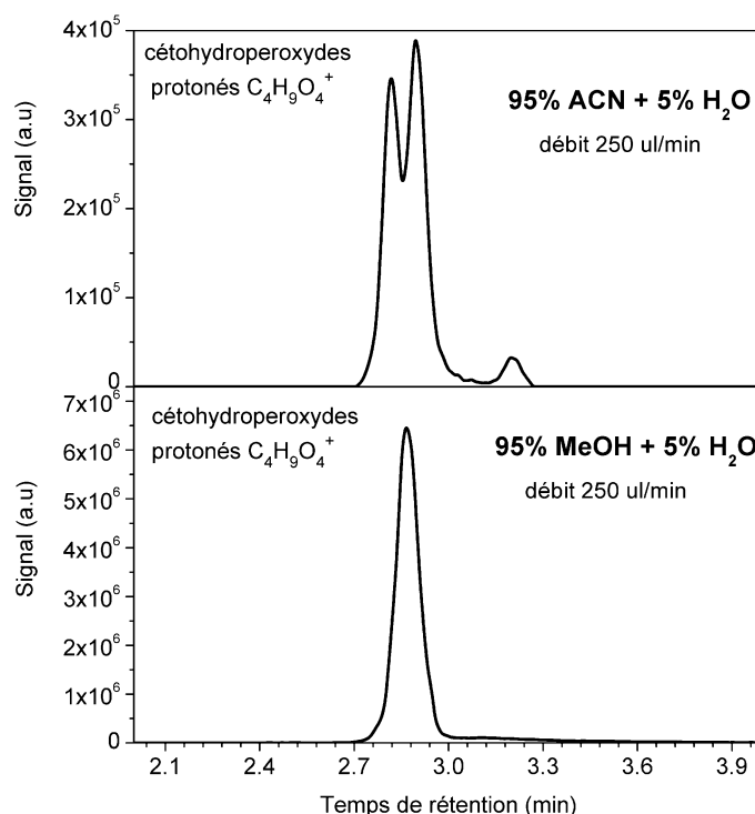
Figure S.15. Signal LC/HRMS (APCI positif) des isomères C_4H_9O_4^+ ( m/z 121.0492) relatifs aux CHPs ( C_4H_8O_4 ) formés lors de l'oxydation de l'éther diéthylique dans le JSR (5000 ppm, 10 atm, T=530 K, \phi = 1 , \tau = 1 s). Etude de la variation de la composition du solvant organique de la phase mobile : 95% d'ACN + 5% d'H 2 O vs. 95% de MeOH + 5% d'H 2 O (débit 250 \mu l/min ). Colonne chromatographique silice Ascentis®.
