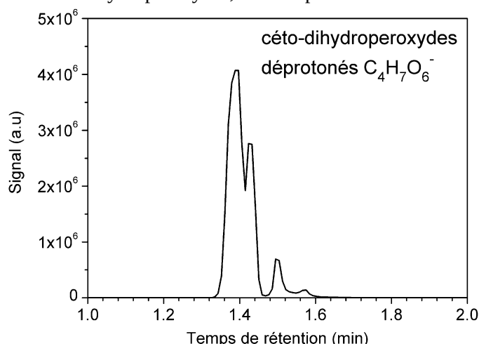
Figure IV. 2. Signal LC/HRMS (APCI négatif) des isomères C_4H_7O_6^- ( m/z 151.0247) relatifs aux céto-dihydroperoxydes ( C_4H_8O_6 ) formés lors de l'oxydation de l'éther diéthylique dans le JSR (5000 ppm, 10 atm, T=530 K, \phi = 1 , \tau = 1 s).
