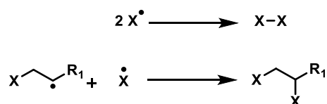
Schéma 32 Terminaison de la réaction en chaîne.
