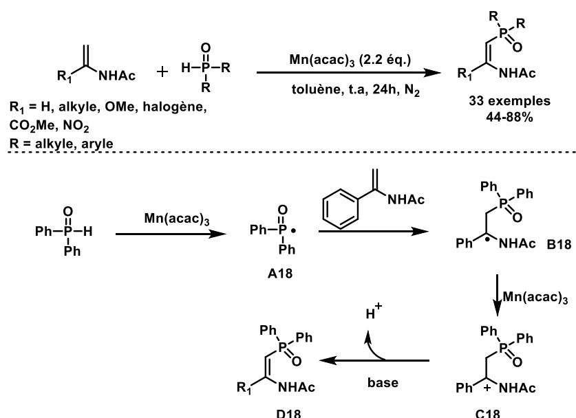
Schéma 25. Phosphorylation d'énamides secondaires médiée par \text{Mn(acac)}_3 .
