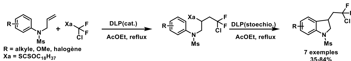
Schéma 55. Synthèse d'indolines portant une chaîne fluorée.
