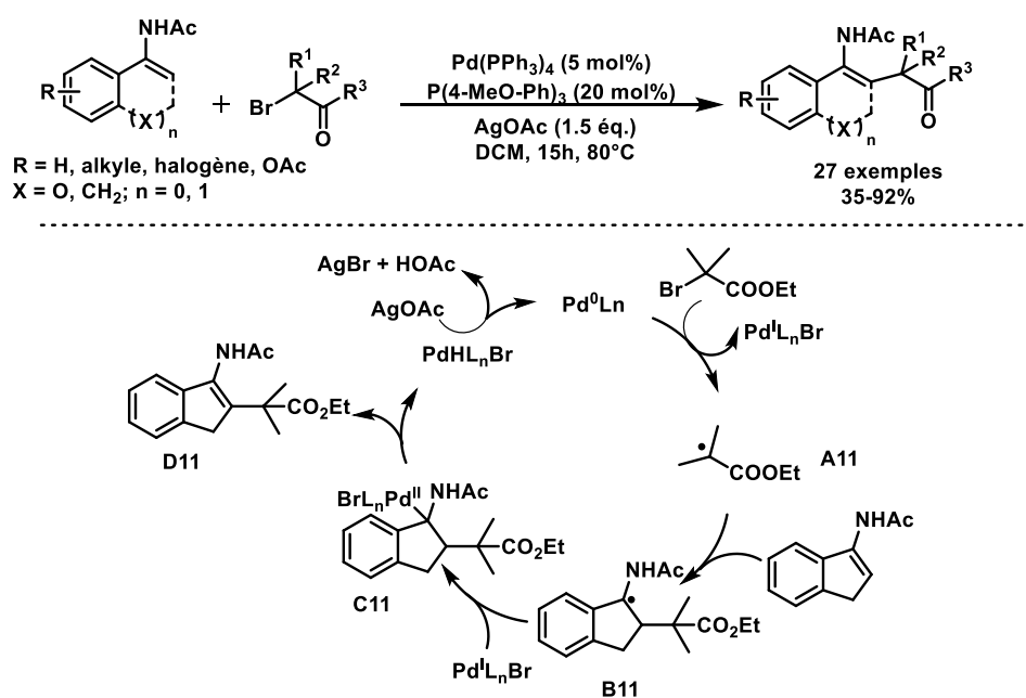
Schéma 18. Alkylation d'énammides secondaires catalysée au Pd (0).
