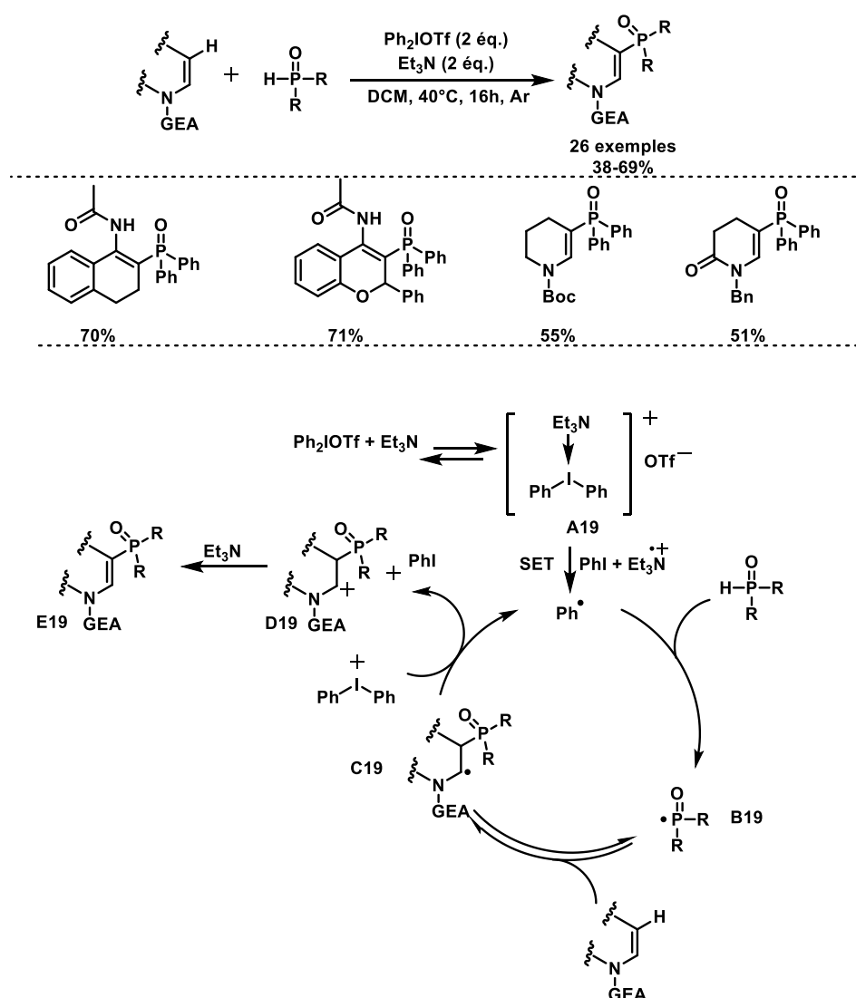
Schéma 26. Phosphorylation d'énamides tertiaires en absence de métal.
