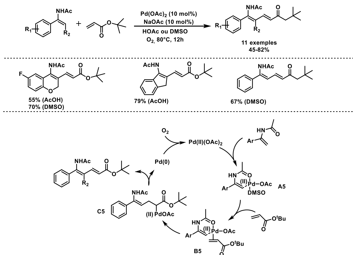
Schéma 9. Oléfination d'énamides secondaires catalysée au Pd (II).
