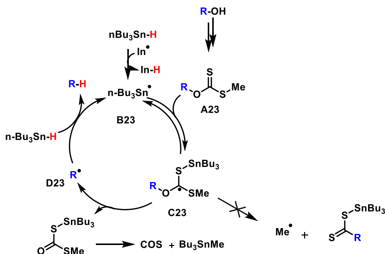
Schéma 44. Mécanisme de la réaction de Barton-McCombie.
