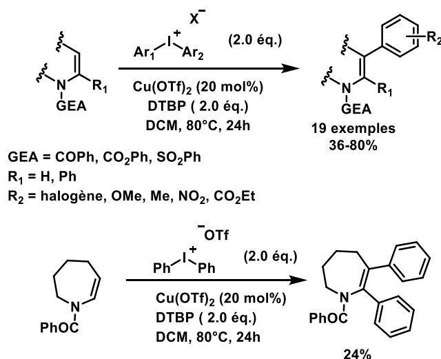
Schéma 7. Arylation d'énamides tertiaires avec des sels d'aryliodonium.
