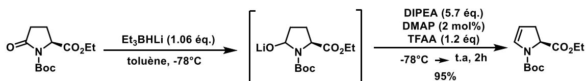
Schéma 74. Synthèse d'énamides par réduction/élimination.
