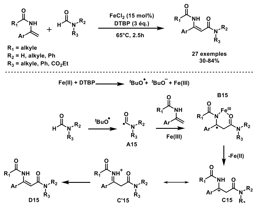
Schéma 22. Amidation d'énammides secondaires catalysée au Fe (II).
