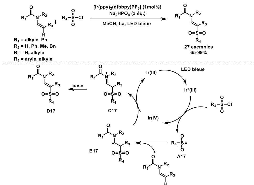
Schéma 24. Sulfonylation d'énamides tertiaires acycliques photo-induite.
