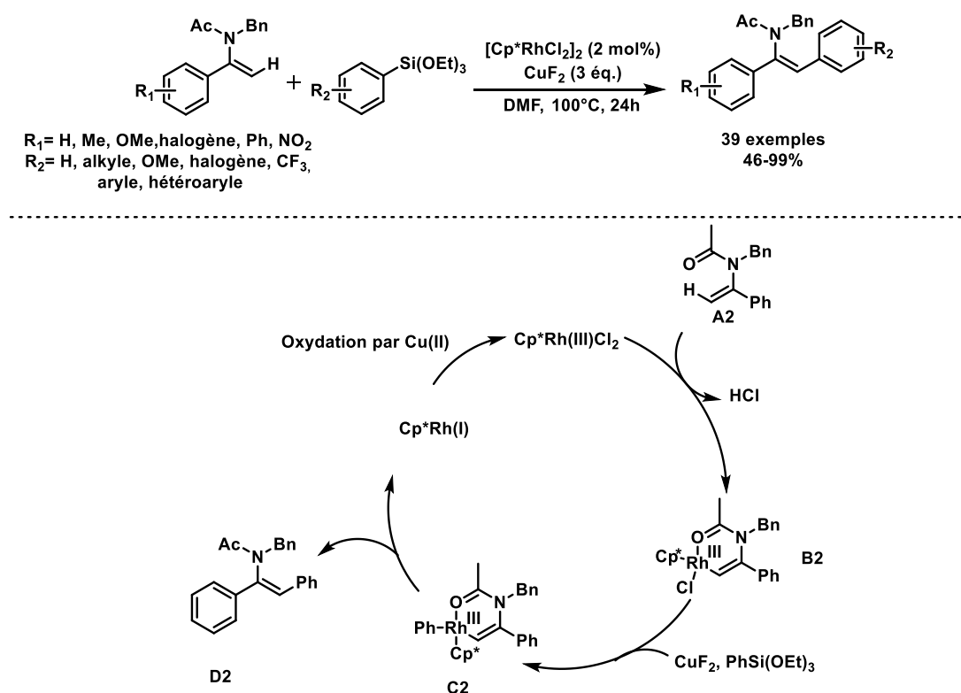
Schéma 5. Arylation d'énamides tertiaires acycliques catalysée au Rh(III) avec des arylsilanes.
