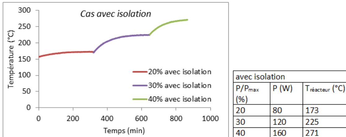
Figure B-7 Profil de T_{\text{réacteur}} en fonction du temps dans le cas avec isolation
