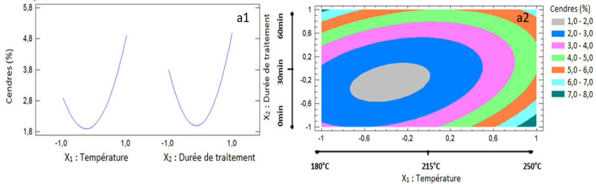
Figure III-11 Effet de la température ( X_1 ) et de la durée de traitement ( X_2 ) sur le taux de cendres (%) (a1 : GO) et les tracés de contour 2D correspondants (a2 : GO)
