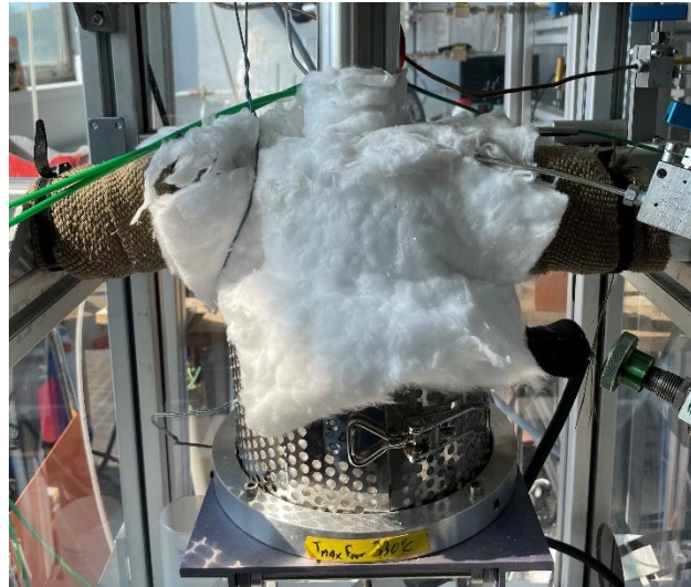
Figure III-18 Réacteur agité équipé d'isolation
