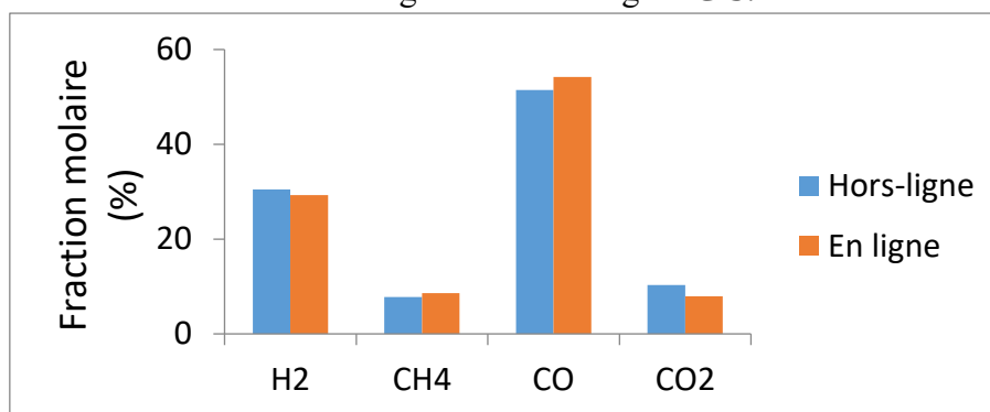
Figure C-5 Comparaison entre les deux configurations du couplage ATG-μGC (hors-ligne et en ligne)
