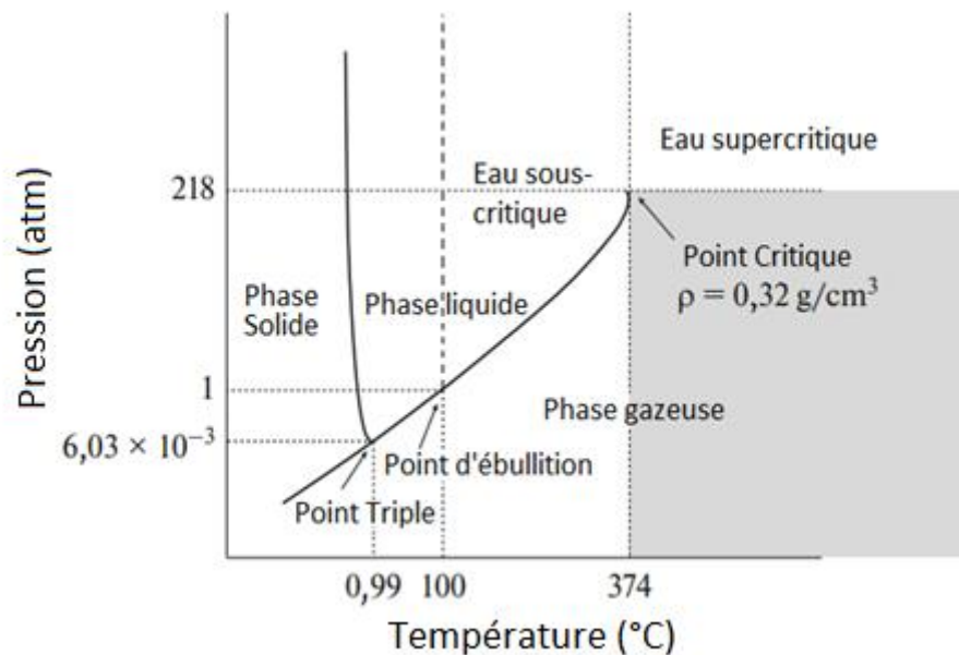
Figure I-12 Diagramme de phase de l'eau pure [64]
