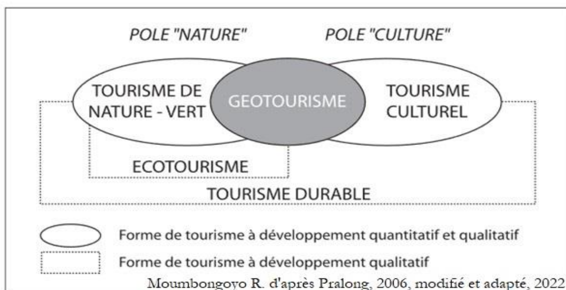
Figure 2: Le géotourisme et sa relation à d'autres formes de tourisme « nature » et « culture »
